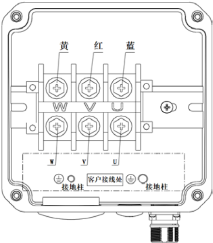
▲ U310C/U313C 接线端子示意图
