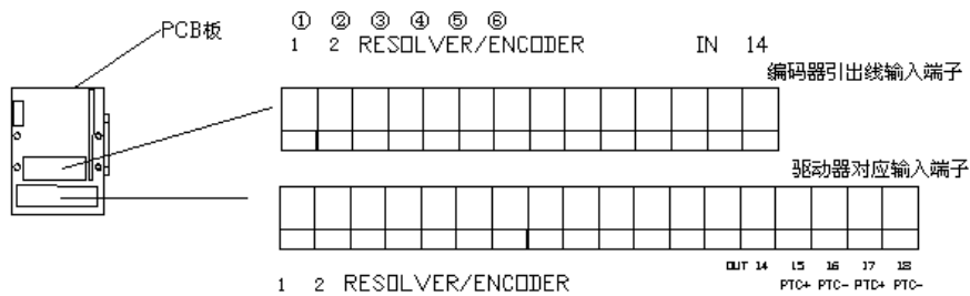
信号接线端子定义如下表（PCB 板仅适用于 U310F/U313F） (* 针对菲仕驱动器来定义，配第三方驱动器时，驱动器侧 Cos+ 与 Cos- 对调)
