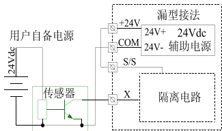
使用外部辅助电源的漏型输入接线图
