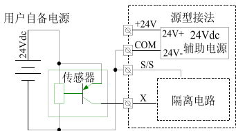
使用外部辅助电源的源型输入接线图
