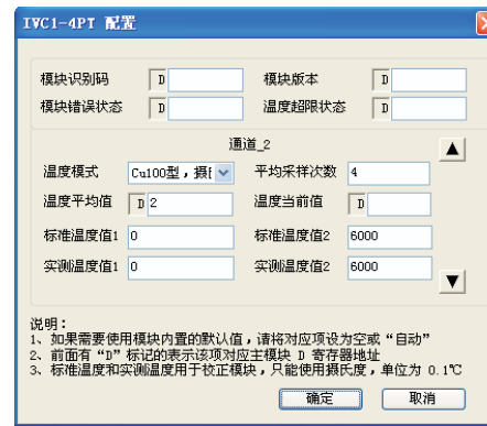
图 4-2 基本应用通道二设置
