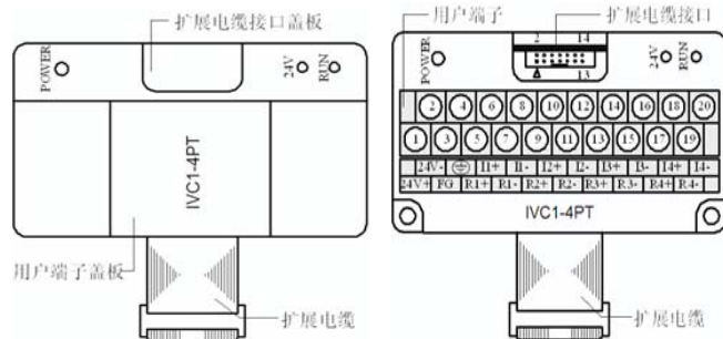
图 1-1 模块接口外观图 图 1-2 模块接口端子图
