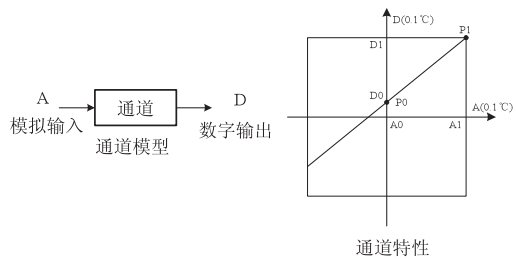
图 3-1 IVC1-4PT 通道特性示意图
