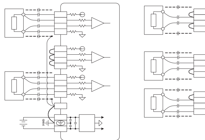
图 1-4 用户端子布线示意图
