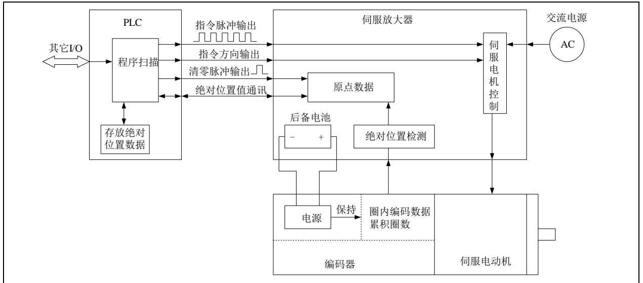
图11-1 绝对位置系统功能图
