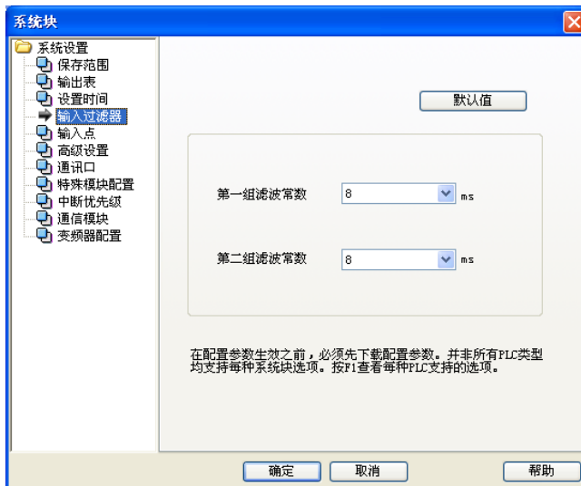
图2-6 设置输入过滤器
