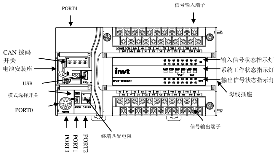
图1-2 IVC2/3/5 系列主模块的外形结构与部件布局
