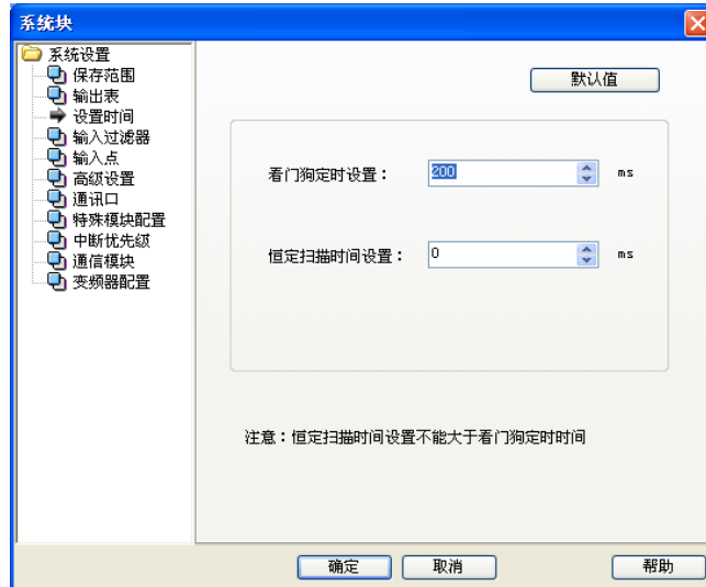
图2-5 设置时间
