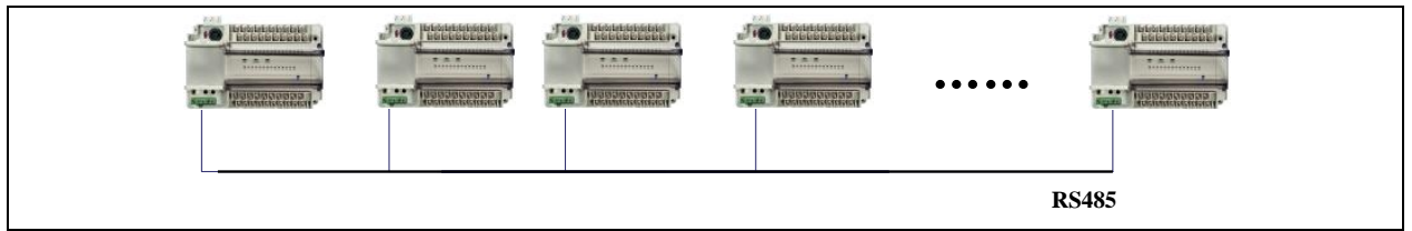
图10-7 N:N 单层网络
