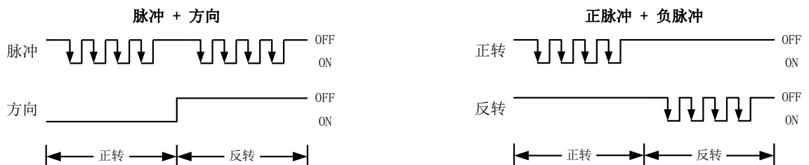
图11-7 脉冲输出形式的定义
