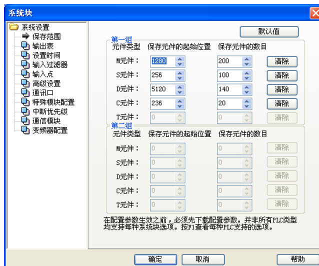
图2-3 配置保存元件地址范围
