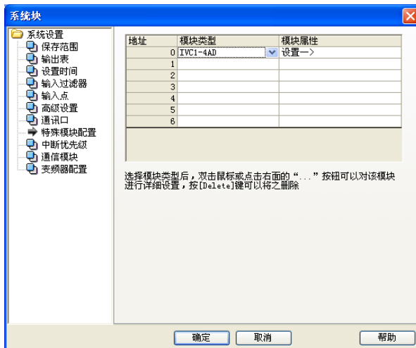
图2-10 配置特殊模块
