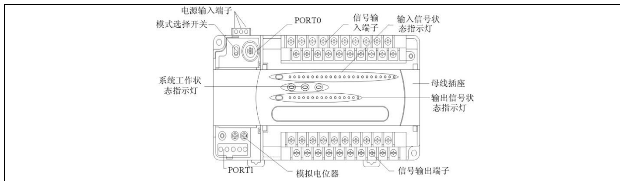
图1-1 IVC1L/1S 系列主模块外形结构
