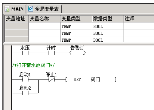
图4-9 采用了符号编址的状态
