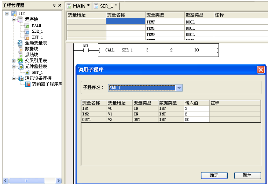
图4-12 调用子程序
