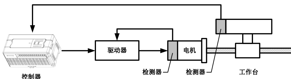
图11-4 闭环控制系统简图
