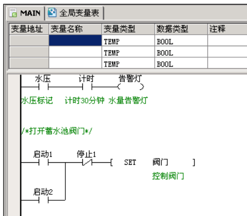
图4-10 显示元件注释时的梯形图程序
