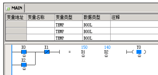
图2-23 被强制软元件的锁标记
