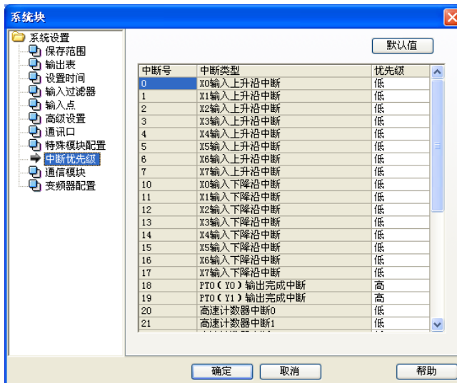
图2-12 设置中断优先级
