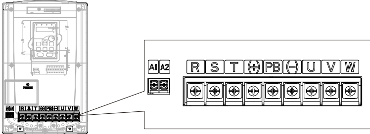
图 4.13 380V 22~30kW 主回路端子示意图
