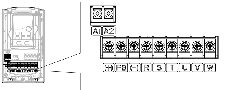
图 4.10 380V 4~5.5 kW 主回路端子示意图
