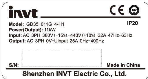
图 3.4 产品铭牌
