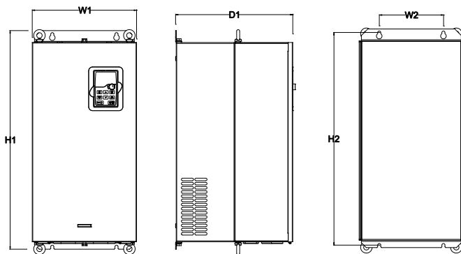
图 C.4 380V 37-110kW 壁挂安装示意图
