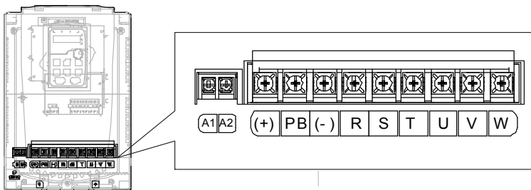
图 4.12 380V 15~18kW 主回路端子示意图
