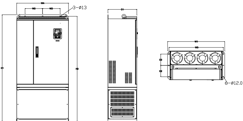
图 C.16 660V 250-350kW 落地安装示意图
