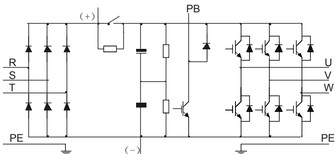
图 3.1 380V（小于 30kW（含））主回路简图
