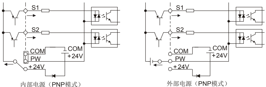
图 4.23 PNP 模式示意图
