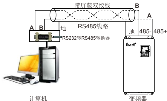
图 11.1 RS485 单机应用时的物理接线图
