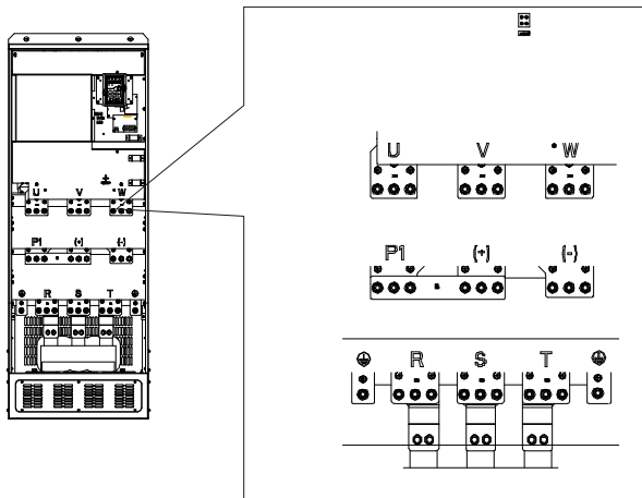
图 4.18 660V 400~630kW 主回路端子示意图
