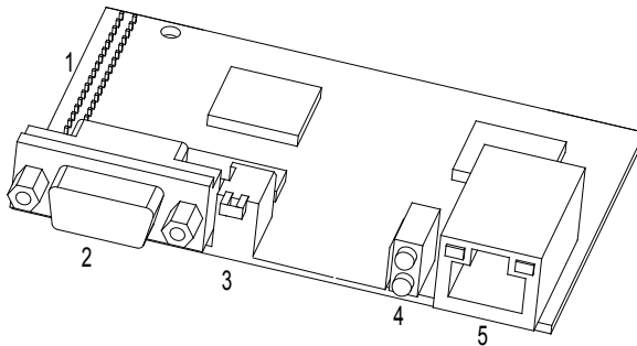
图 A.1 EC-TX-103 通讯卡外形图
