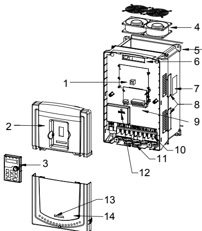
图 3.6 产品结构示意图
