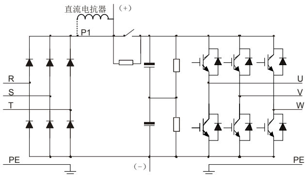
图 3.2 380V（大于 37kW（含））主回路简图
