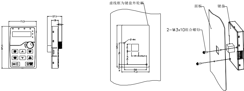
键盘无支架安装开孔尺寸及示意图
