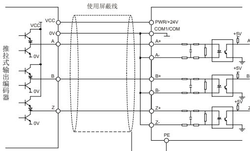
推拉式输出方式接线图 2
