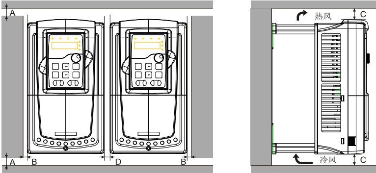
图 4.4 并行安装
