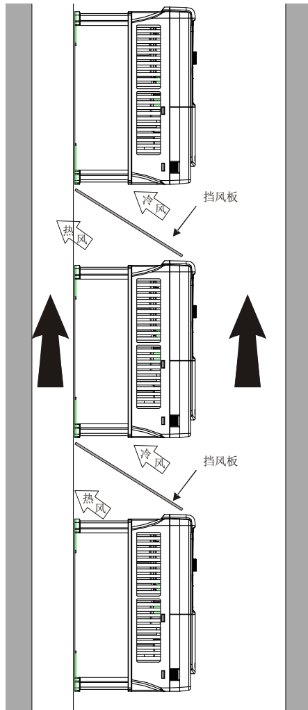
图 4.5 垂直安装
