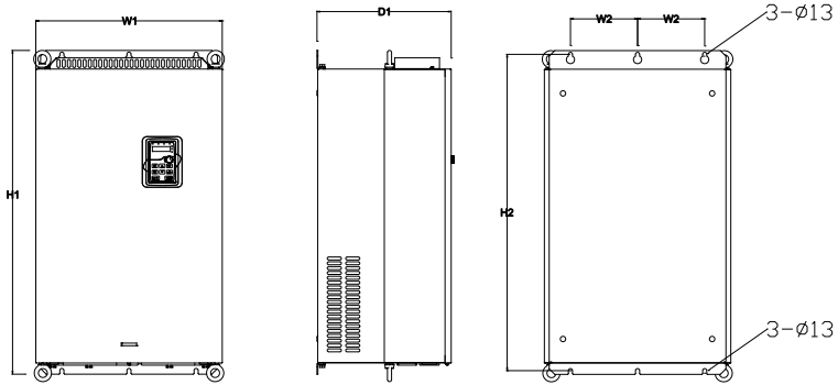
图 C.5 380V 132-200kW 壁挂安装示意图
