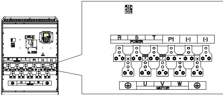
图 4.17 380V 220~315kW、660V 250~350kW 主回路端子示意图
