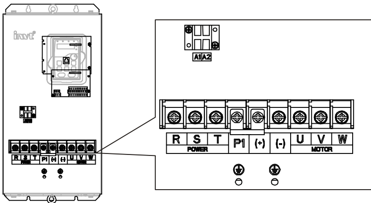
图 4.14 380V 37~55kW、660V 22~45kW 主回路端子示意图
