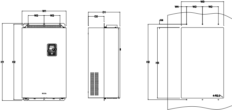
图 C.9 380V 132-200kW 法兰安装示意图
