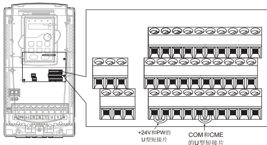
图 4.21 U 型短接位置示意图
