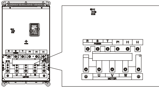
图 4.16 380V 132~200kW、660V 160~220kW 主回路端子示意图
