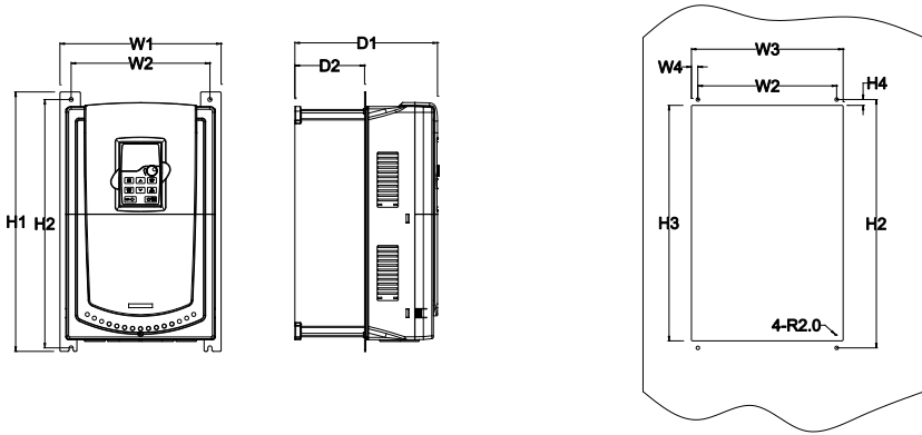
图 C.7 380V 1.5-30kW 法兰安装示意图
