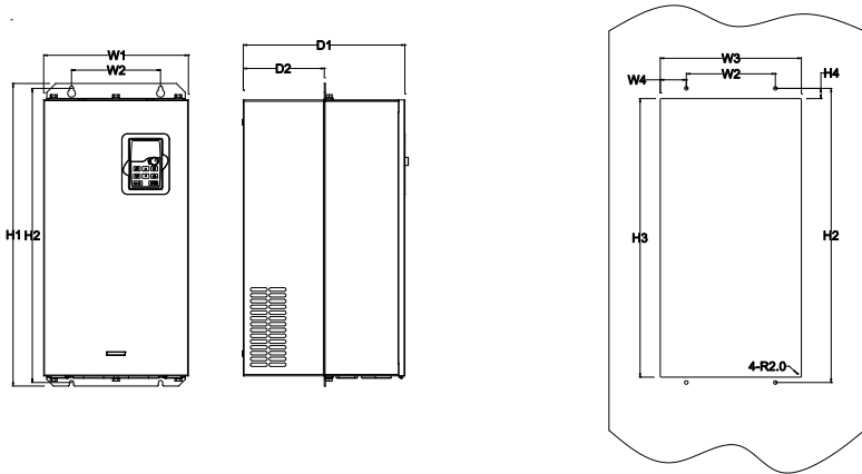
图 C.8 380V 37-110kW 法兰安装示意图
