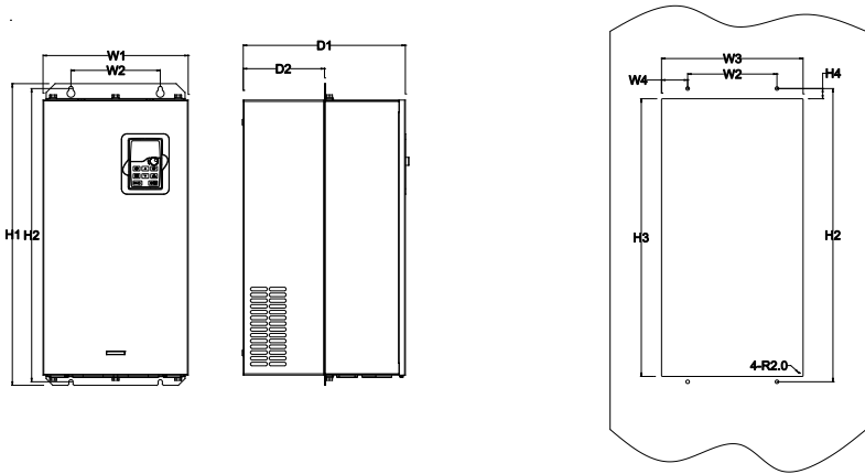
图 C.14 660V 22-132kW 法兰安装示意图
