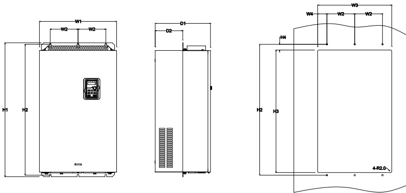
图 C.15 660V 160-220kW 法兰安装示意图
