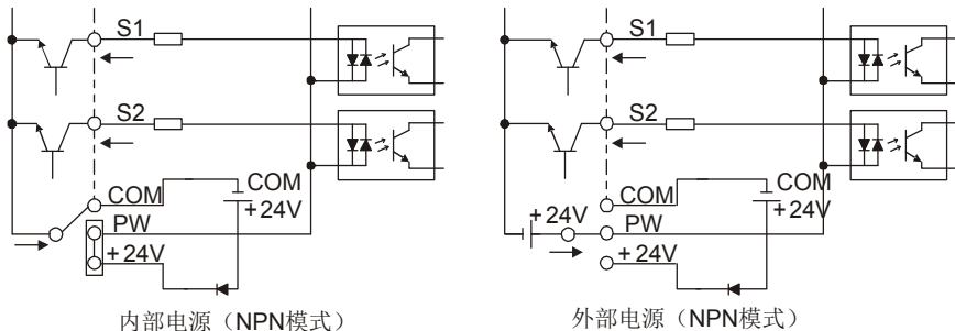
图 4.22 NPN 模式示意图
