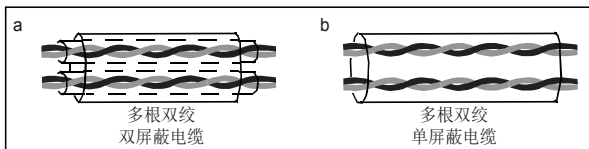
图 D.2 动力电缆布线
