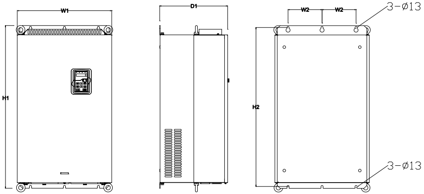
图 C.12 660V 160-220kW 壁挂安装示意图
