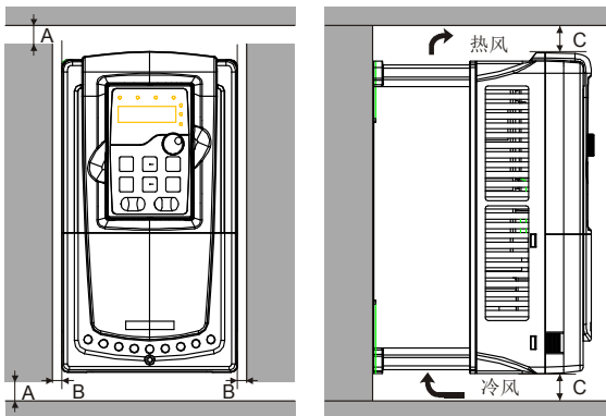
图 4.3 单台安装
