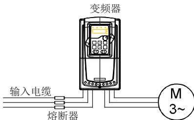
图 4.24 熔断器配置图
