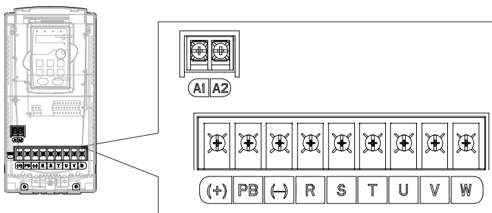
图 4.11 380V 7.5~11kW 主回路端子示意图
