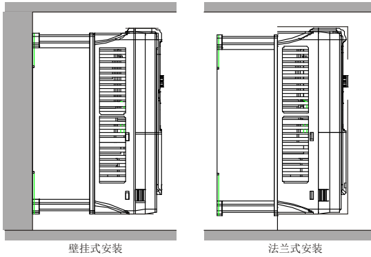
图 4.2 安装方式
