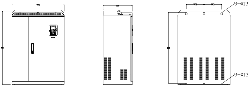
图 C.6 380V 220-315kW 壁挂安装示意图
