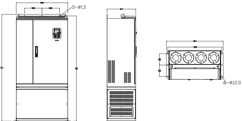
图 C.10 380V 220-315kW 落地安装示意图
