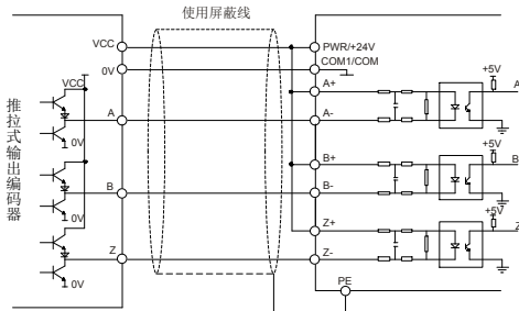
推拉式输出方式接线图 1
