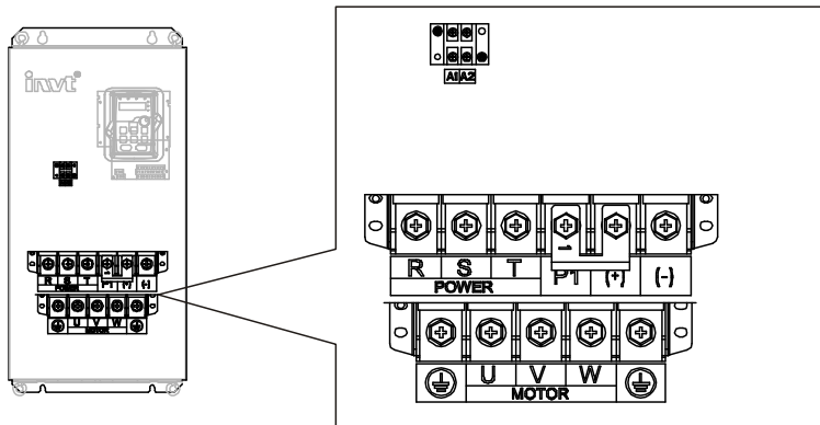
图 4.15 380V 75~110kW、660V 55~132kW 主回路端子示意图
