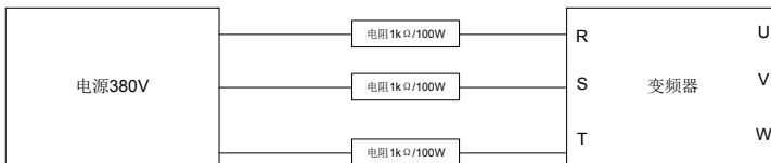
图 10.1 380V 驱动装置充电电路示例
