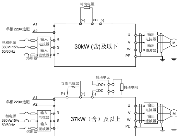
图 4.7 380V 主回路接线图
