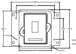
键盘转接支架
