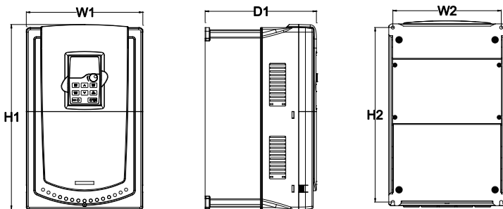
图 C.3 380V 1.5-30kW 壁挂安装示意图
