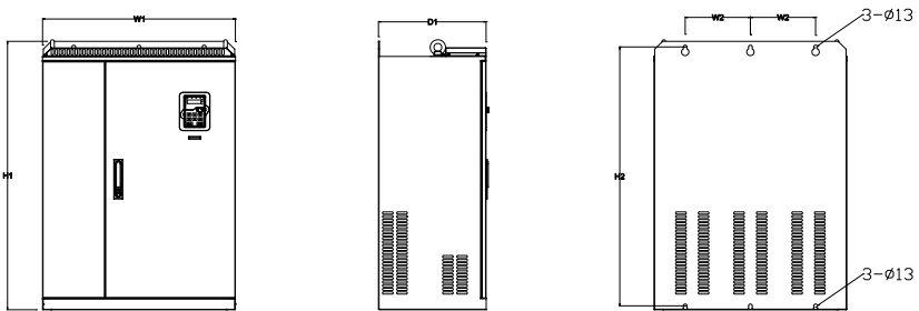
图 C.13 660V 250-350kW 壁挂安装示意图
