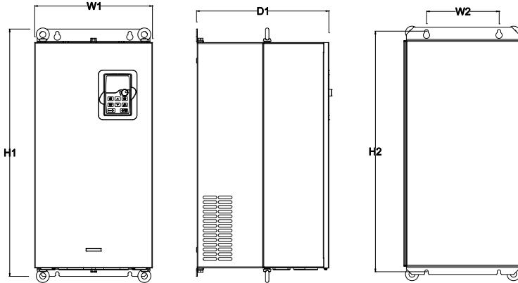
图 C.11 660V 22-132kW 壁挂安装示意图
