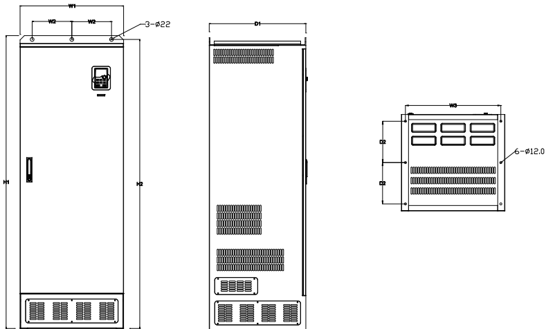
图 C.17 660V 400-630kW 落地安装示意图
