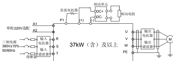
图 4.8 660V 主回路接线图
