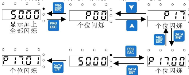
图 5-4 查看参数示意图
