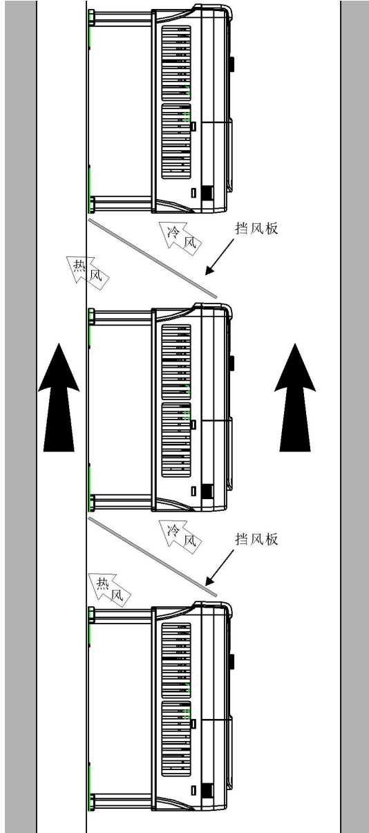
图 4-5 垂直安装
