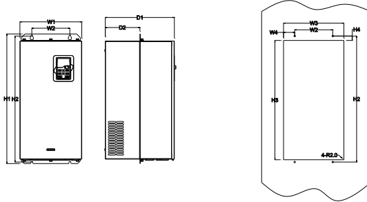
380V 37-110kW 法兰安装示意图
