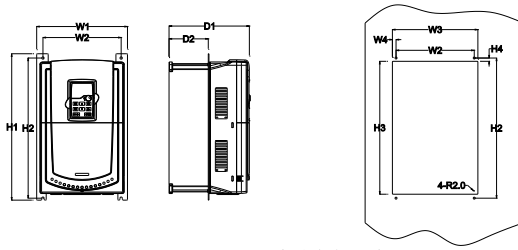
380V 1.5-30kW 法兰安装示意图
