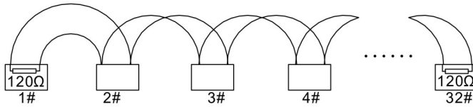
图 2 菊花接法现场接线图
