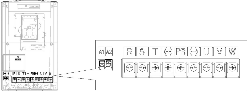
图 4-13 380V 22~30kW 主回路端示意图
