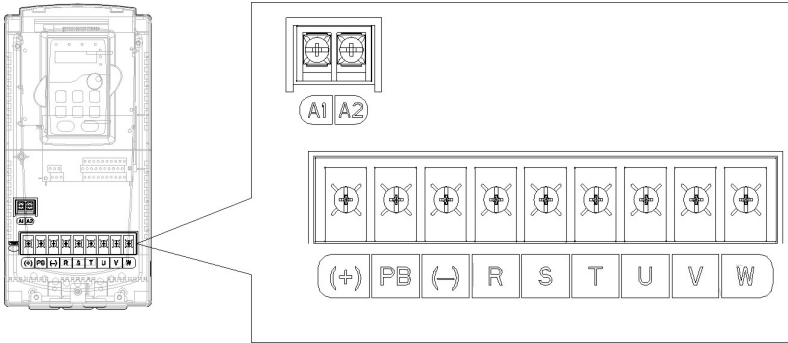
图 4-11 380V 7.5~11kW 主回路端示意图
