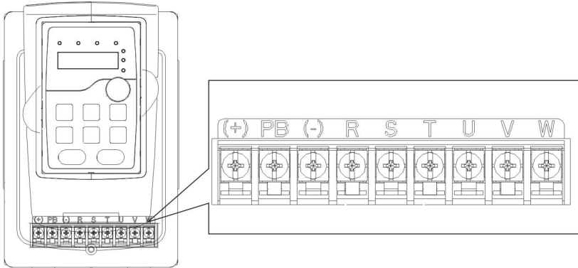
图 4-9 380V 1.5~2.2kW 主回路端子示意图
