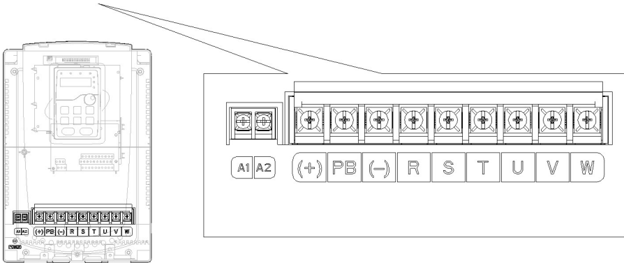
图 4-12 380V 15~18kW 主回路端示意图
