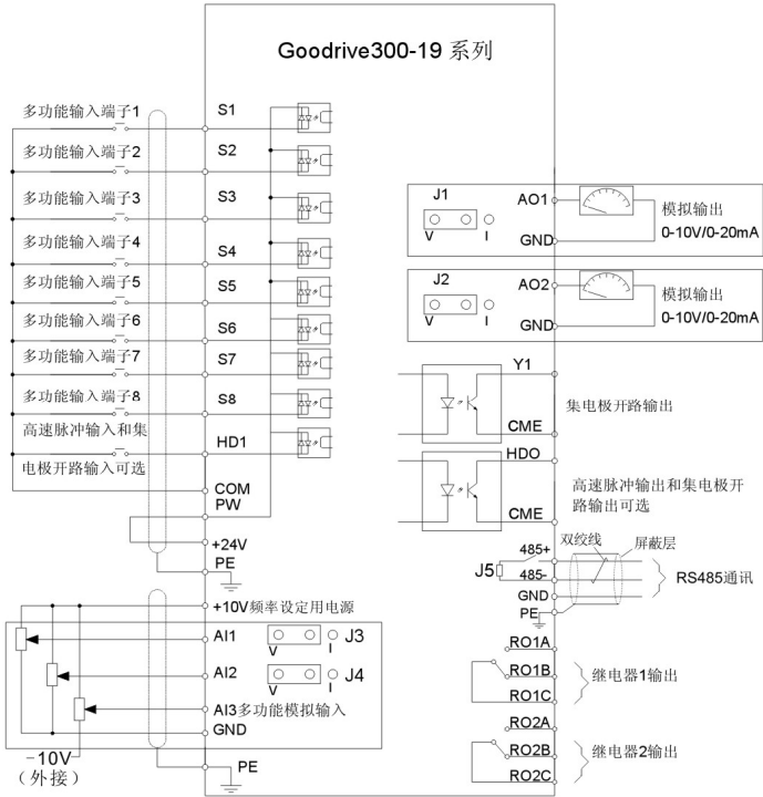
图 4-20 控制回路接线图
