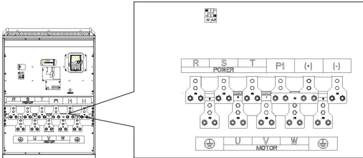
图 4-17 380V 220~315kW 主回路端子示意图
