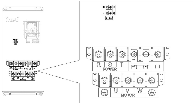
图 4-15 380V 75~110kW 主回路端示意图
