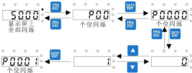
图 5-2 修改参数示意图
