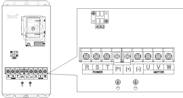
图 4-14 380V 37~55kW 主回路端示意图
