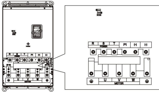
图 4-16 380V 132~200kW 主回路端子示意图
