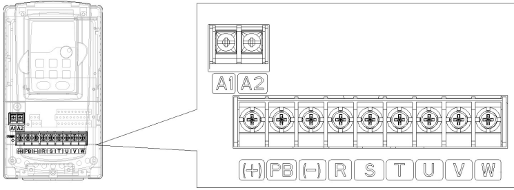
图 4-10 380V 4~5.5 kW 主回路端示意图
