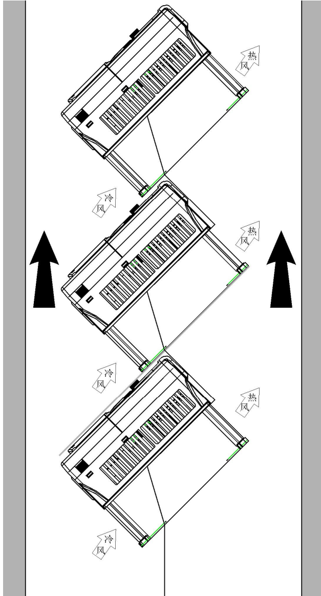
图 4-6 倾斜安装
