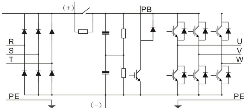
图 3-2 380V（小于 30kW（含））主回路简图
