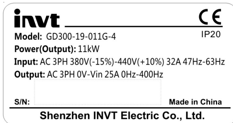
图 3-3 产品铭牌
