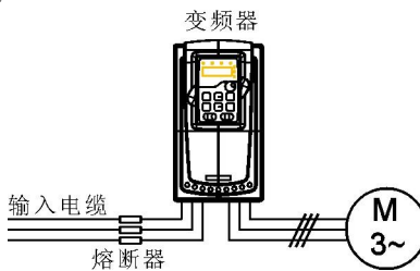
图 4-25 熔断器配置图
