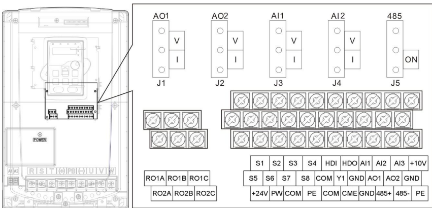
图 4-21 控制端子示意图
