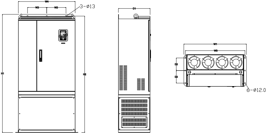
380V 220-315kW 落地安装示意图
