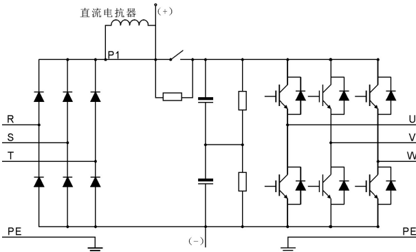
图 3-1 380V（大于 37kW（含））主回路简图
