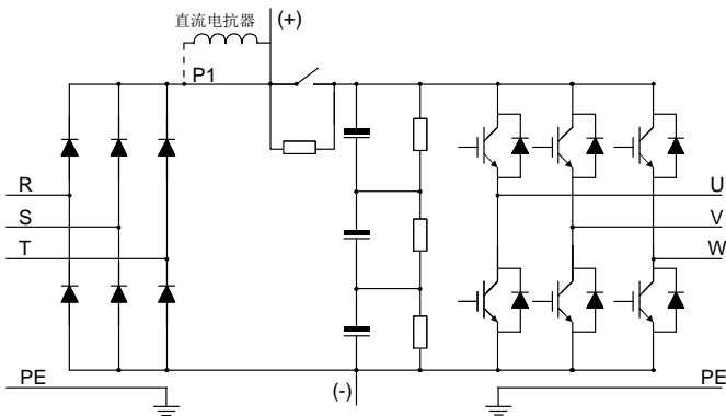
图 3-4 500V (≥22kW) 主回路简图
