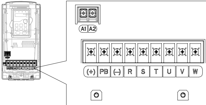
图 4-12 380V 7.5~11kW 和 500V 4~18.5kW 主回路端子示意图
