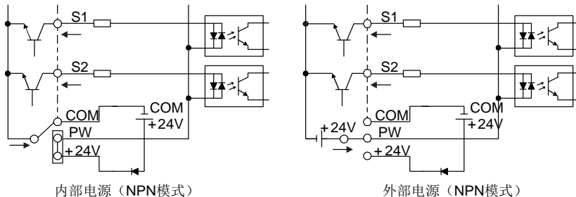
图 4-24 NPN 模式示意图
