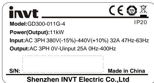
图 3-6 产品铭牌
