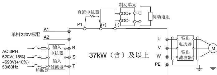
图 4-9 660V 主回路接线图
