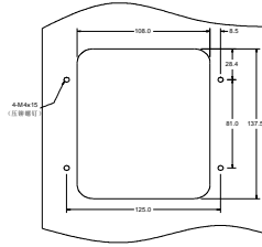
客户安装尺寸
