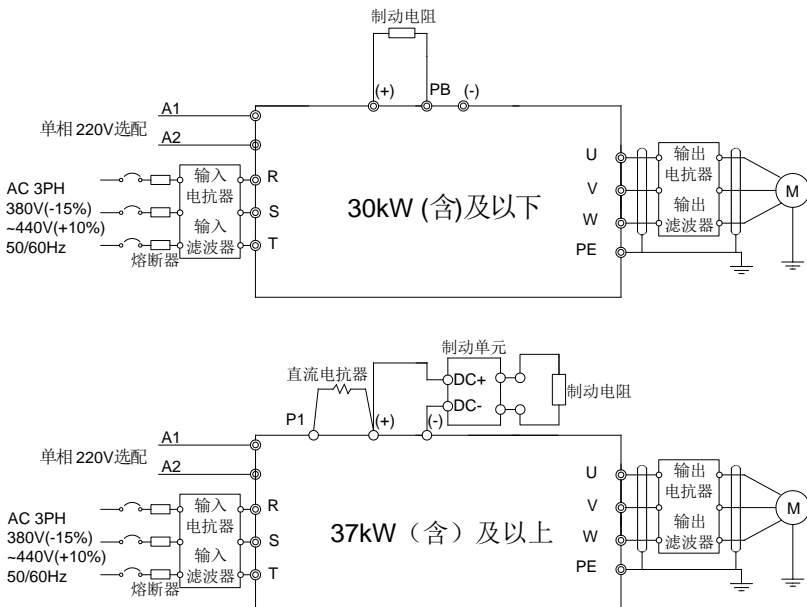
图 4-7 380V 主回路接线图
