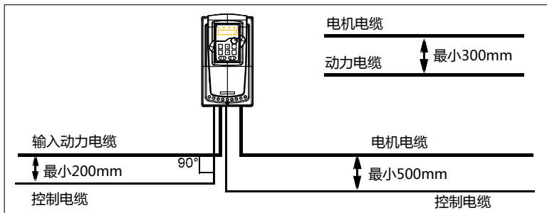
布线距离
