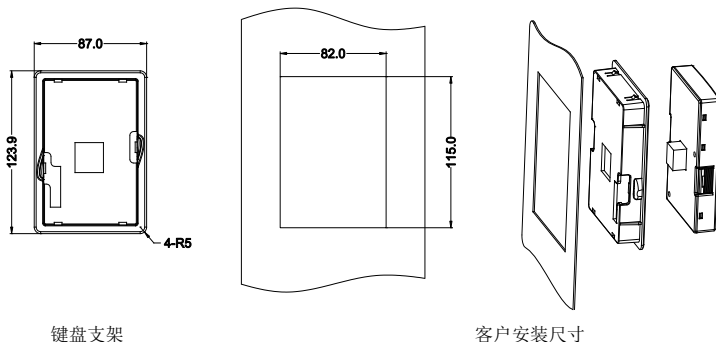
键盘支架
