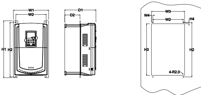
380V 1.5~30kW 法兰安装示意图
