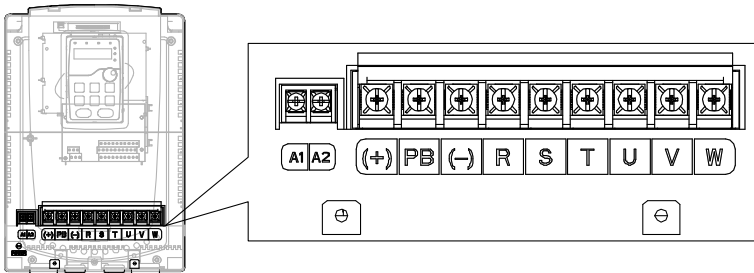
图 4-13 380V 15~18kW 主回路端子示意图
