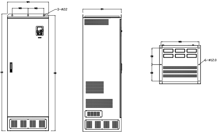
380V 350~500kW 落地安装示意图
