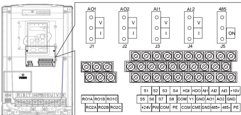
图 4-22 控制端子示意图
