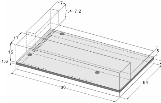
EC-TX-103 通讯卡外形尺寸图（单位：mm）
