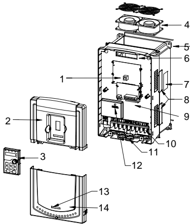
图 3-8 产品结构示意图
