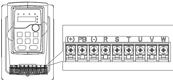
图 4-10 380V 1.5~2.2kW 主回路端子示意图
