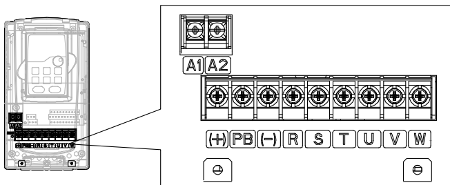
图 4-11 380V 4~5.5 kW 主回路端子示意图
