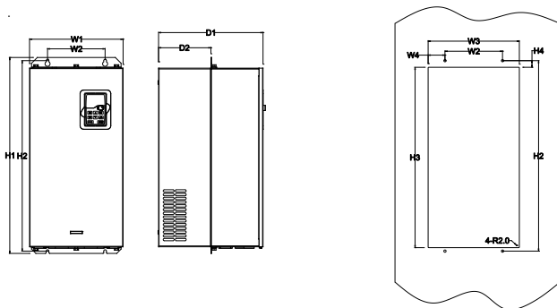
380V 37~110kW 法兰安装示意图
