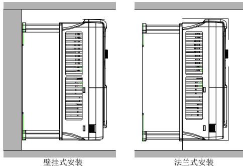
图 4-2 安装方式
