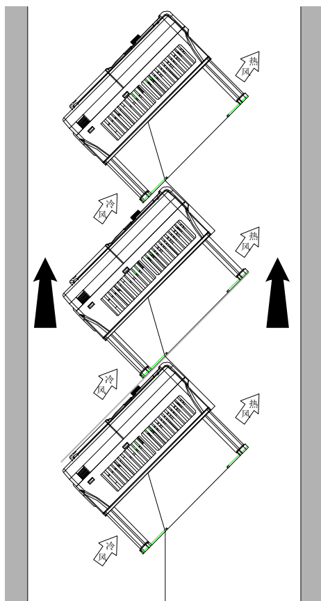
图 4-6 倾斜安装
