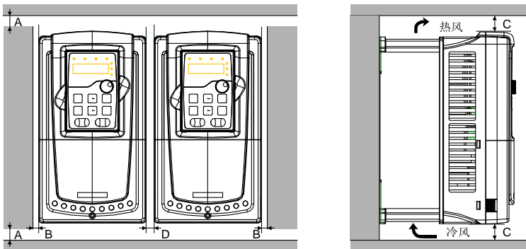
图 4-4 并行安装
