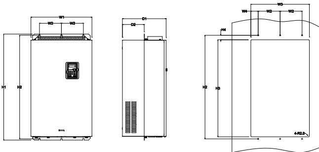
380V 132~200kW 法兰安装示意图
