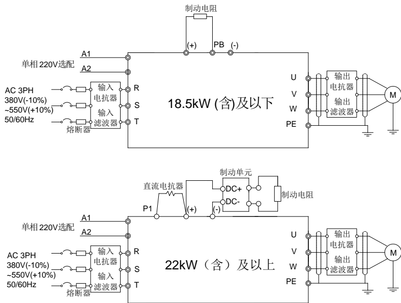
图 4-8 500V 主回路接线图
