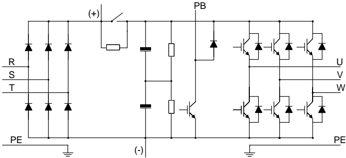
图 3-3 500V (≤18.5kW) 主回路简图
