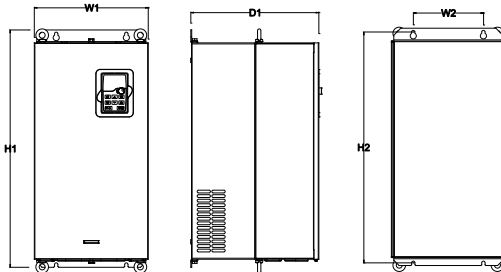
500V 22~75kW 壁挂安装示意图
