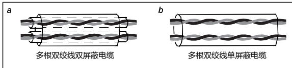
动力电缆布线
