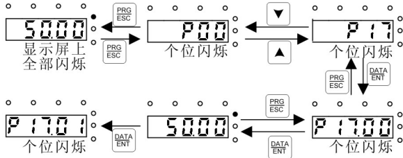
注意：在设定数值时,利用 能快速移位,或者通过 + 来调整。 图 5-5 查看参数示意图
