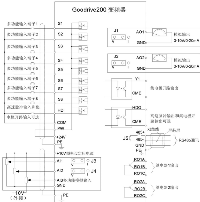
图 4-20 控制回路接线图
