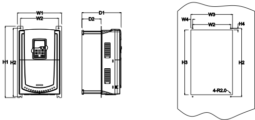
1.5-30kW 法兰安装示意图
