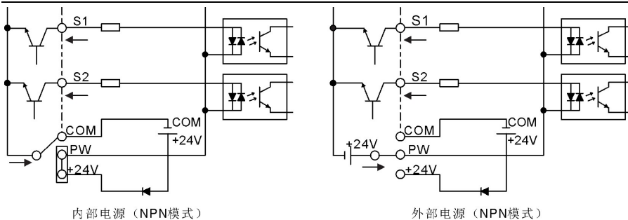
图 4-23 NPN 模式示意图
