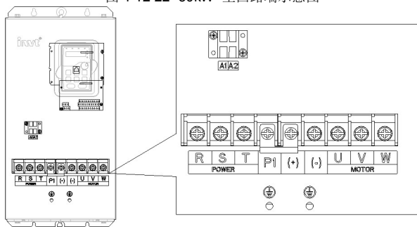
图 4-13 37~55kW 主回路端示意图
