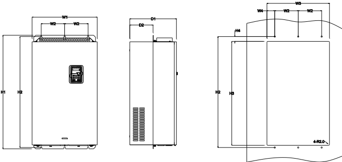
132-200kW 法兰安装示意图 法兰安装尺寸表（单位：mm）
