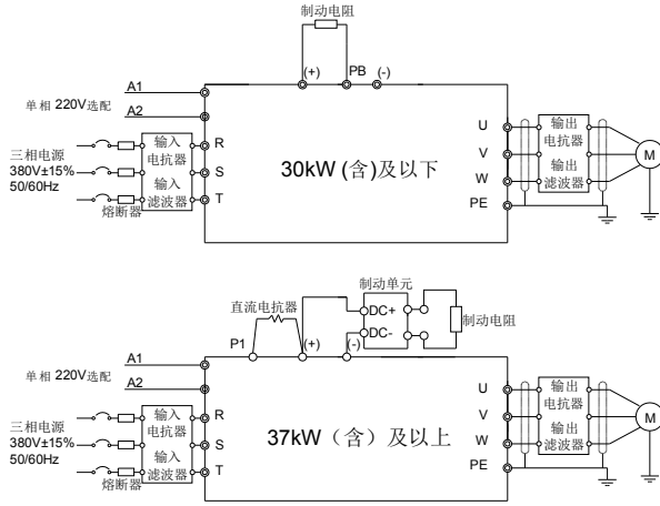
图 4-7 主回路接线图
