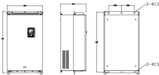
132-200kW 壁挂安装示意图
