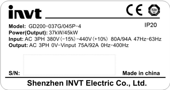
图 3-3 产品铭牌
