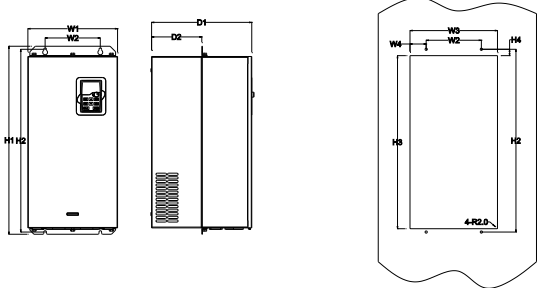
37-110kW 法兰安装示意图
