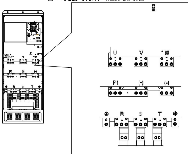
图 4-17 350~500kW 主回路端示意图
