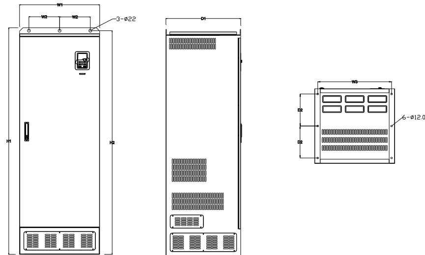
50-500kW 落地安装示意图
