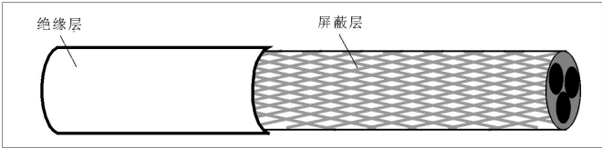
电缆剖面
