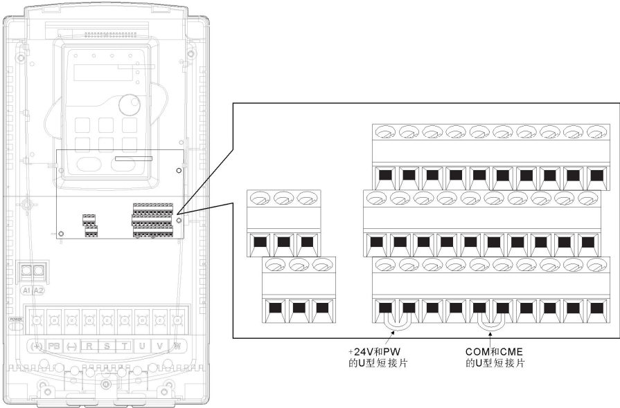
图 4-22 U 型短接位置示意图
