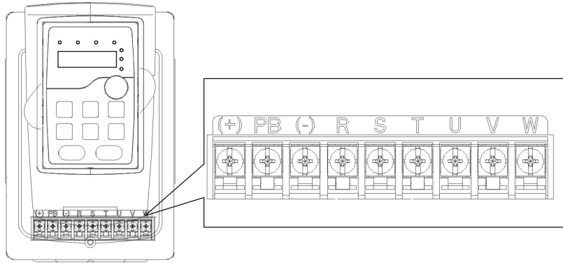
图 4-8 1.5~2.2 kW 主回路端子示意图
