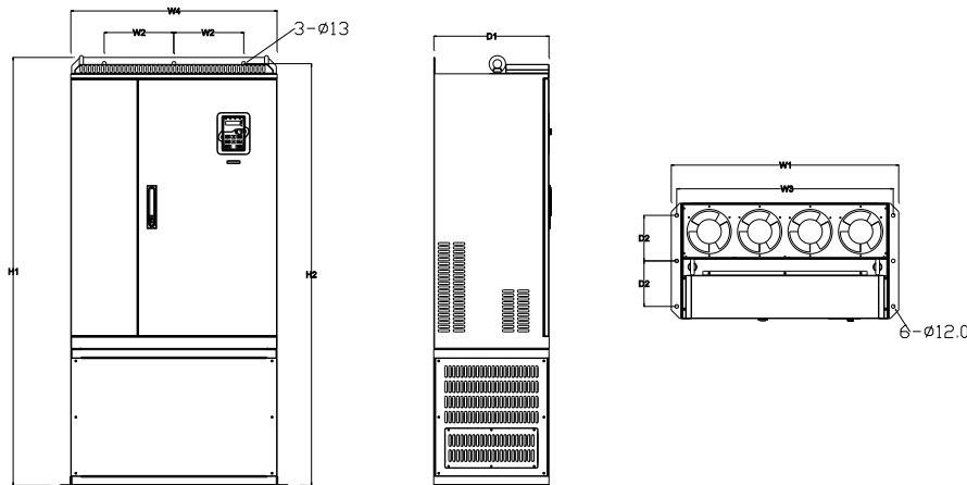
220-315kW 落地安装示意图
