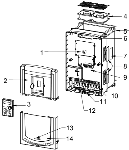
图 3-4 产品结构示意图
