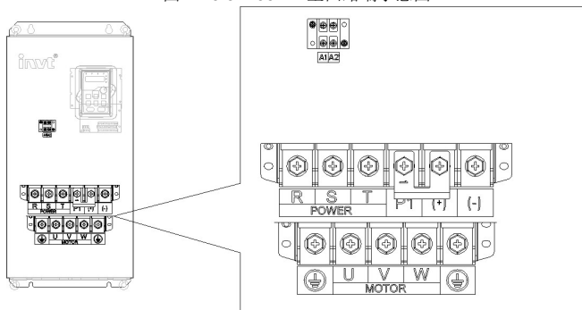
图 4-14 75~110kW 主回路端示意图
