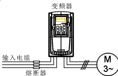
图 4-25 熔断器配置图
