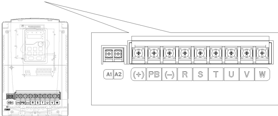
图 4-11 15~18kW 主回路端示意图
