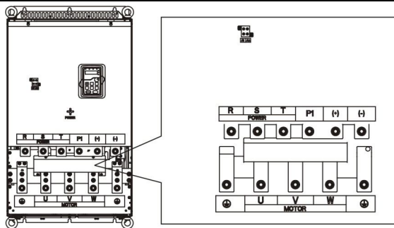
图 4-15 132~200kW 主回路端示意图
