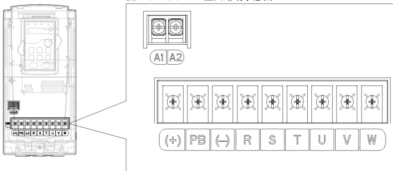
图 4-10 7.5~11kW 主回路端示意图
