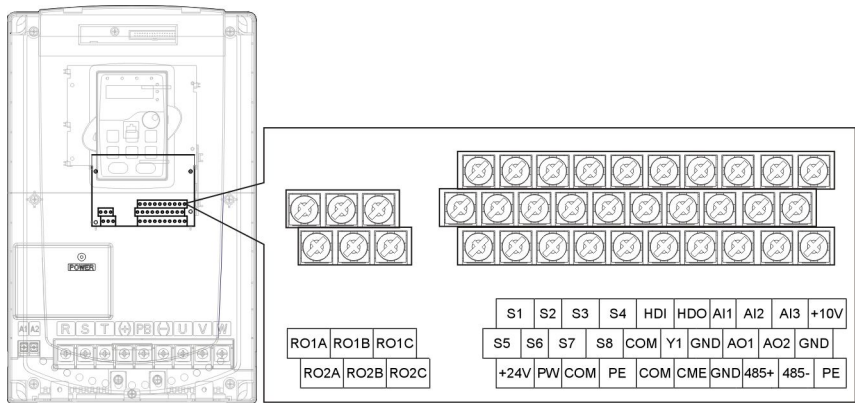
图 4-21 控制端子示意图
