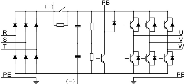
图 3-1 主回路简图 (小于 30kW (含))
