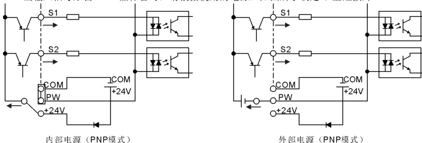
图 4-24 PNP 模式示意图
