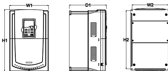
1.5-30kW 壁挂安装示意图
