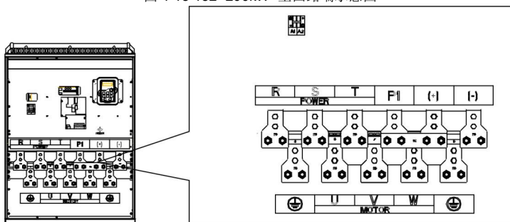
图 4-16 220~315kW 主回路端示意图
