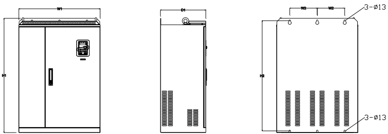
220-315kW 壁挂安装示意图 壁挂安装尺寸表（单位：mm）
