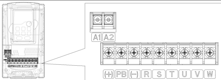
图 4-9 4~5.5 kW 主回路端示意图
