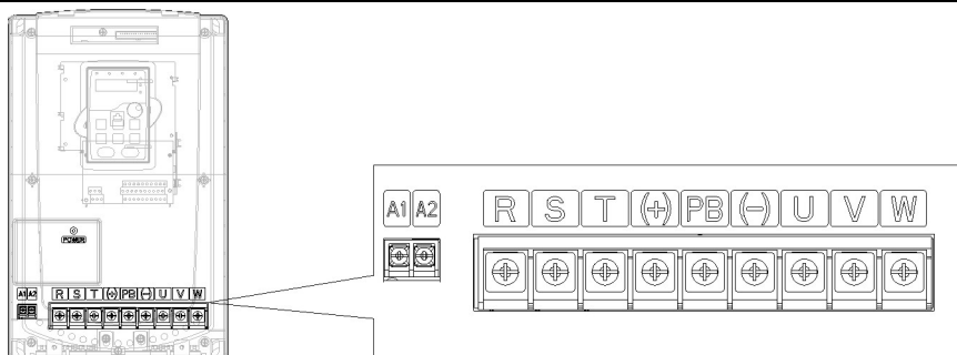
图 4-12 22~30kW 主回路端示意图
