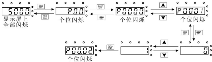
注意：在设定数值时,利用 能快速移位,或者通过 + 来调整。 图 5-3 修改参数示意图
