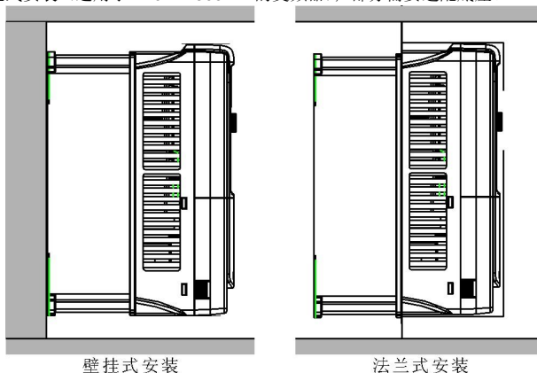
图 4-2 安装方式
