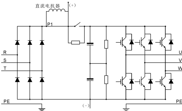
图 3-2 主回路简图 (大于 37kW (含))
