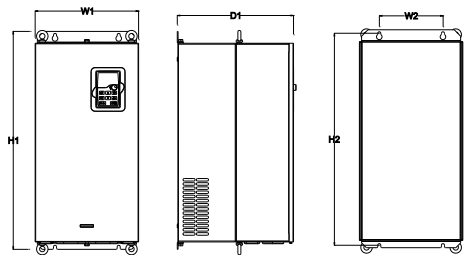
37-110kW 壁挂安装示意图
