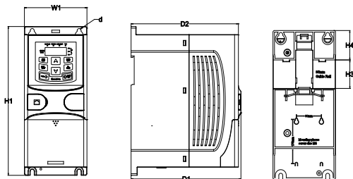
图 B-5 单相 220V 2.2kW(含)以下/三相 380V 4kW(含)以下导轨安装示意图
