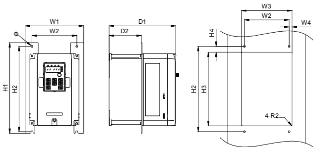
图 B-7 三相 380V 5.5~7.5kW 法兰安装示意图
