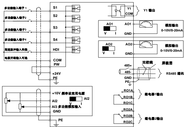
图 3-8 5.5kW 以上控制回路接线图
