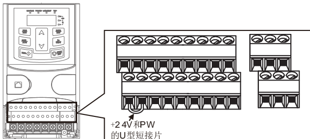
图 3-11 U 型短接位置示意图
