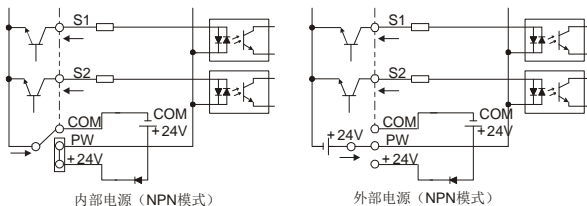
图 3-12 NPN 模式示意图
