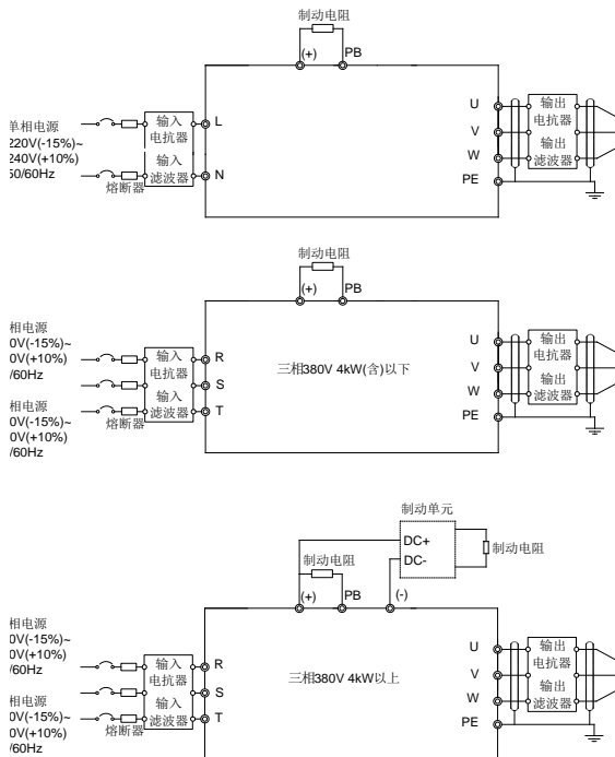
图 3-3 主回路接线图
