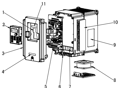
图 2-4 三相 380V 4kW 以上产品结构示意图
