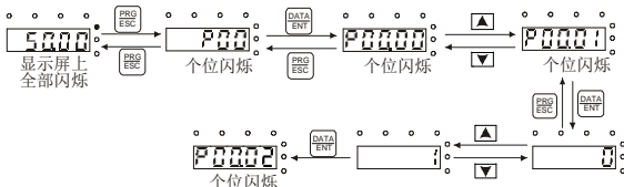
图 4-4 修改参数示意图
