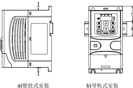
图 3-1 安装方式
