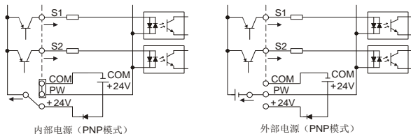
图 3-13 PNP 模式示意图
