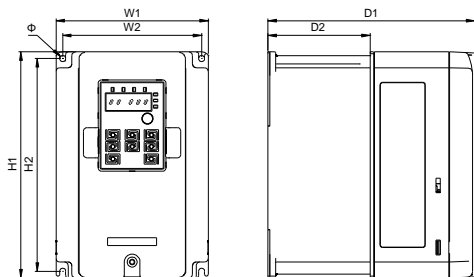
图 B-6 三相 380V 5.5~7.5kW 壁挂安装示意图
