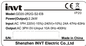
图 2-1 产品铭牌
