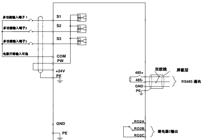
图 3-7 5.5kW(含)以下控制回路接线图
