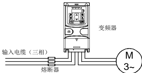
图 3-14 熔断器配置图
