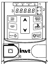
图 4-1 贴膜键盘示意图
