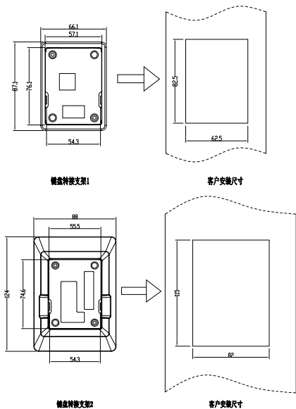
图 B-3 外形尺寸与安装尺寸图
