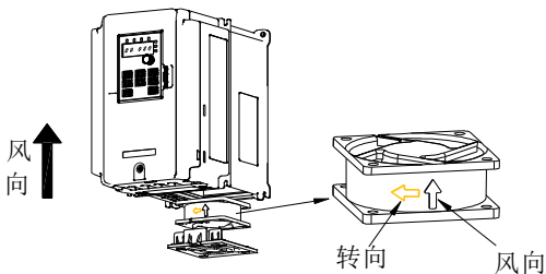
图 6-2 三相 380V 4kW 以上机器风扇维护示意图
