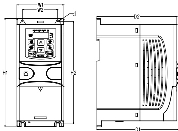
图 B-4 单相 220V 2.2kW(含)以下/三相 380V 4kW(含)以下壁挂安装示意图
