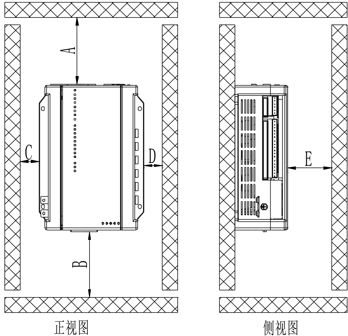
图 5-3 RCU 控制单元安装空间示意图
