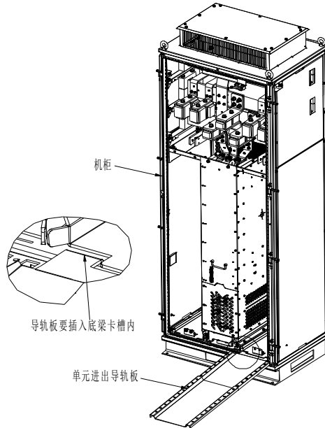
图 3-16 单元进出导轨板放置示意图
