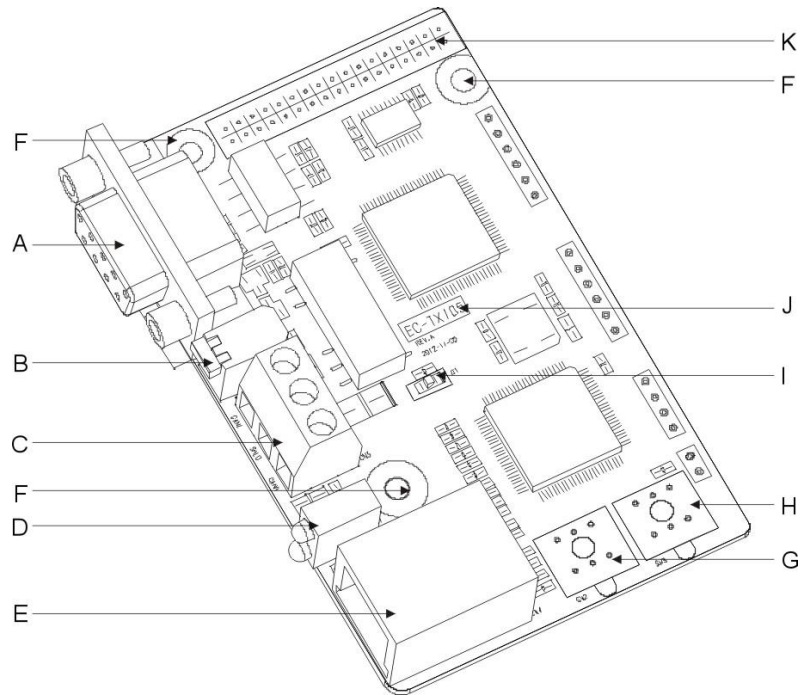
图 B-5 EC-TX105 系列通讯卡外形图
