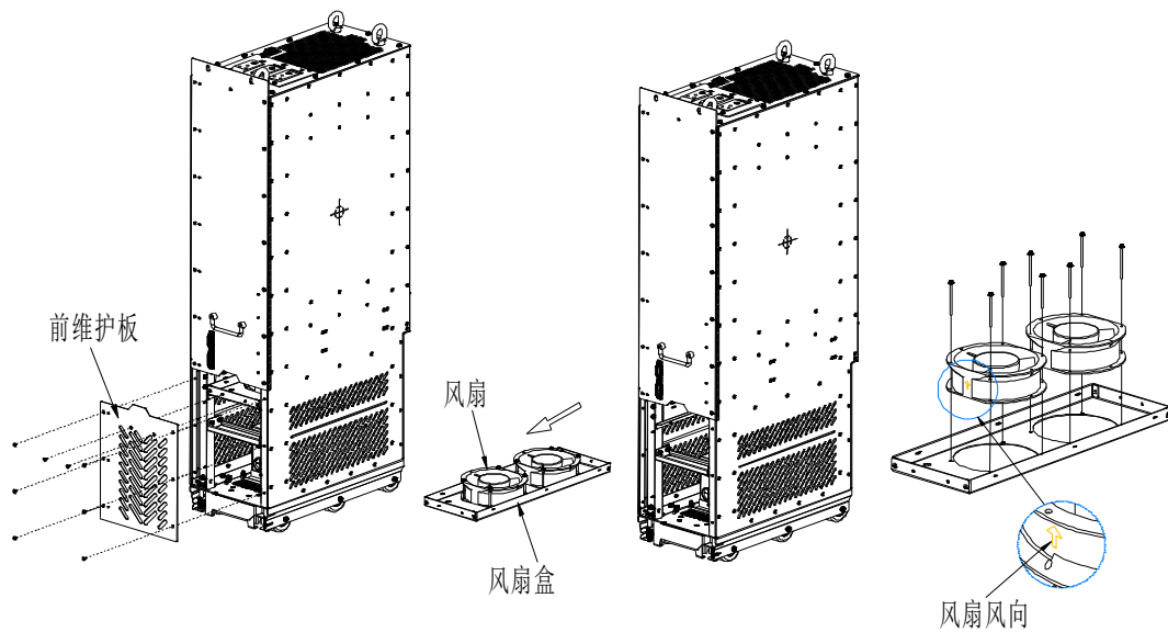
图 6-2 回馈整流滤波器风扇维护示意图
