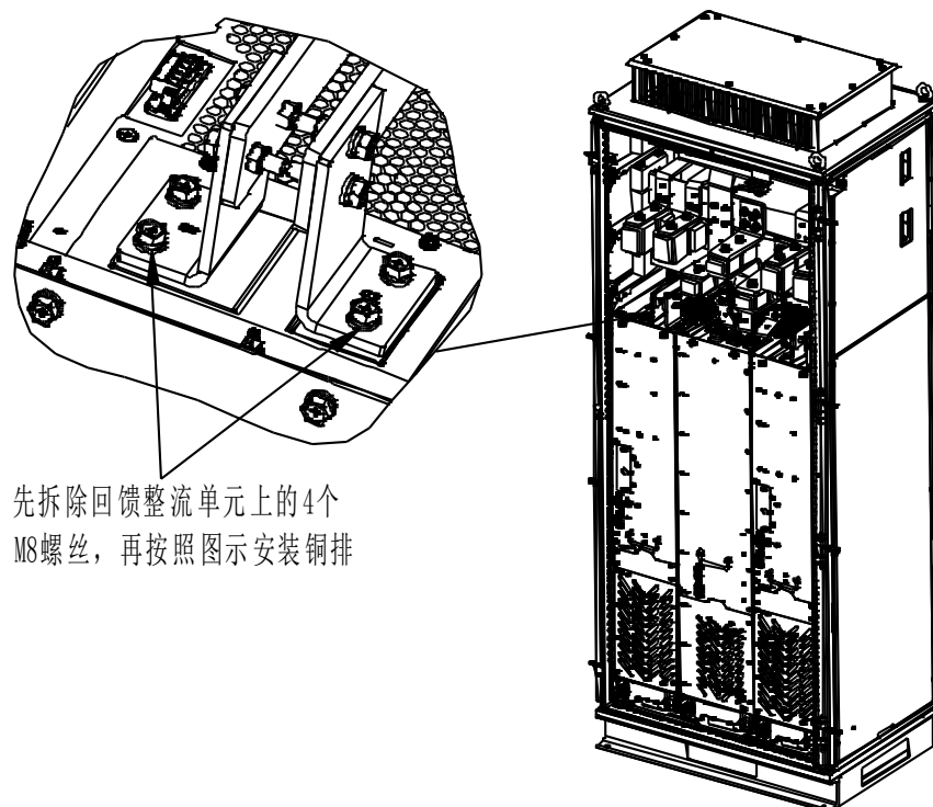
图 3-21 单元安装顶部铜排示意图
