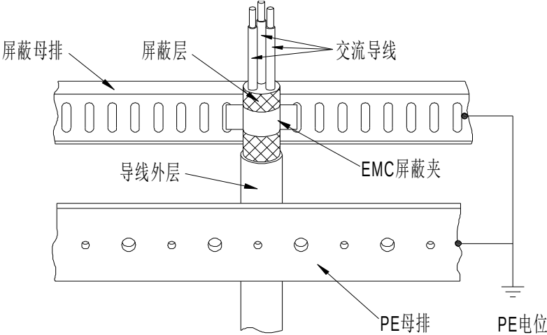
图 4-8 功率电缆屏蔽连接示意图
