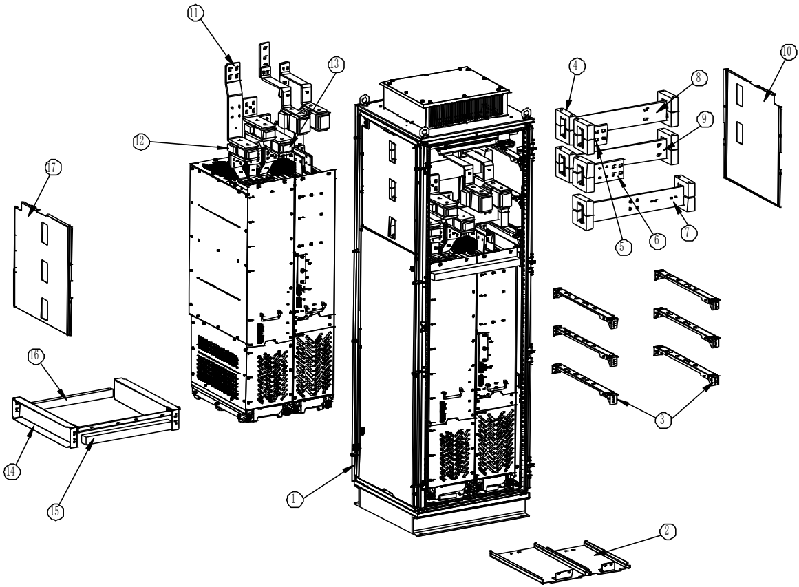
图 3-13 L+A8-600 柜体安装示意图
