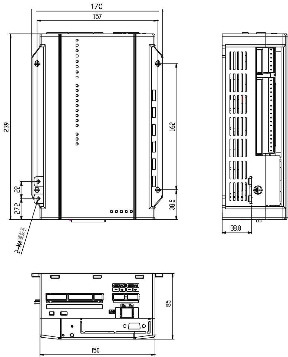
图 5-2 RCU 控制单元尺寸图（单位：mm）
