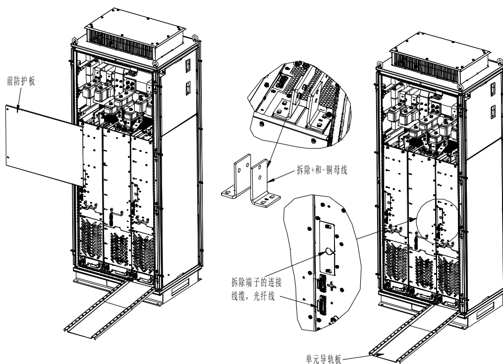
图 6-6 回馈整流单元更换示意图
