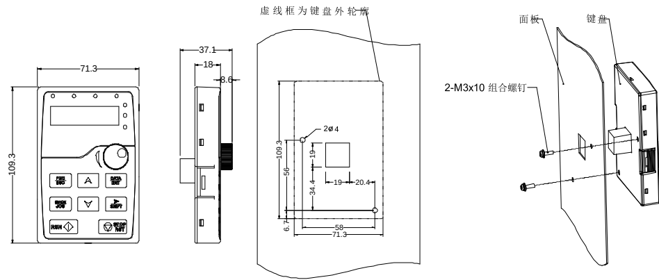
图 3-22 LED 键盘结构图
