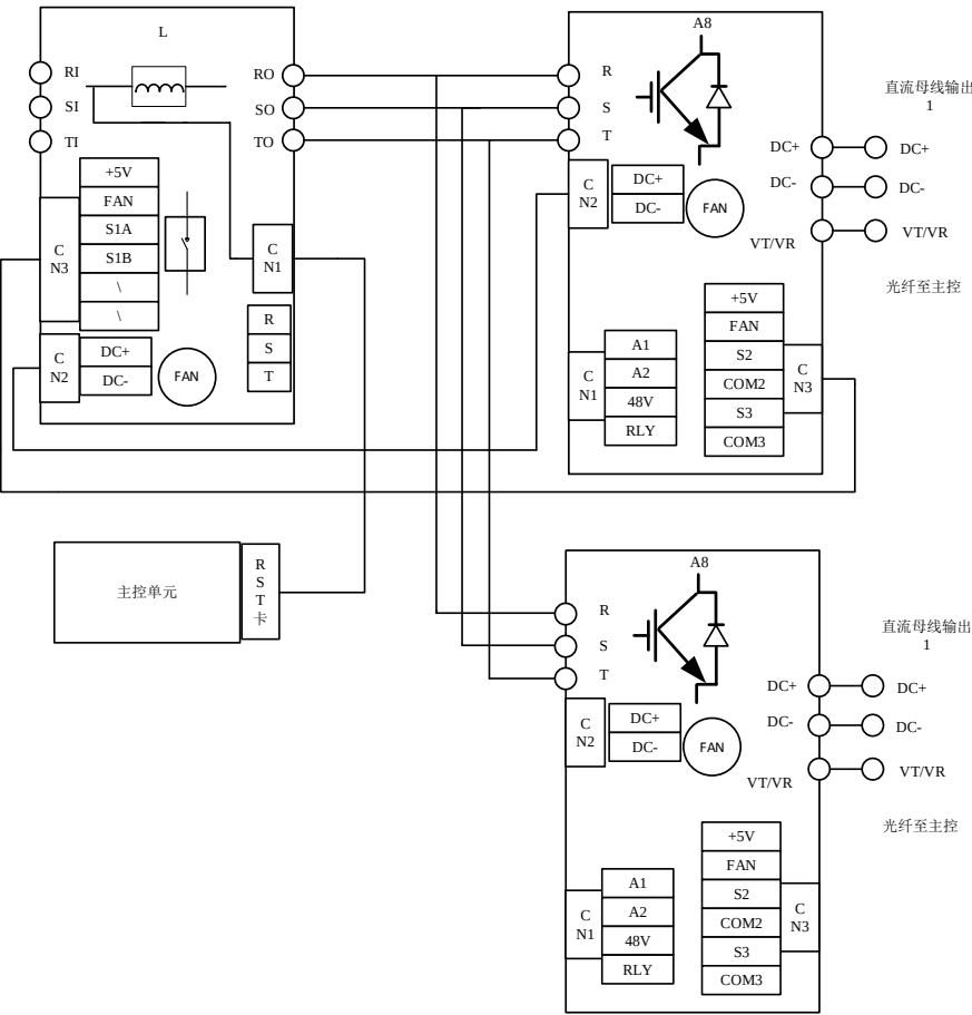
图 4-9 回馈整流接线图
