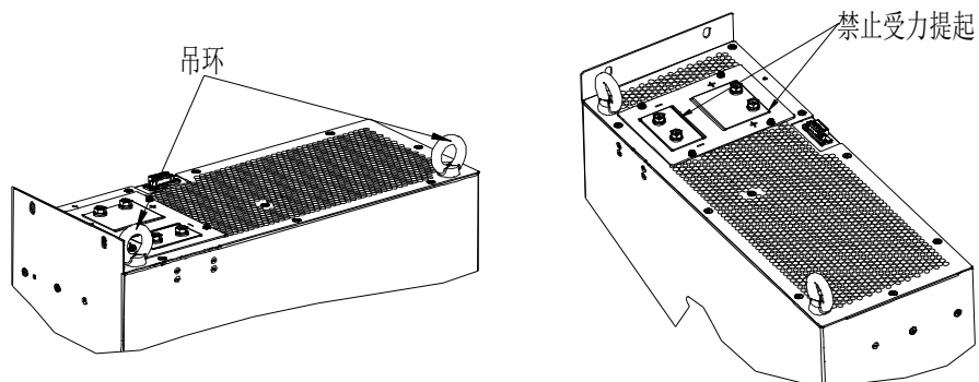
图 3-5 单元顶部示意图
