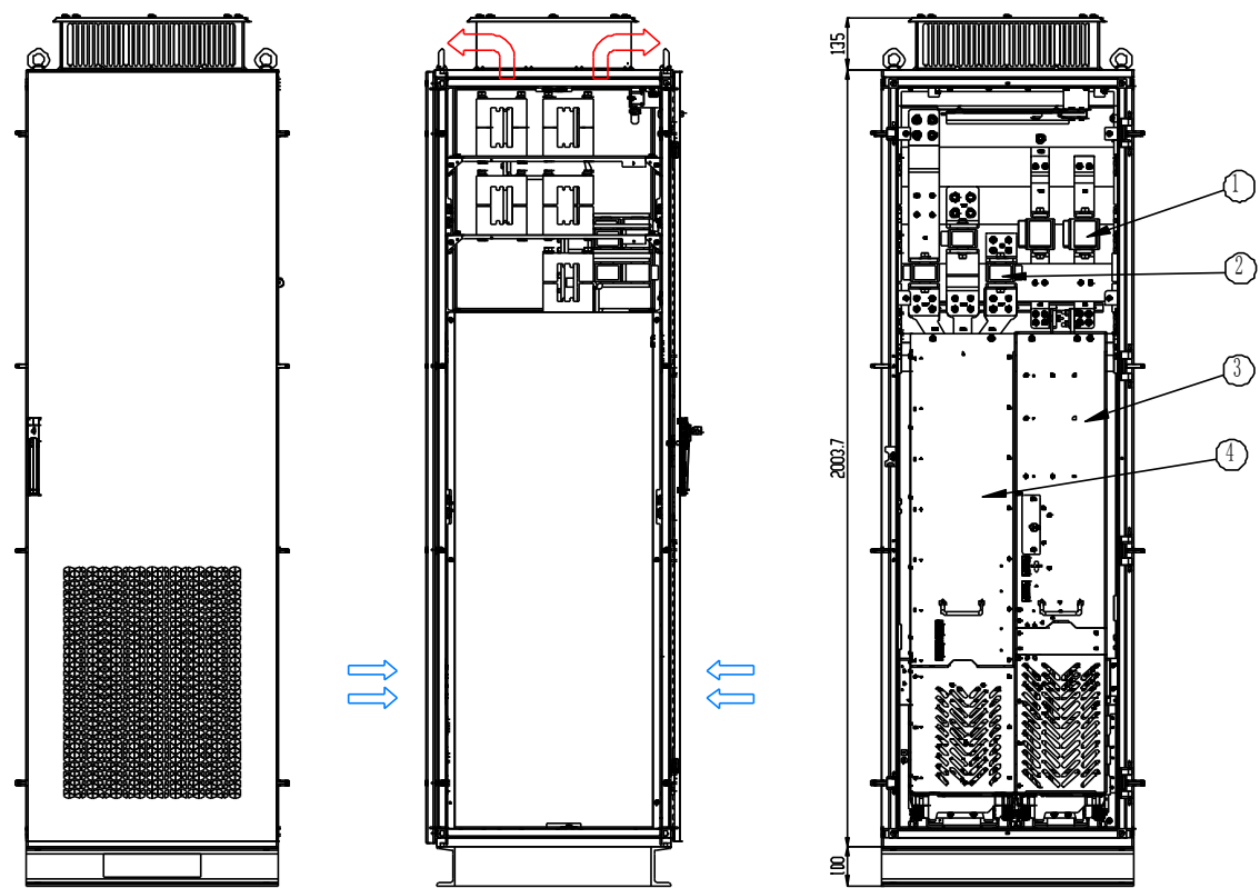
图 3-12 L+A8-600 柜体布局
