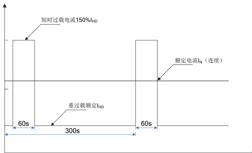
图 2-4 重过载应用
