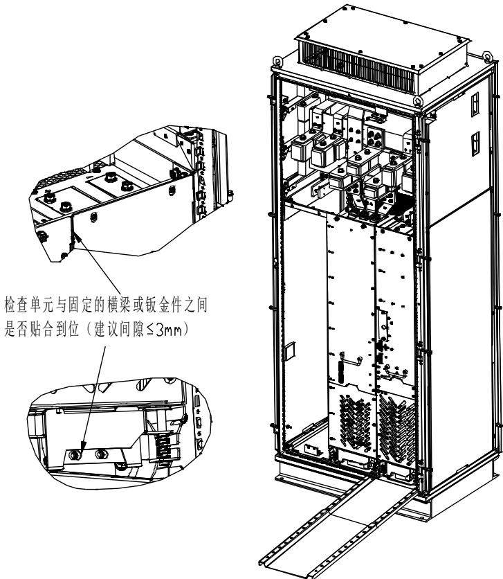
图 3-19 单元推入到位检查示意图
