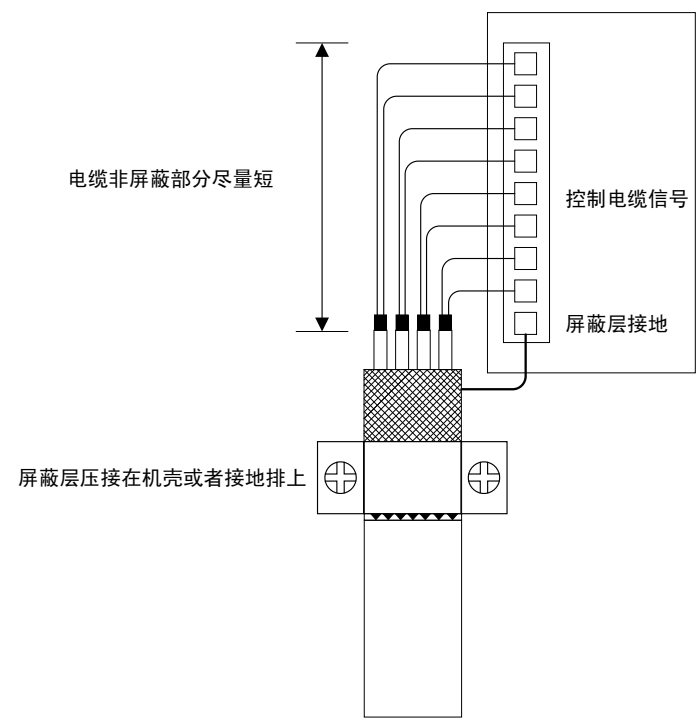
图 4-7 控制电缆屏蔽连接示意图
