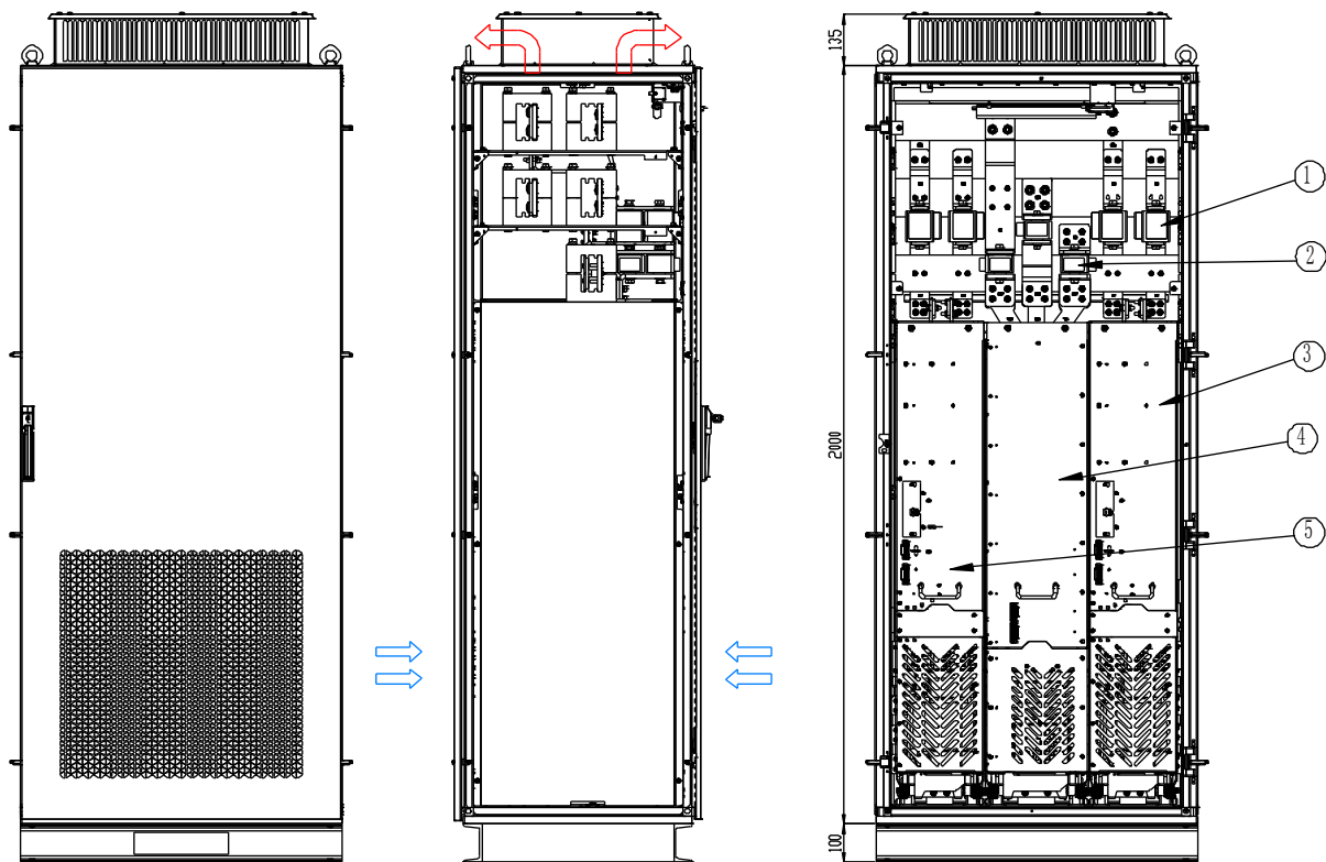
图 3-14 L+2*A8 柜体布局
