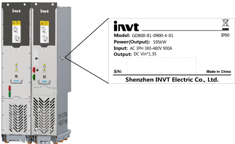
图 2-1 产品铭牌
