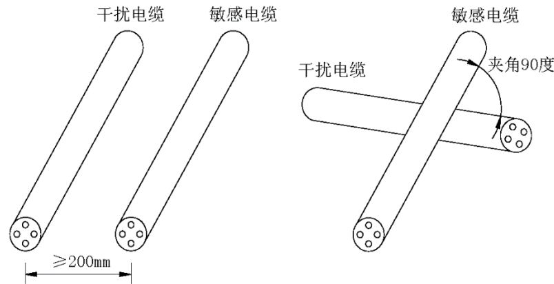
图 4-4 敏感电缆与干扰电缆布线示意图
