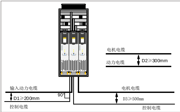
图 4-3 电缆布置一般原则
