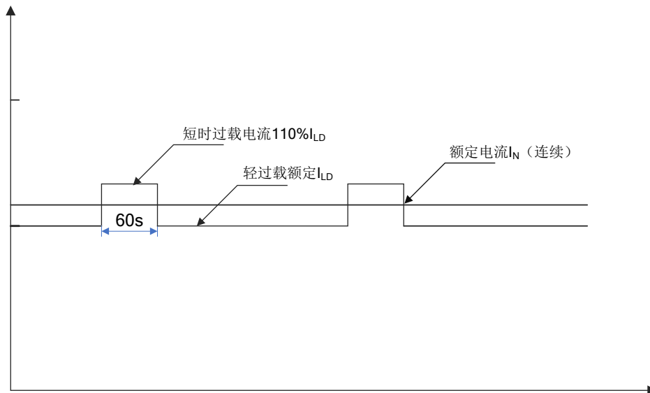
图 2-3 轻过载应用
