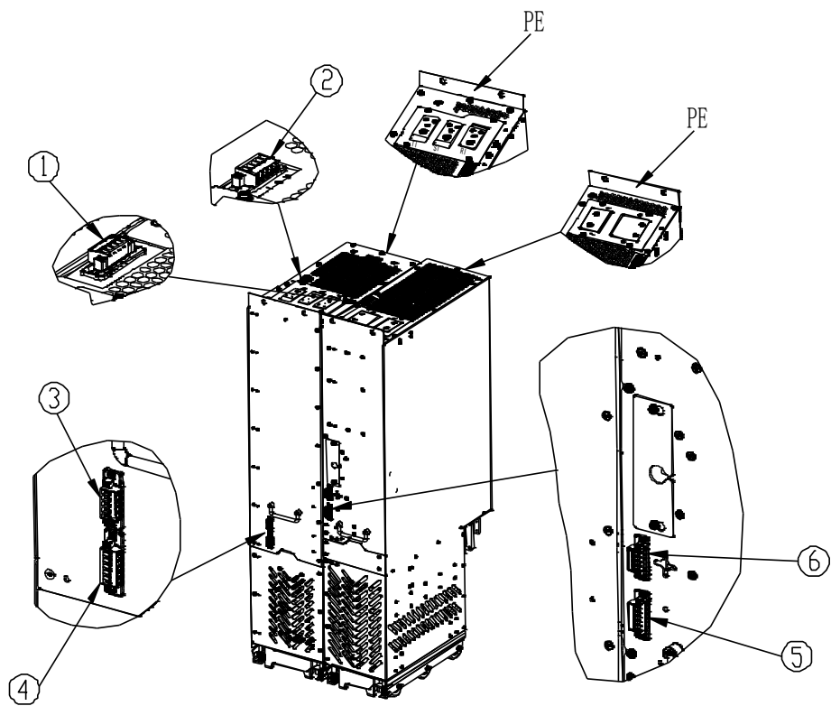
图 4-10 回馈整流滤波接线端子示意图
