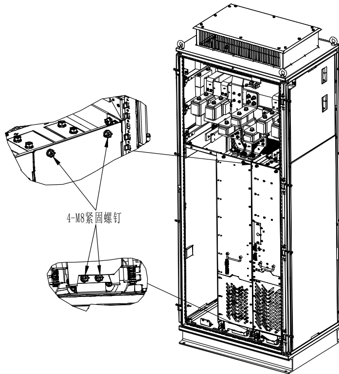
图 3-20 单元固定示意图
