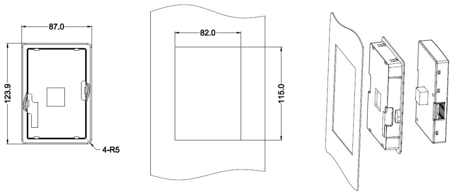
图 3-23 键盘支架安装图
