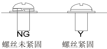
图 4-11 螺丝安装要求图
