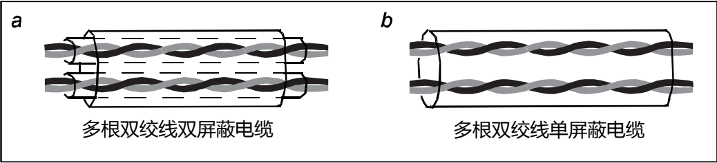
图 4-2 控制电缆
