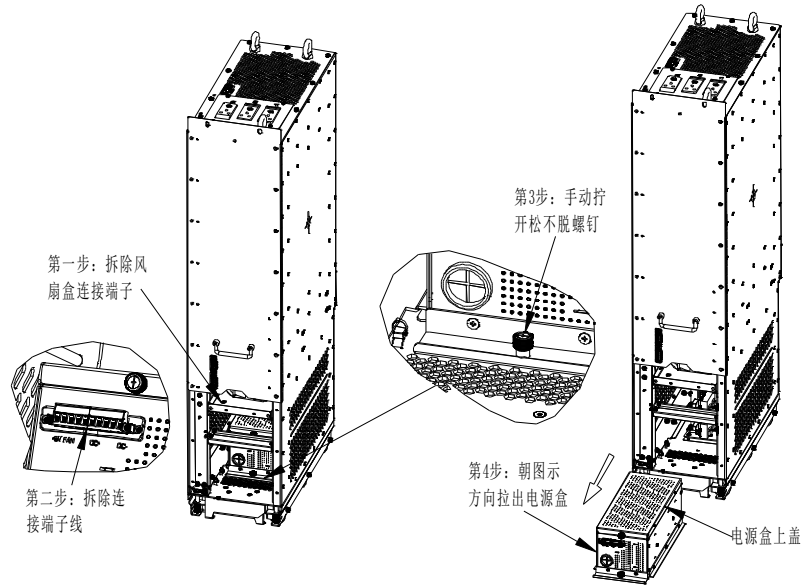
图 6-4 回馈整流滤波器拆电源盒示意图
