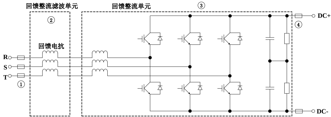
图 2-5 回馈整流主回路简图
