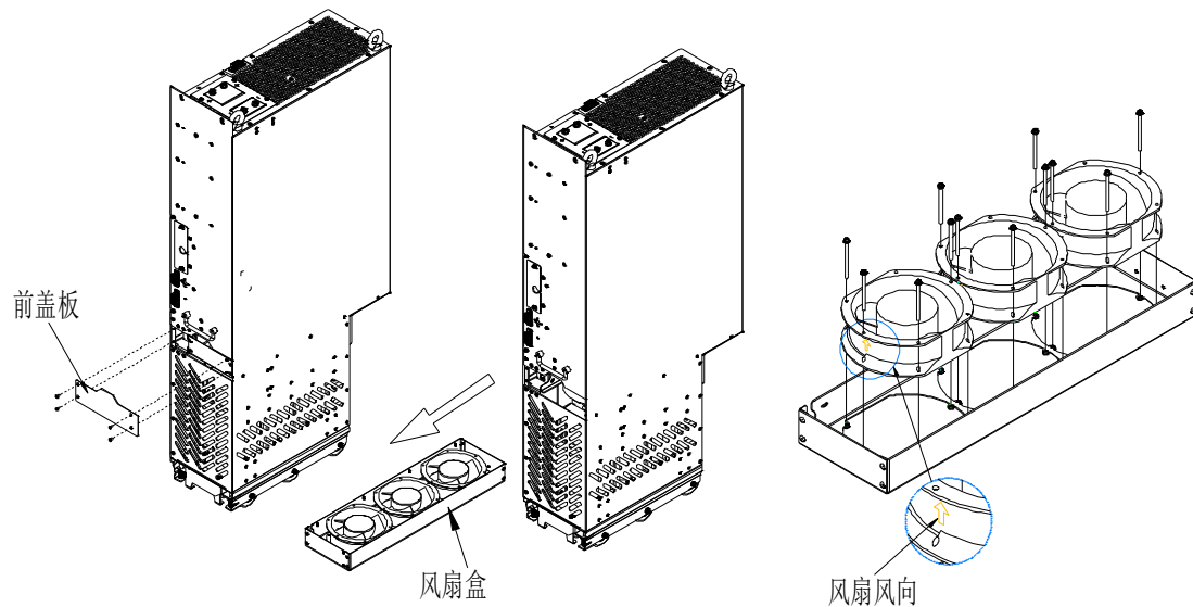
图 6-1 回馈整流单元风扇维护示意图
