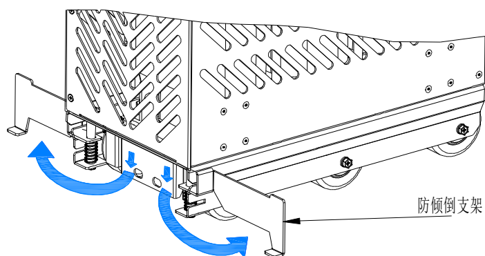
图 3-7 打开防倾倒支架示意图
