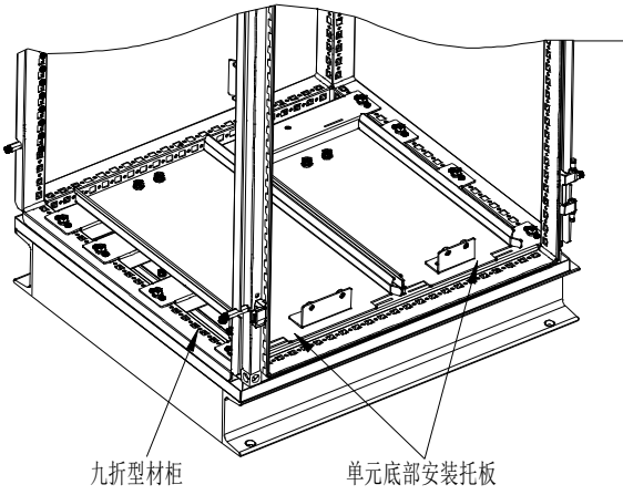
图 3-11 安装单元托盘
