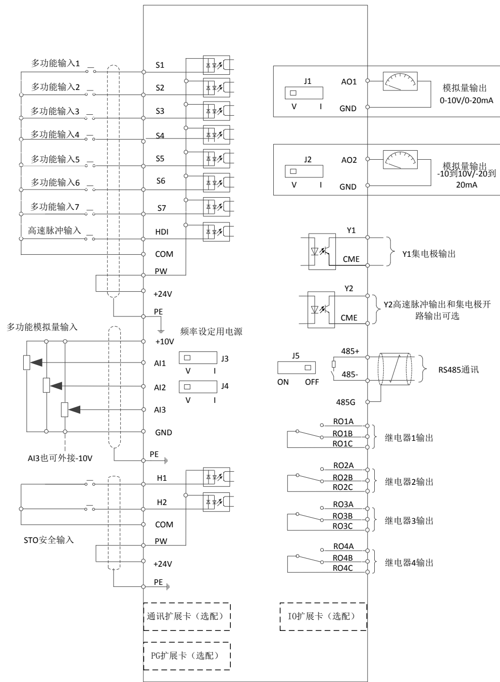
图 5-5 RCU 控制单元接口示意图
