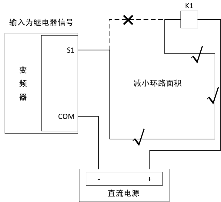
图 4-5 非差分信号布线环路示意图
