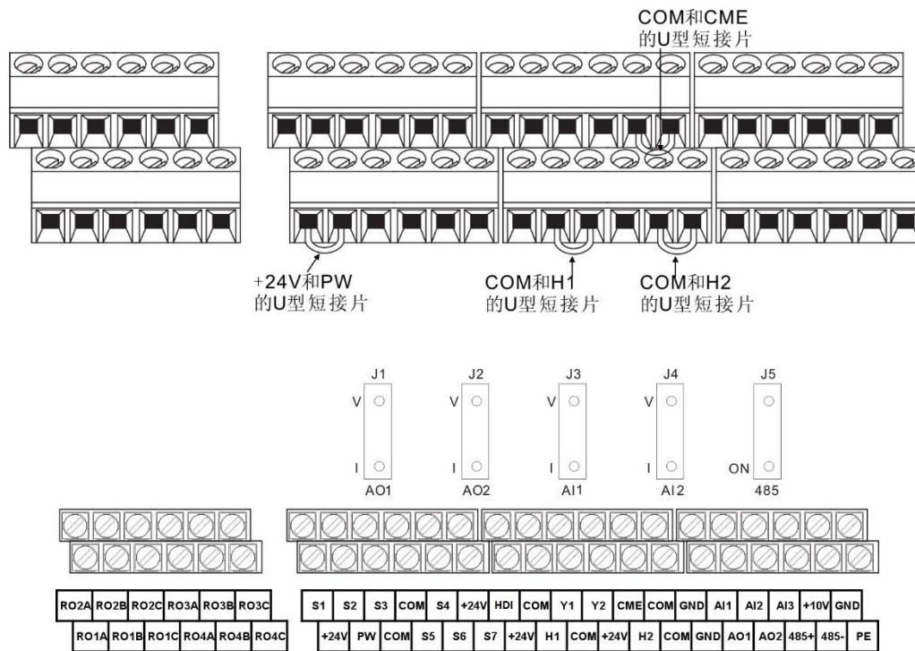
图 5-6 RCU 控制单元接口端子示意图
