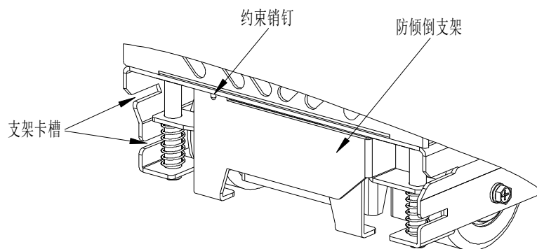
图 3-6 单元底部示意图
