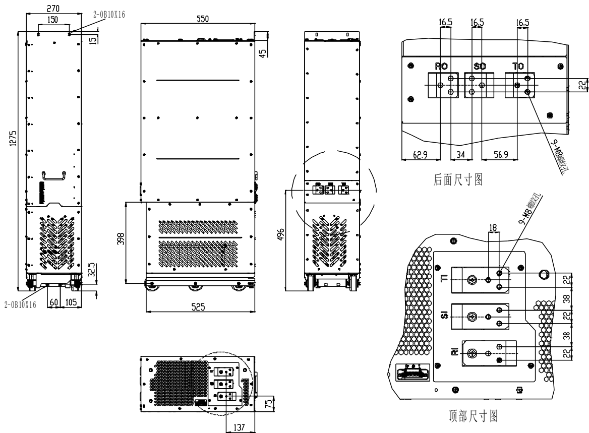
图 C-1 安装尺寸图
