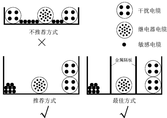
图 4-6 多种电缆敷设示意图
