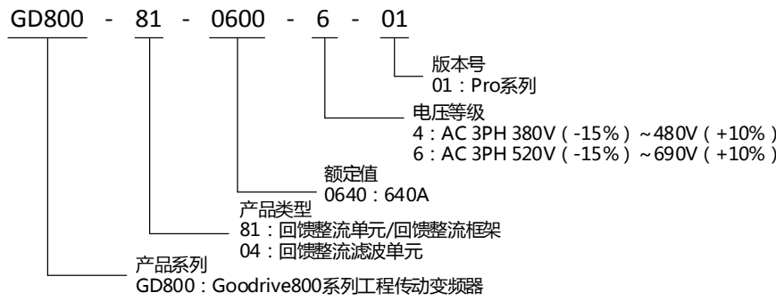
图 2-2 产品型号
