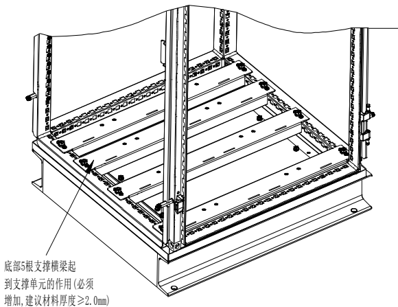
图 3-10 安装支撑横梁示意图
