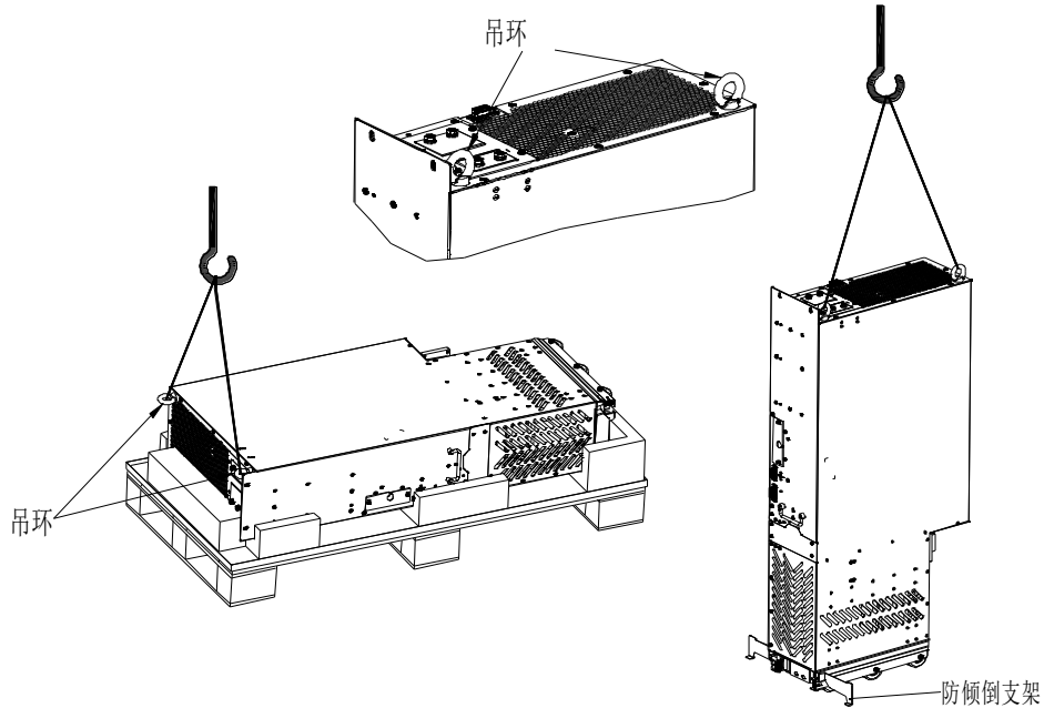
图 3-4 单元吊装示意图
