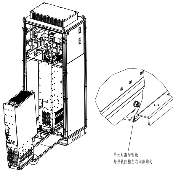
图 3-17 单元入柜放置示意图
