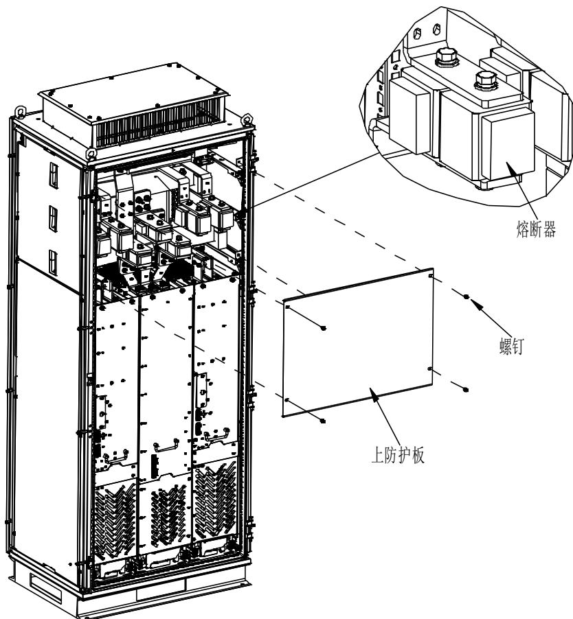
图 6-5 回馈整流滤波器更换熔断器示意图
