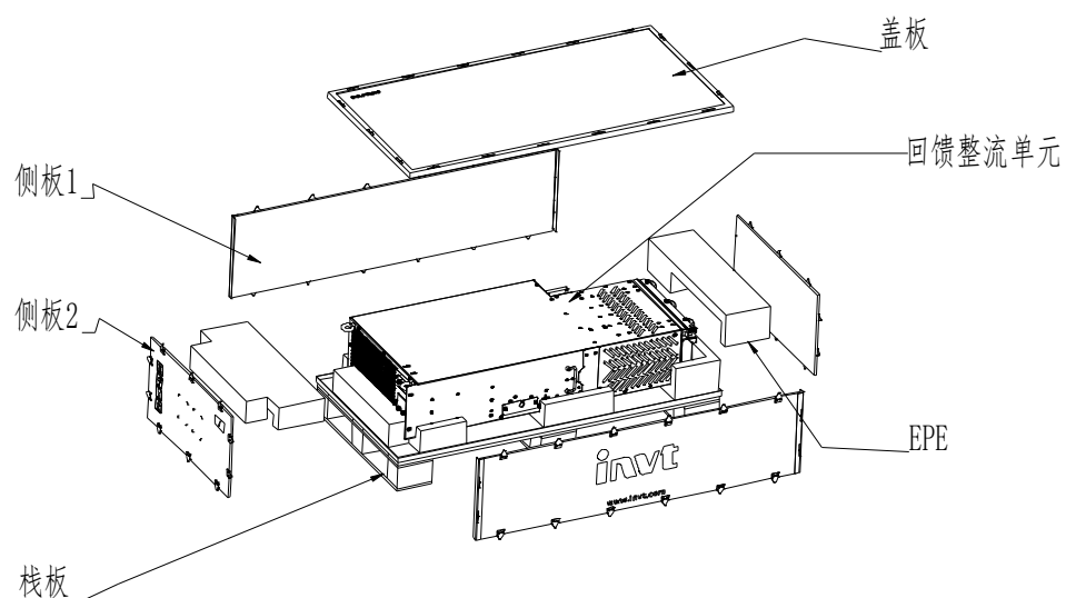
图 3-3 拆封示意图
