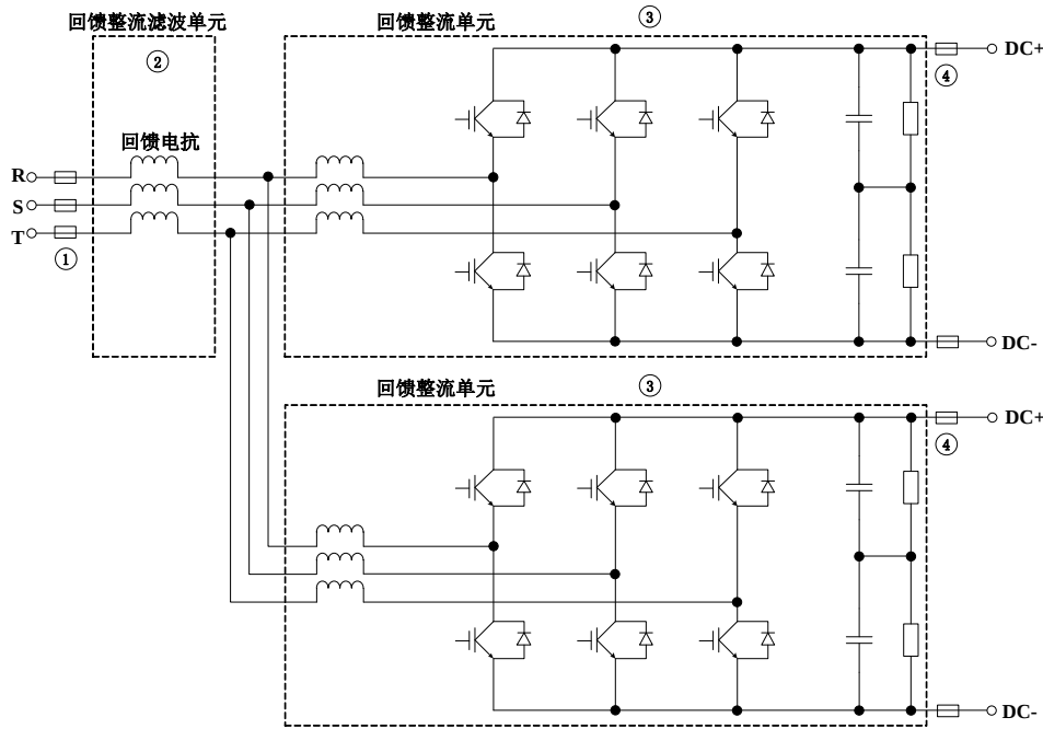
图 2-6 回馈整流并机系统简图
