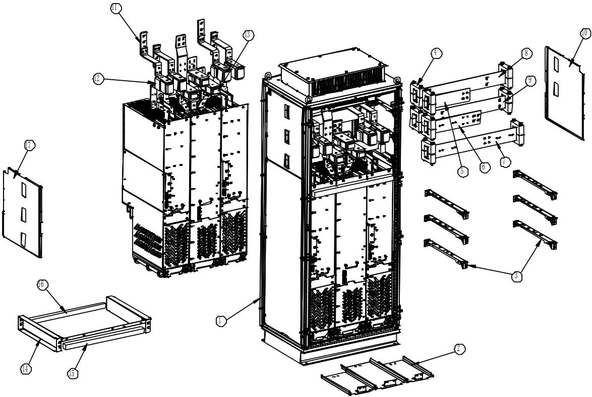
图 3-15 L+2*A8-850 柜体安装示意图
