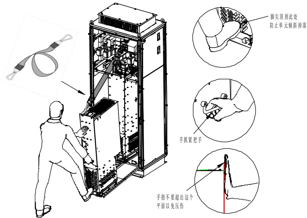
图 3-18 回馈整流单元入柜示意图
