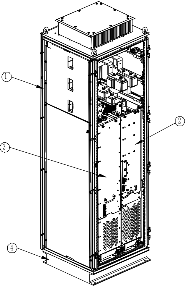
图 2-7 回馈整流框架（L+A8）结构示意图
