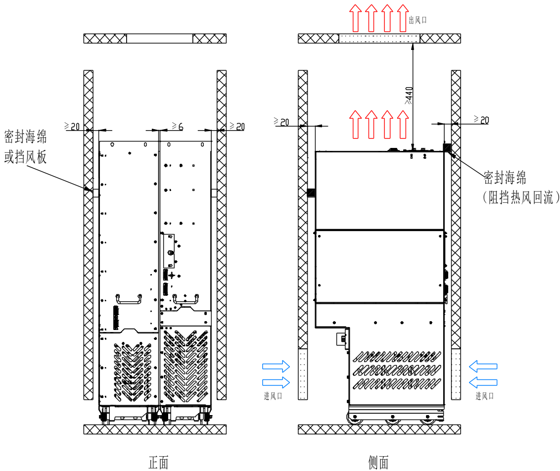
图 3-9 安装空间要求
