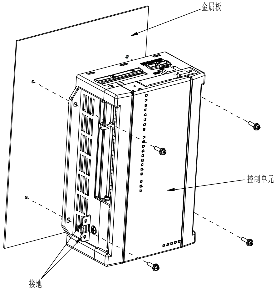
图 5-4 RCU 控制单元安装示意图
