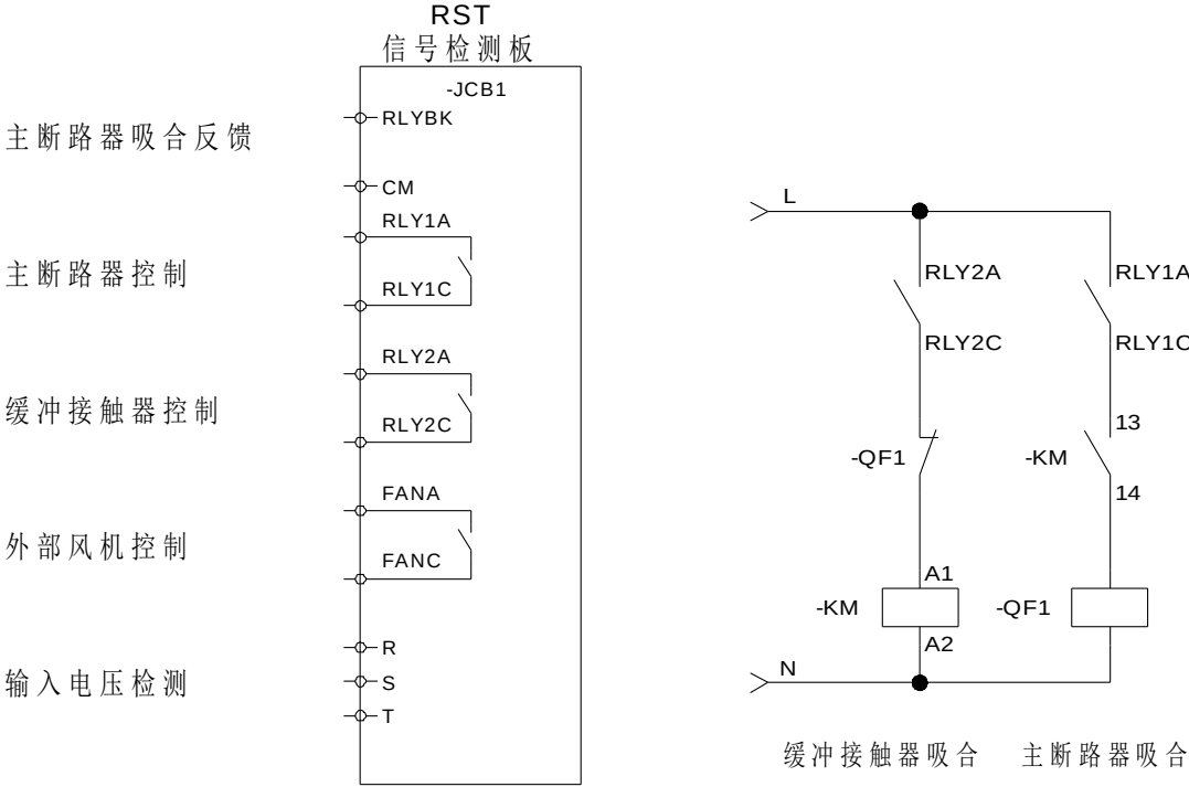
图 5-7 缓冲控制原理图
