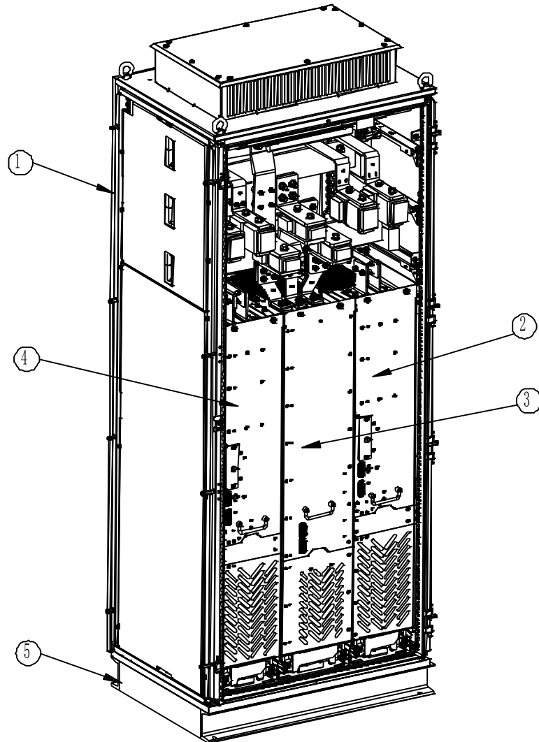
图 2-8 回馈整流框架 (L+2*A8) 结构示意图
