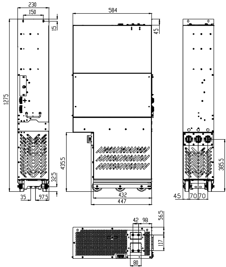
图 C-2 安装尺寸图
