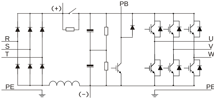
图 3-1 380V (30kW~110kW (含)) 主回路简图
