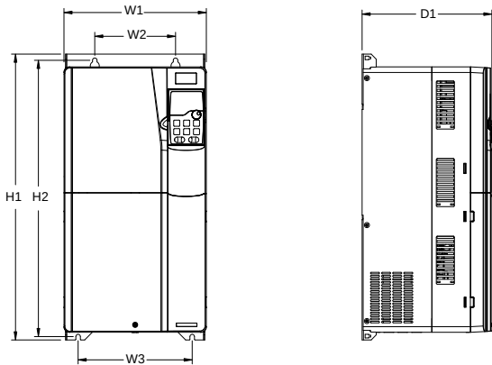
图 C-4 380V 45~75kW 壁挂安装示意图
