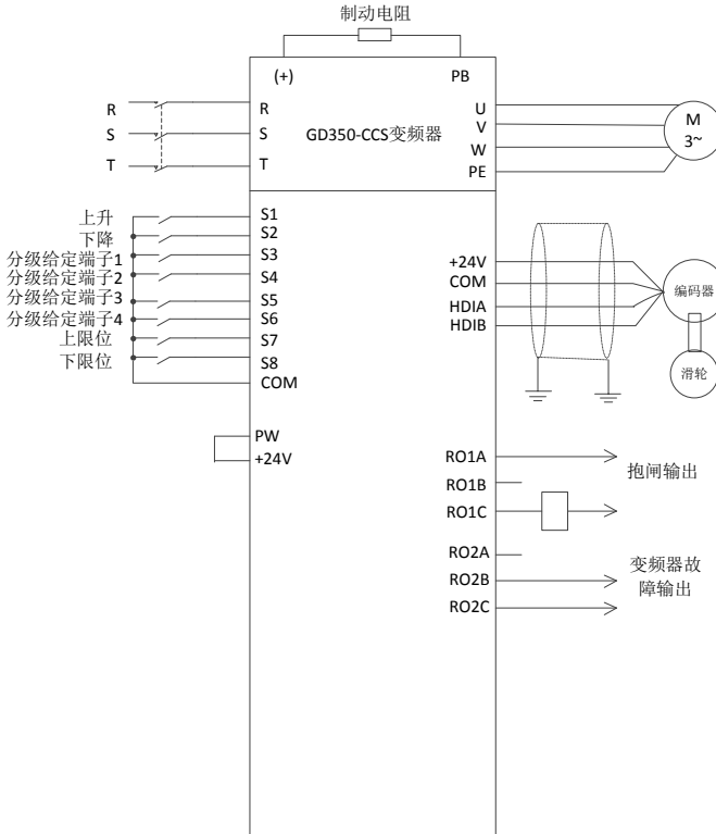
图 5-16 外部测量（HDI）接线图（开环）
