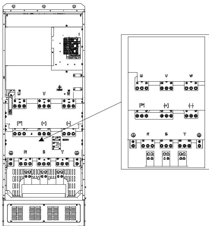
图 4-12 380V 355~500kW 主回路端子示意图
