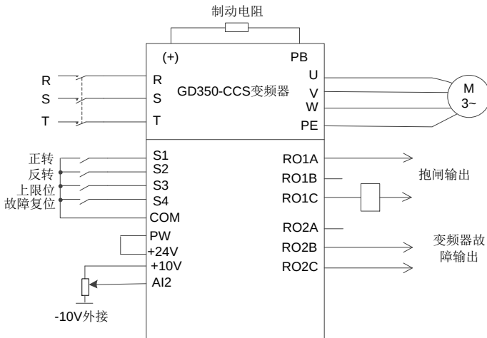
图 5-8 开环矢量卷扬应用接线参考图（选用模拟量给定选用-10V~10V）
