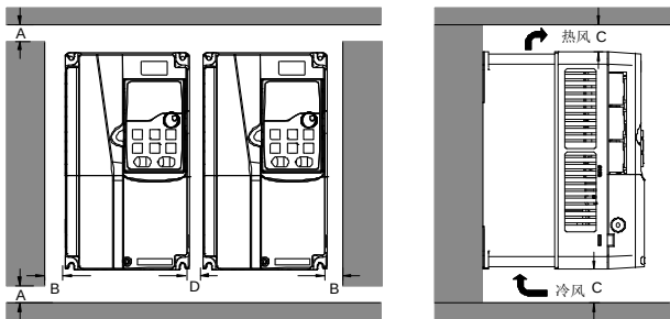
图 4-4 并行安装
