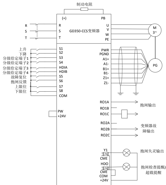
图 5-15 内部测量（电机编码器）接线图
