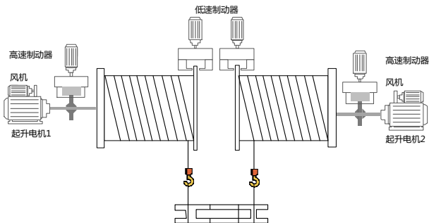
图 5-12 机械结构示意图 2
