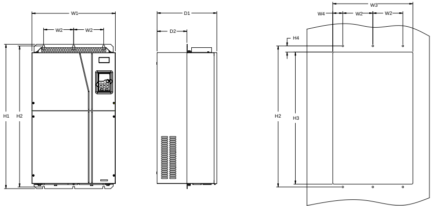
图 C-10 380V 132~200kW 法兰安装示意图
