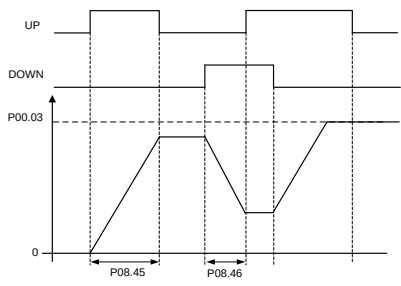
图 5-10 电动电位器调试示意图
