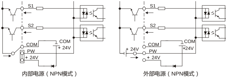
图 4-16 NPN 模式示意图
