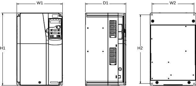
图 C-3 380V 30~37kW 壁挂安装示意图
