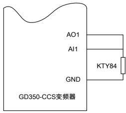
图 5-21 模拟量端口与 KTY84 接线图
