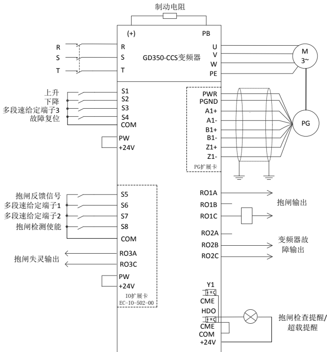
图 5-2 提升闭环矢量接线图
