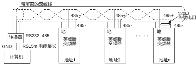
图 11-4 菊花接法运用图
