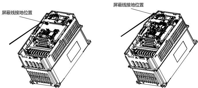
图 A-4 扩展卡地线连接示意图
