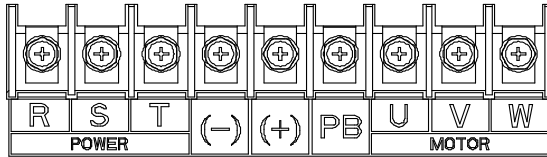
图 4-9 三相 380V 45~110kW 主回路端子示意图
