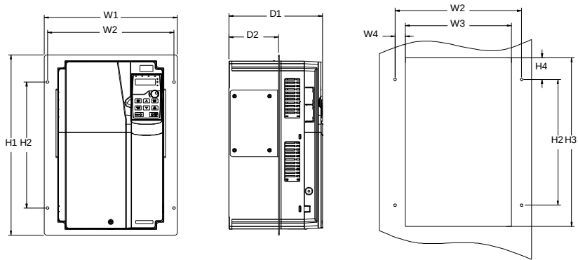
图 C-8 380V 30~75kW 法兰安装示意图
