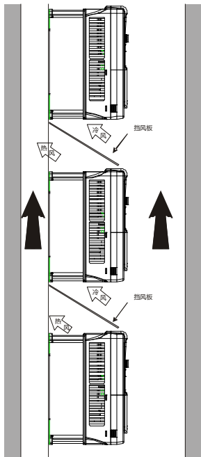
图 4-5 垂直安装
