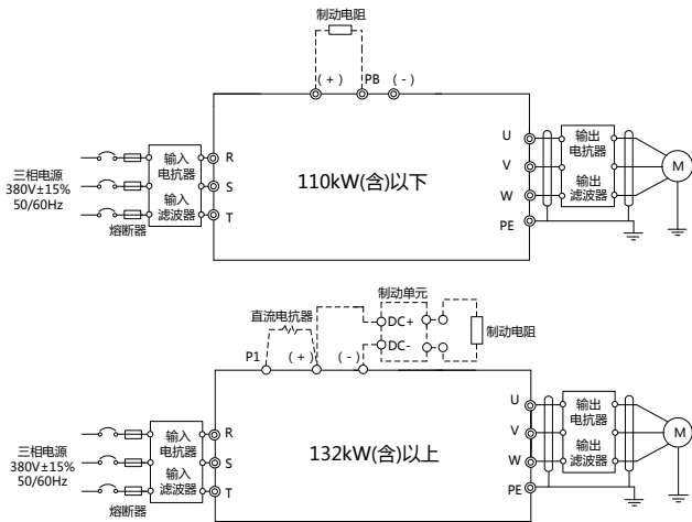
图 4-7 AC 3PH 380V~480V 主回路接线图
