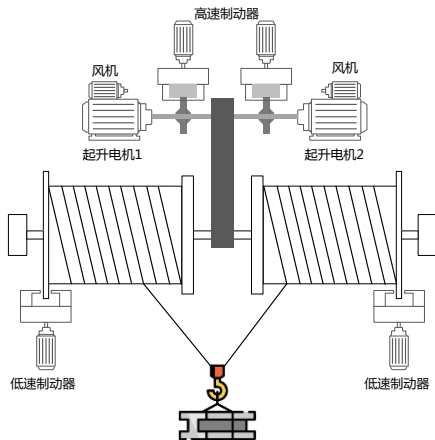
图 5-11 机械结构示意图 1
