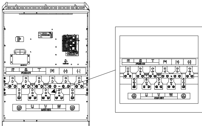
图 4-11 380V 220~315kW 主回路端子示意图
