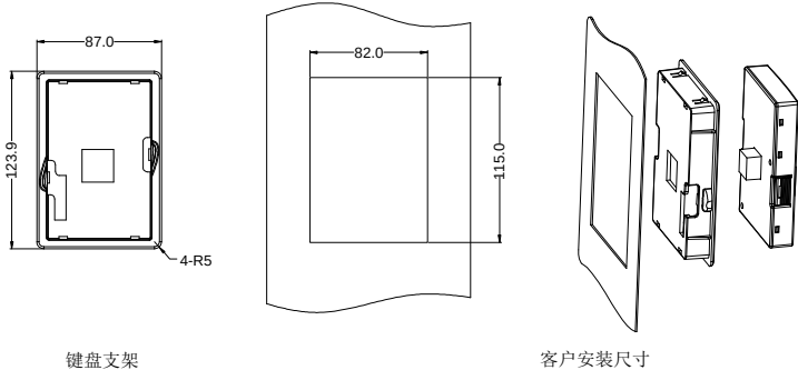
图 C-1 380V 30~500kW 键盘安装架（选配）
