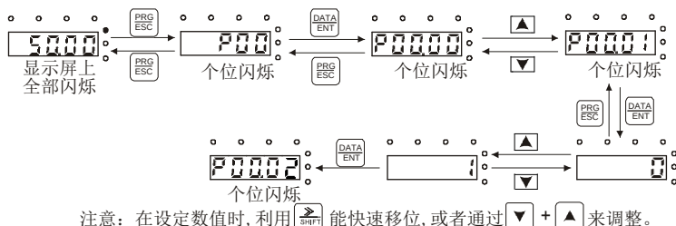
图 6-3 修改参数示意图
