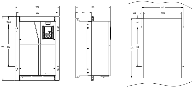
图 C-9 380V 90~110kW 法兰安装示意图
