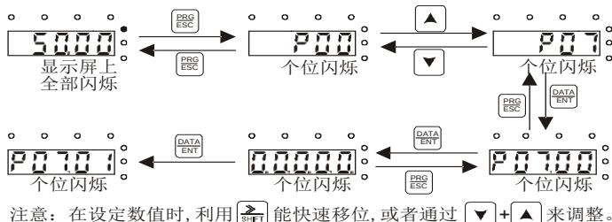
图 6-4 设定密码示意图
