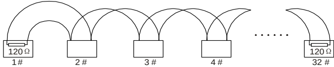
图 11-2 菊花接法现场接线图
