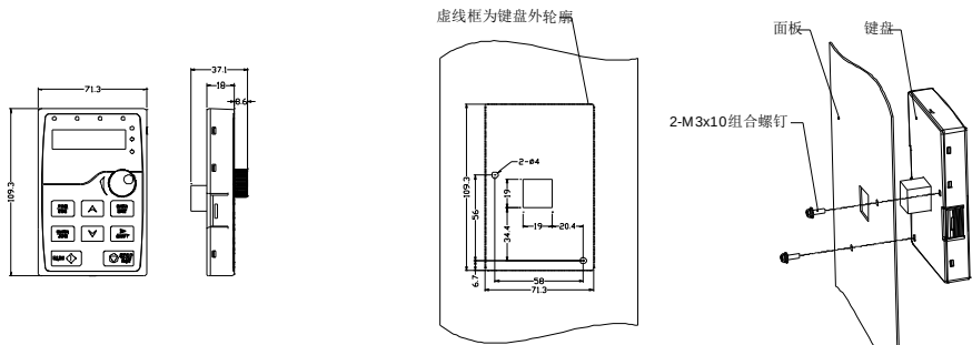
键盘无支架安装开孔尺寸及示意图
