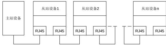
图 A-5 线型网络拓扑电气连接图
