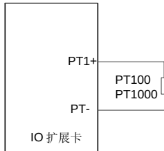
图 5-19 PT100/PT1000 使用扩展卡进行温度测量
