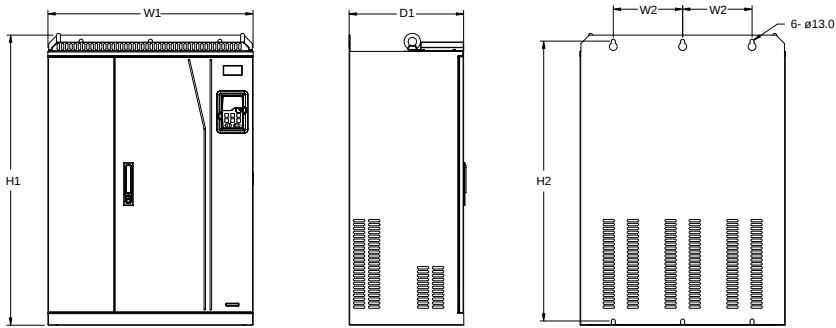
图 C-7 380V 220~315kW 壁挂安装示意图
