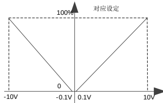
图 5-6 AI2 模拟量输入对应频率设定（选用模拟量给定选用-10V~10V）
