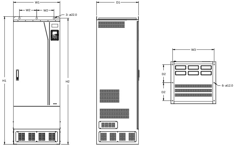
图 C-12 380V 355~500kW 落地安装示意图
