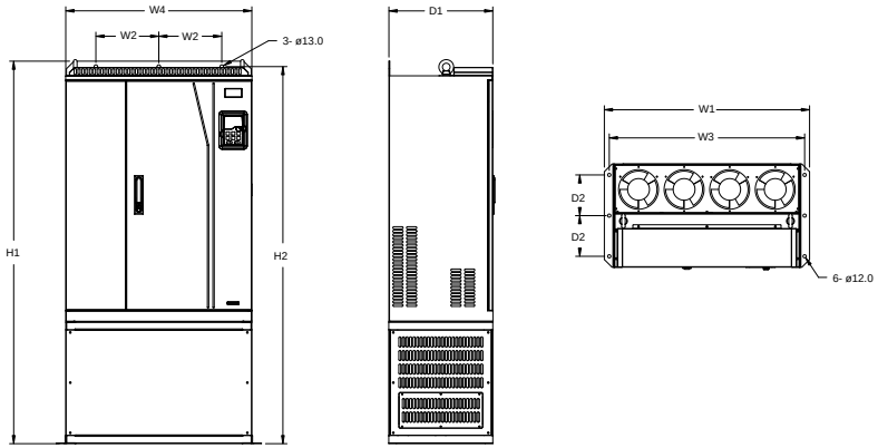
图 C-11 380V 220~315kW 落地安装示意图
