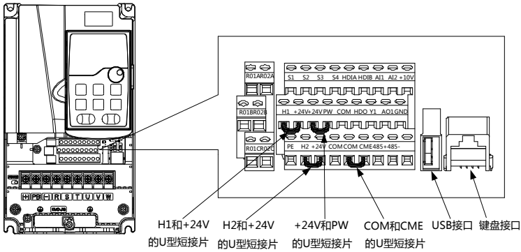
图 4-15 U 型短接位置示意图
