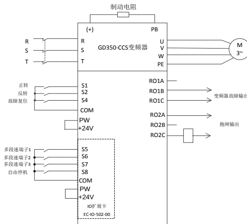
图 5-3 平移应用调试
