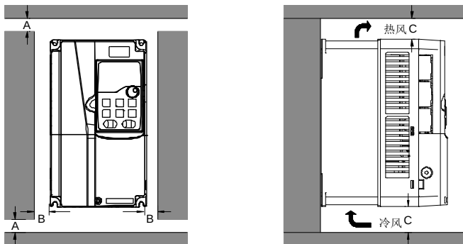
图 4-3 单台安装
