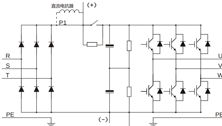
图 3-2 380V (大于 132kW (含)) 主回路简图
