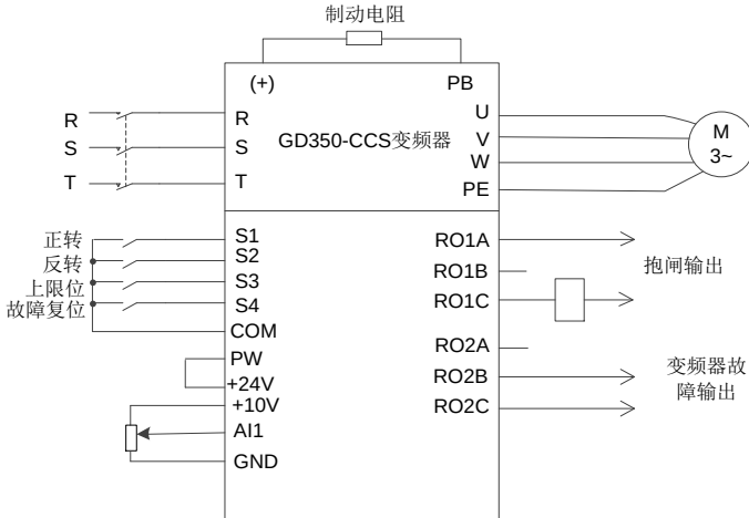
图 5-7 开环矢量卷扬应用接线参考图（推荐模拟量给定选用 0V~10V）
