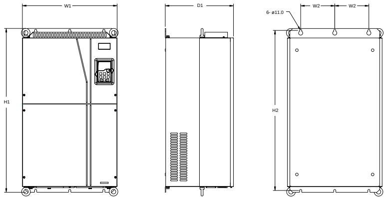
图 C-6 380V 132~200kW 壁挂安装示意图
