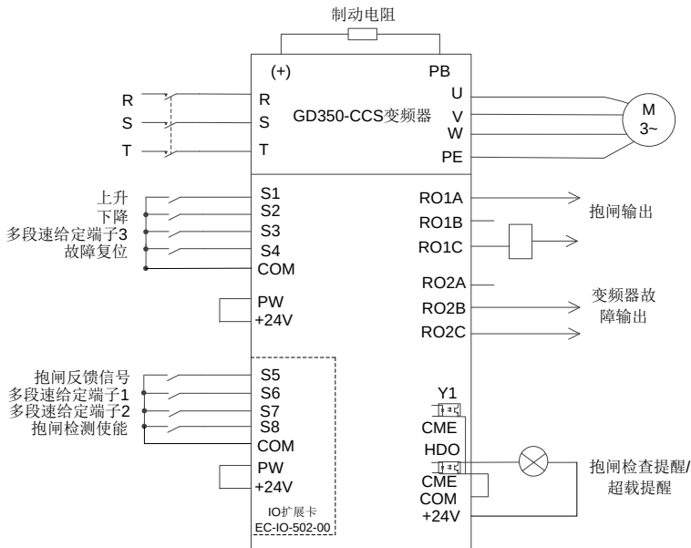
图 5-1 提升开环矢量接线图
