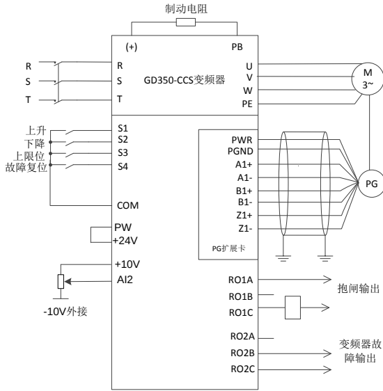
图 5-5 闭环矢量卷扬应用接线参考图（选用模拟量给定选用-10V~10V）
