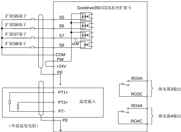
图 4-18 I/O 扩展卡 2 控制回路接线图
