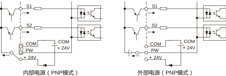
图 4-17 PNP 模式示意图
