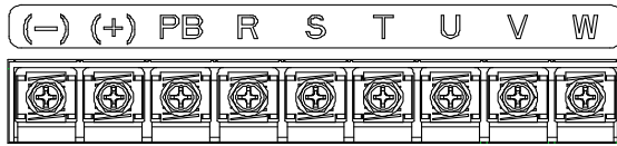
图 4-8 三相 380V 30~37kW 主回路端子示意图
