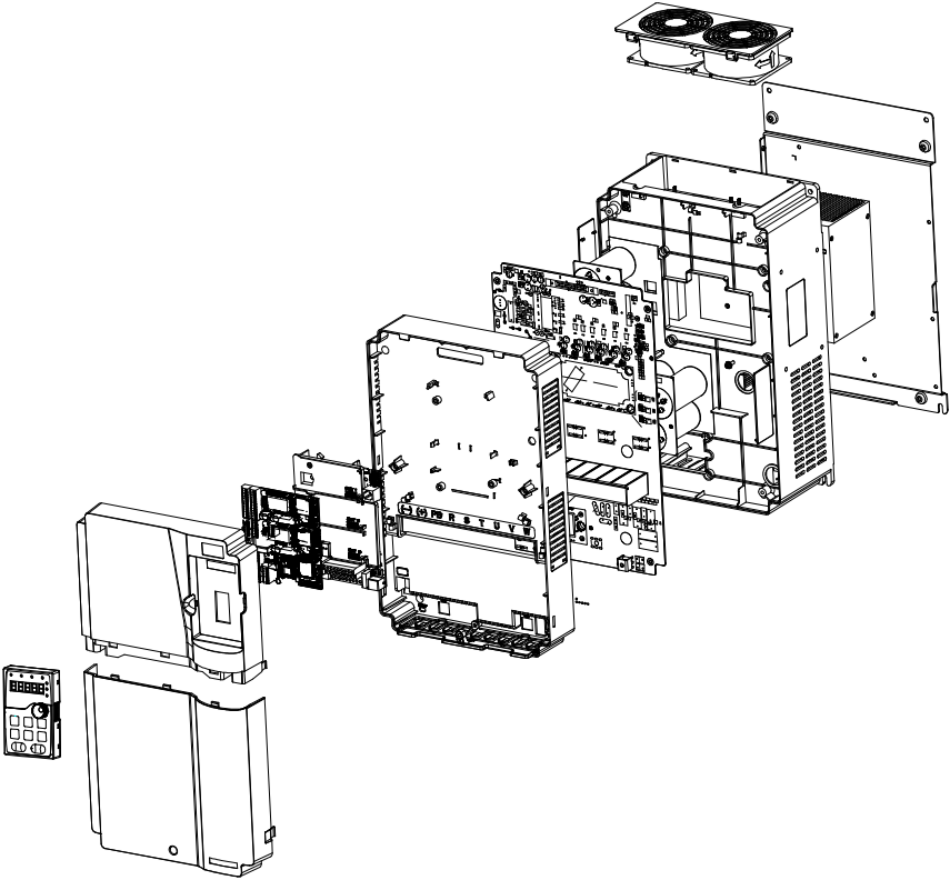
图 C-2 变频器结构图
