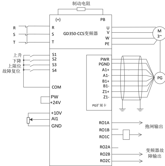
图 5-4 闭环矢量卷扬应用接线参考图（推荐模拟量给定选用 0V~10V）
