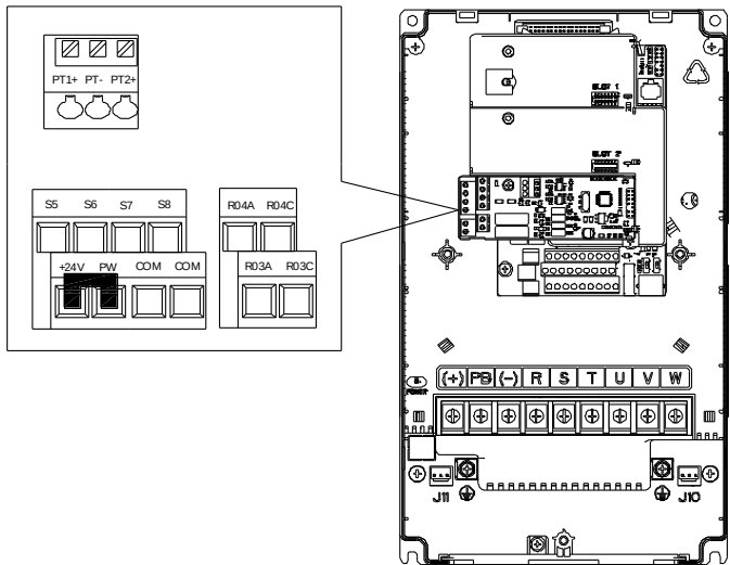
图 4-19 I/O 扩展卡 2 端子排列图
