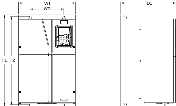
图 C-5 380V 90~110kW 壁挂安装示意图
