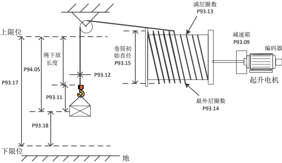
图 5-13 内部测量（电机编码器）：使用滑轮组
