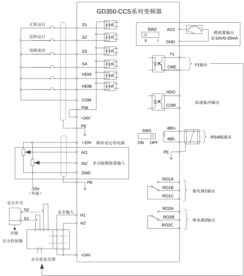
图 4-14 基本控制回路接线图
