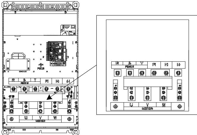
图 4-10 380V 132~200kW 主回路端子示意图
