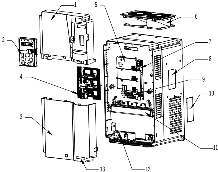
图 3-5 产品结构示意图
