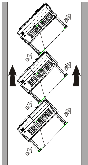
图 4-6 倾斜安装
