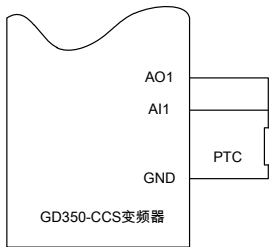
图 5-22 模拟量端口与 PTC 接线图
