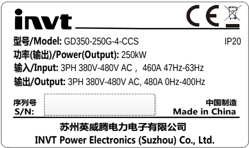
图 3-3 产品铭牌
