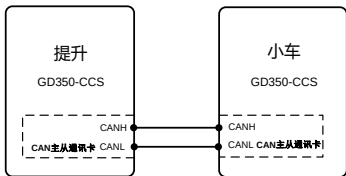
塔吊应用
