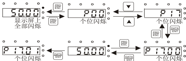
图 6-5 查看参数示意图
