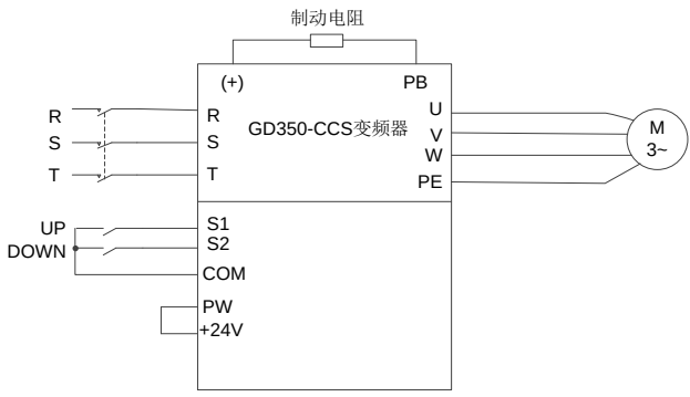
图 5-9 电动电位器调试接线图
