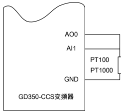
图 5-20 模拟量端口与 PT100/PT1000 接线图
