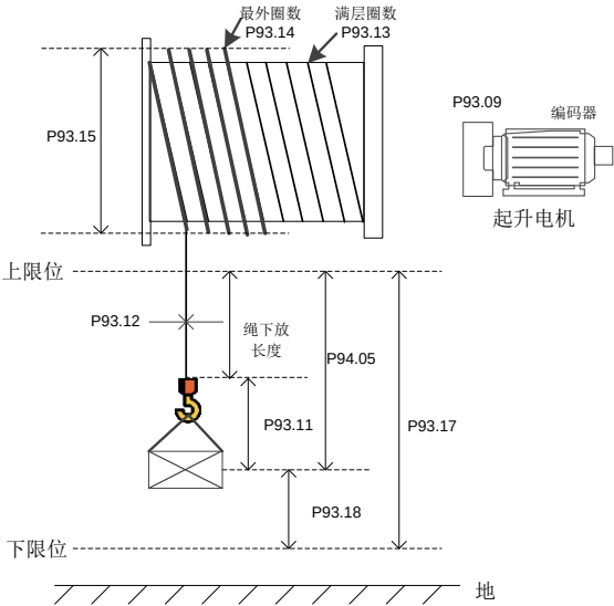
图 5-14 内部测量（电机编码器）：未使用滑轮组
