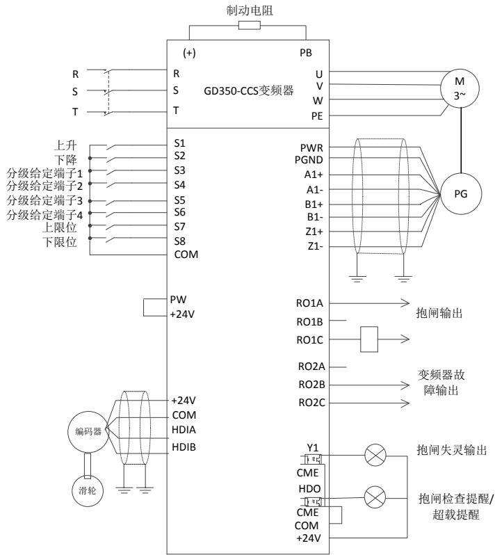
图 5-17 外部测量（HDI）接线图（闭环）
