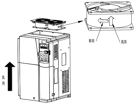
图 10-1 7.5kW（含）以上机器风扇维护示意图
