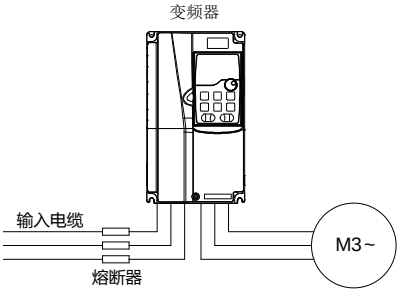
图 4-20 熔断器配置图
