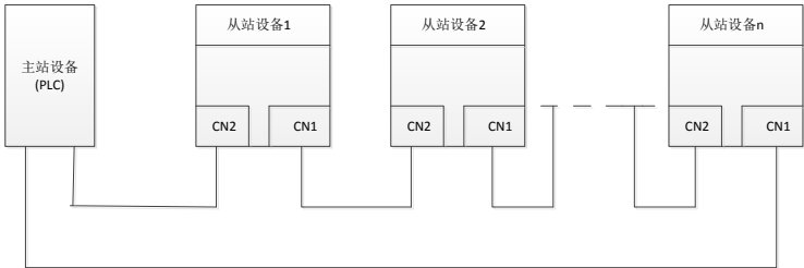
图 A-10 环型网络拓扑电气连接图
