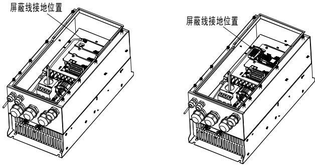
图 A-3 扩展卡地线连接示意图
