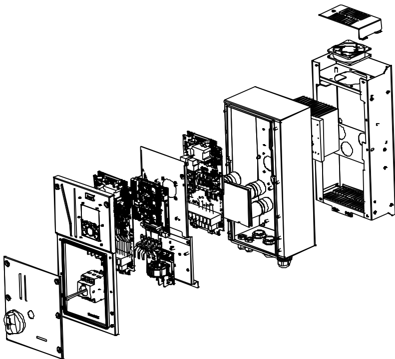
图 C-1 变频器结构图
