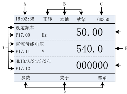
图 5-2 液晶显示器主界面
