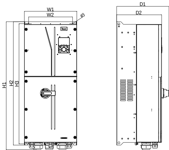
图 C-3 045G/055P~110G 壁挂安装示意图
