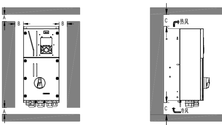
图 4-3 单台安装
