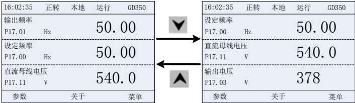
图 5-5 运行参数显示状态图
