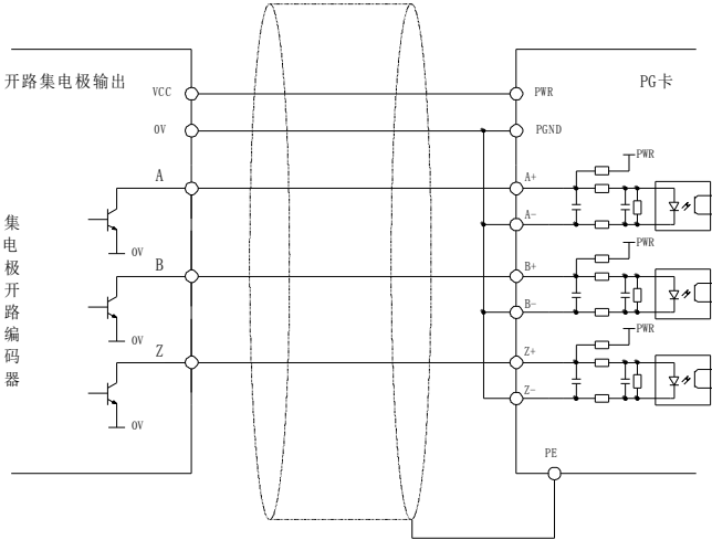
使用屏蔽线
