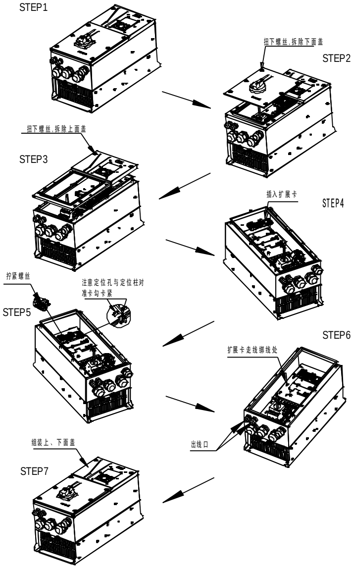
图 A-2 扩展卡安装步骤示意图
