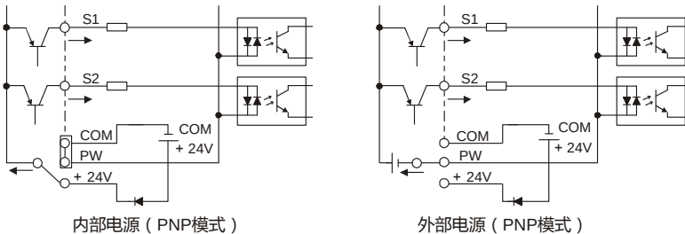
图 4-18 PNP 模式示意图
