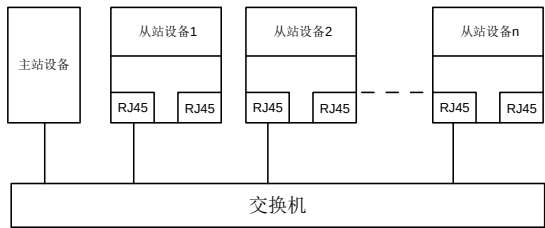
图 A-7 星型网络拓扑电气连接图
