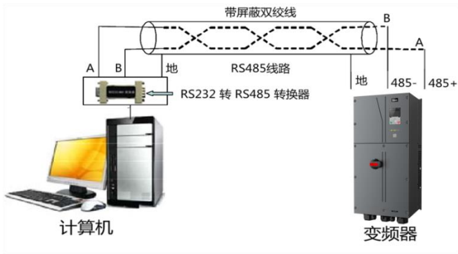
图 10-1 RS485 单机应用时的物理接线图
