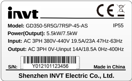
图 3-3 产品铭牌
