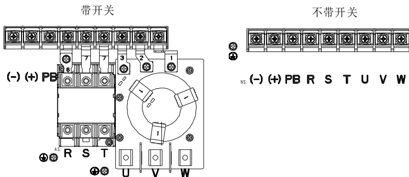
图 4-11 030G/037P~037G/045P 主回路端子示意图
