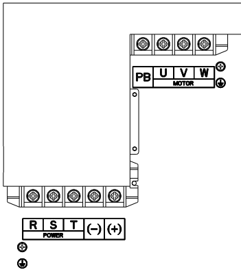
图 4-13 075G/090P~110G 主回路端子示意图
