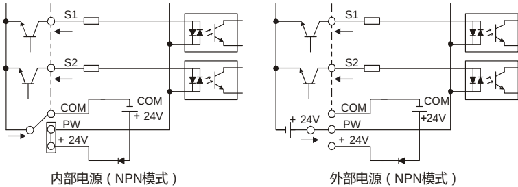
图 4-17 NPN 模式示意图
