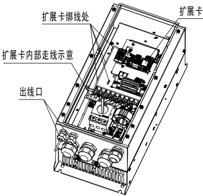
图 A-4 扩展卡走线方式示意图
