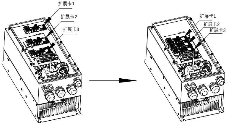
图 A-1 7R5G/011P（含）以上机型效果图
