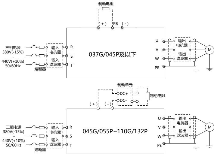
图 4-7 主回路接线图
