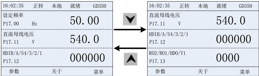
图 5-3 停机参数显示状态图
