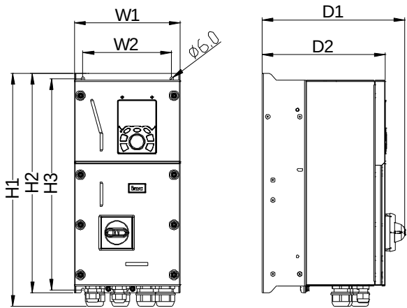
图 C-2 004G/5R5P~037G/045P 壁挂安装示意图
