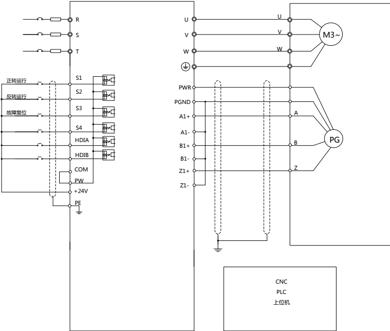
使用屏蔽线
