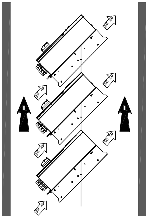
图 4-6 倾斜安装
