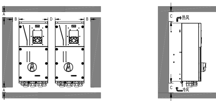
图 4-4 并行安装
