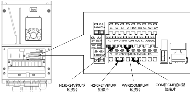
图 4-16 U 型短接位置示意图
