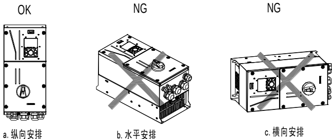
图 4-1 变频器安装方向
