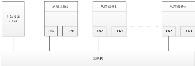
图 A-9 星型网络拓扑电气连接图
