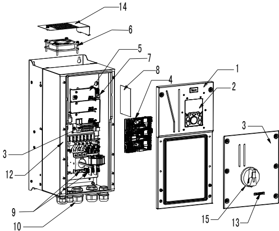
图 3-5 产品结构示意图
