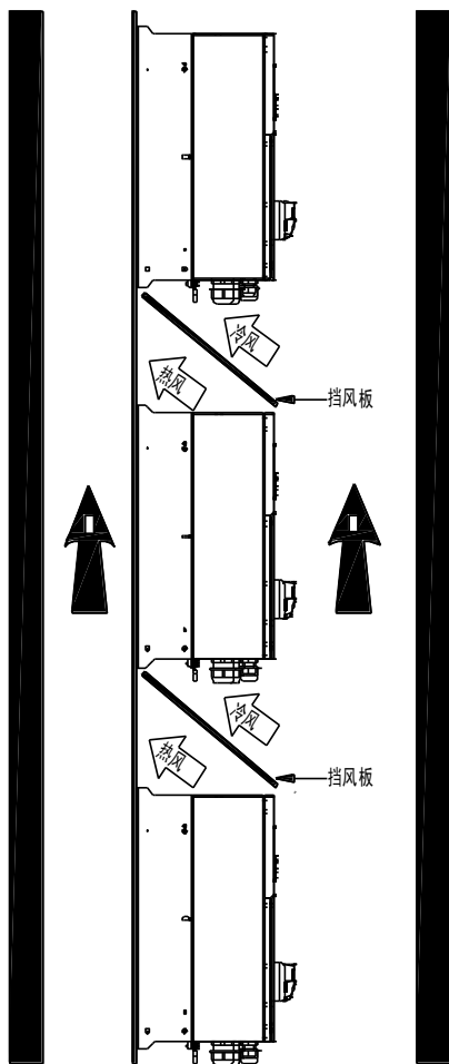
图 4-5 垂直安装
