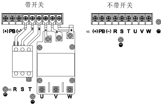
图 4-8 004G/5R5P~5R5G/7R5P 主回路端子示意图
