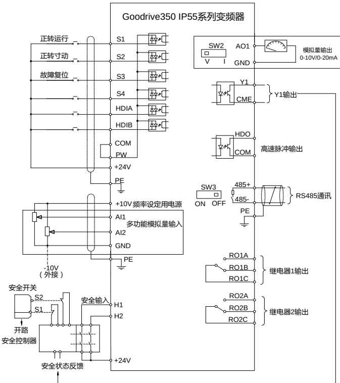
图 4-15 控制回路接线图
