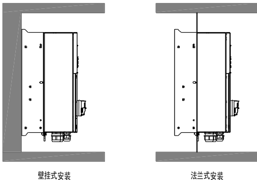
图 4-2 安装方式
