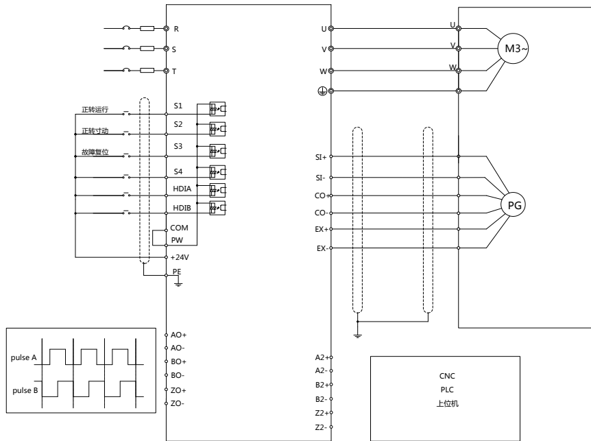
使用 EC-PG504-00 时外部接线图如下所示:
