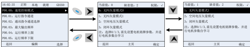
图 5-15 参数选择编辑界面示意图
