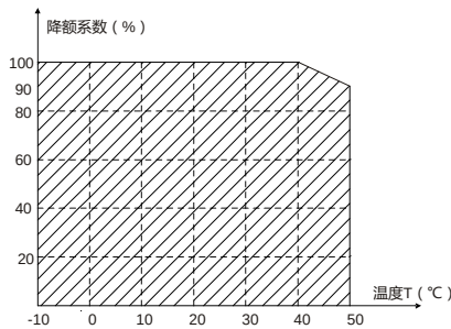
图 B-1 温度实际降额示意图
