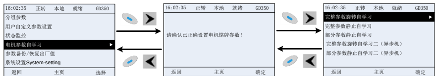
图 5-18 参数自学习操作示意图
