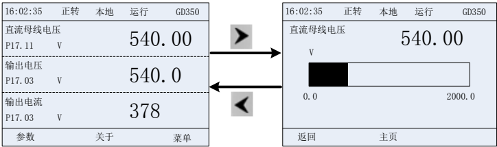
图 5-6 运行参数显示状态图
