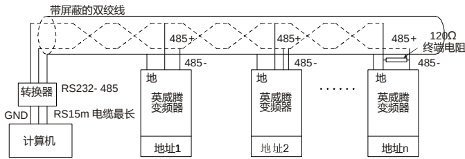
图 10-5 为星形连接方式图，此时在线路距离最远的两个设备上必须连接终端电阻（1# 与 15# 设备）。
