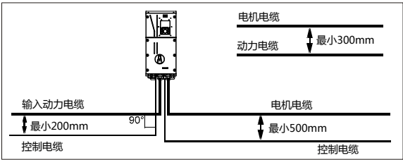
图 D-4 布线距离
