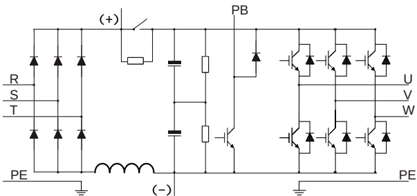
图 3-2 018G/022P~110G（含）主回路简图
