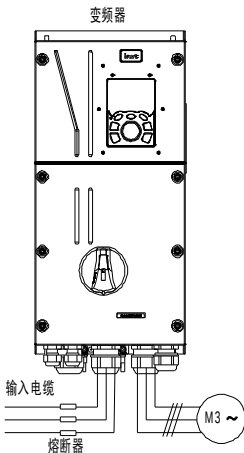
图 4-19 熔断器配置图
