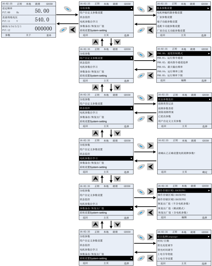
图 5-9 进入/退出各级菜单示意图 2
