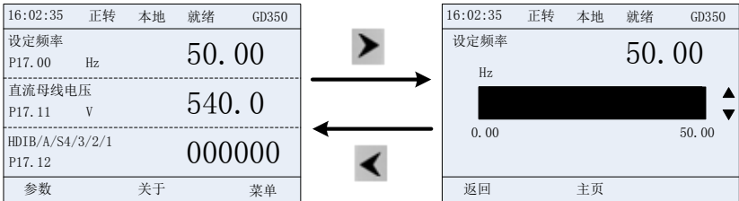
图 5-4 停机参数显示状态图
