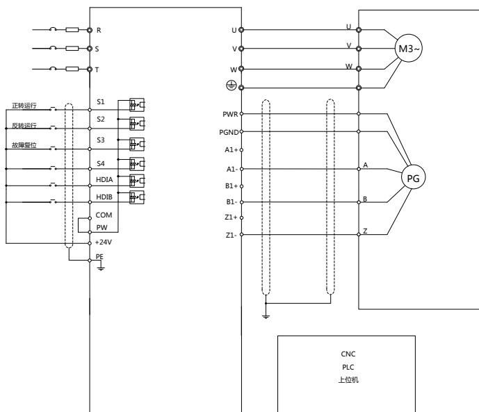
使用屏蔽线
