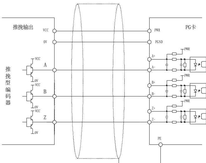
使用屏蔽线
