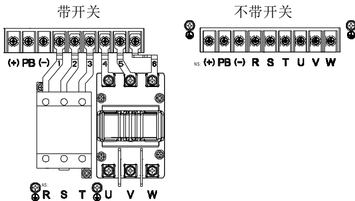
图 4-9 7R5G/011P~015G/018P 主回路端子示意图
