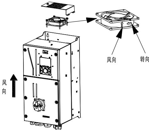
图 9-1 7R5G/011P（含）以上机器风扇维护示意图
