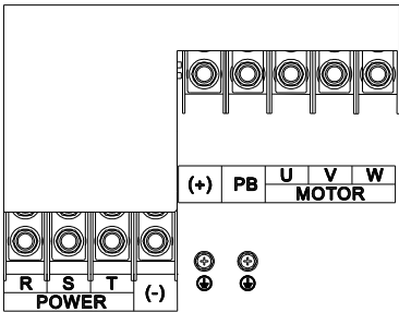
图 4-13 075G/090P~110G 主回路端子示意图
