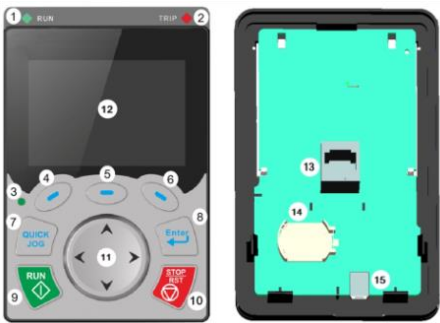
图 5-1 键盘示意图
