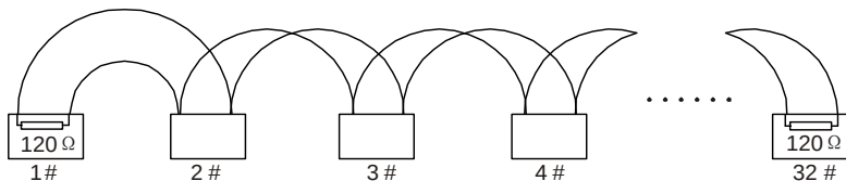
图 10-2 菊花接法现场接线图
