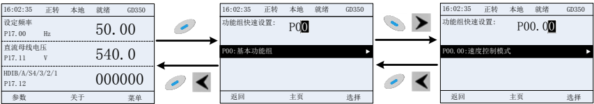
图 5-8 进入/退出各级菜单示意图 1
