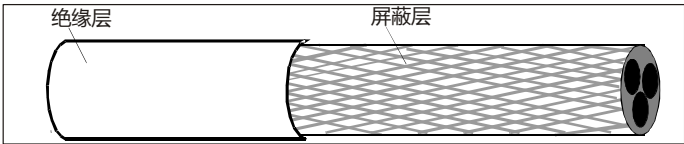
图 D-1 电缆剖面
