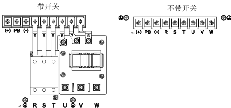
图 4-11 030G/037P~037G/045P 主回路端子示意图
