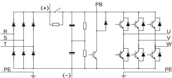
图 3-1 015G/018P（含）以下主回路简图
