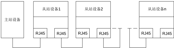
图 A-6 线型网络拓扑电气连接图
