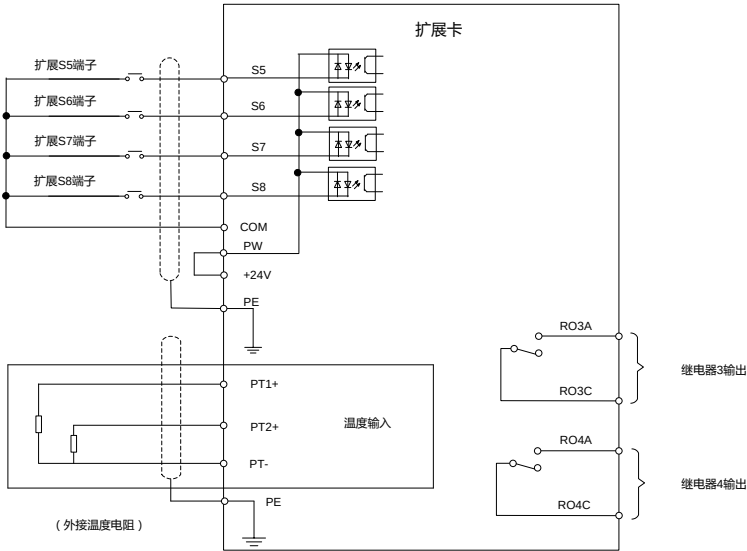
图 A-5 IO 扩展卡 2 控制回路接线图
