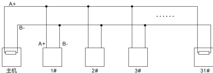
图 10-3 菊花简化接线图
