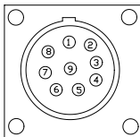
图 2-14 调试航插图
