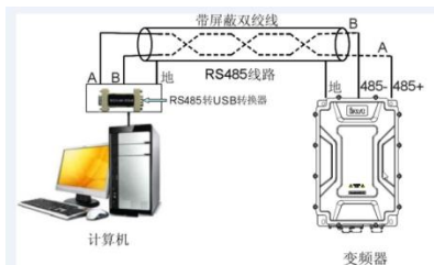
图 2-16 逆变器和上位机接线图
