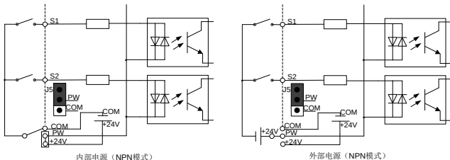
图 2-9 NPN 模式示意图
