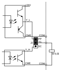
图 2-12 Y 电路推挽输出
