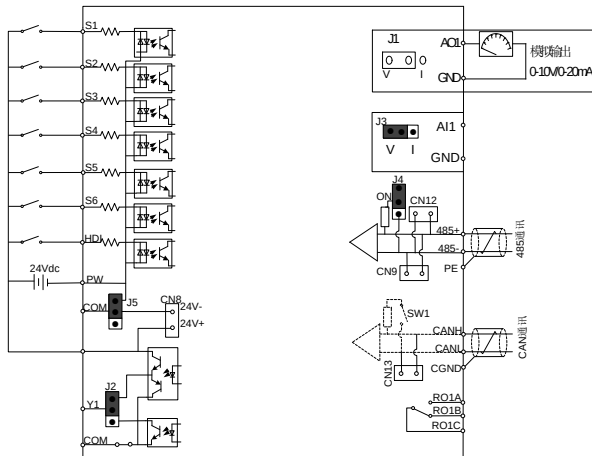
图 2-7 控制回路接线图
