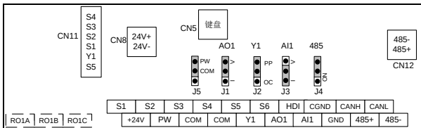
图 2-8 控制端子示意图
