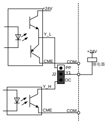
图 2-11 Y 电路集电极开路输出
