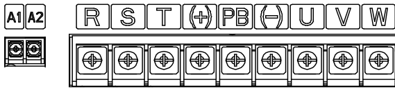
图 4-12 022G/030P~030G/037P 主回路端子示意图
