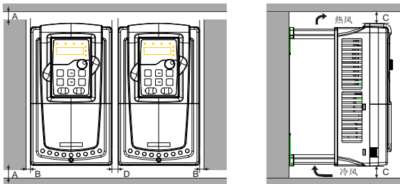
图 4-3 并行安装
