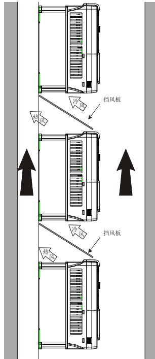
图 4-4 垂直安装
