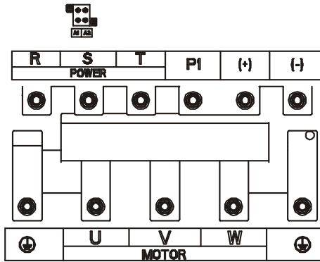
图 4-15 132G/160P~200G/220P 主回路端子示意图
