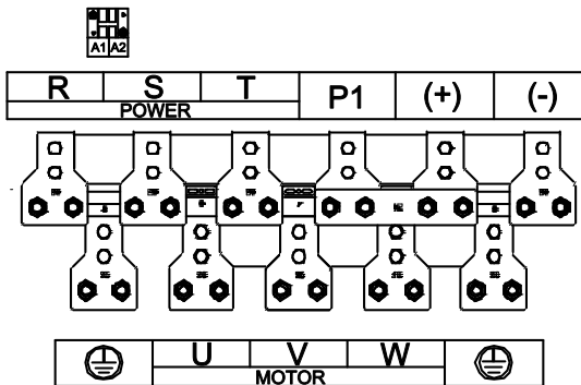
图 4-16 220G/250P~315G/355P 主回路端子示意图
