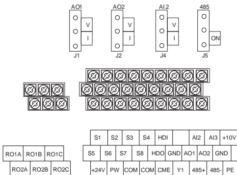
图 4-21 015G/018P 及以下控制端子示意图
