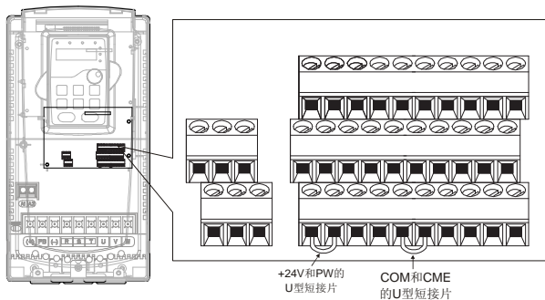
图 4-23 U 型短接位置示意图
