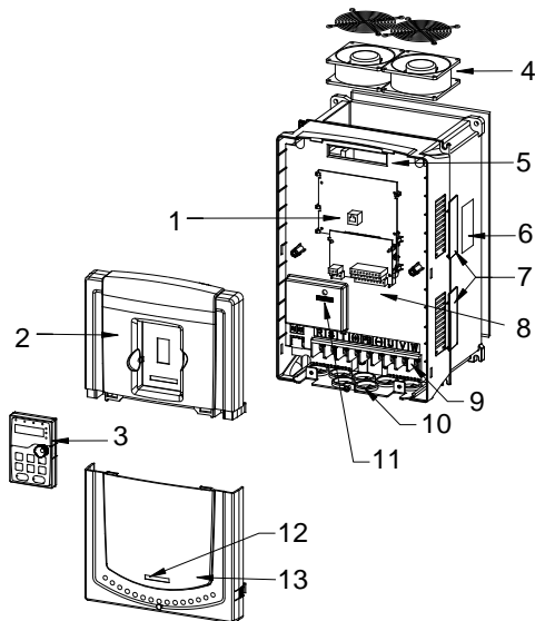
图 3-5 产品结构示意图
