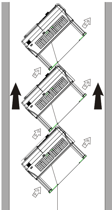
图 4-5 倾斜安装
