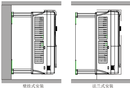
图 4-2 安装方式
