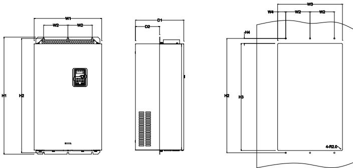
图 B-11 132G/160P~200G/220P 法兰安装示意图
