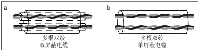
图 C-3 动力电缆布线
