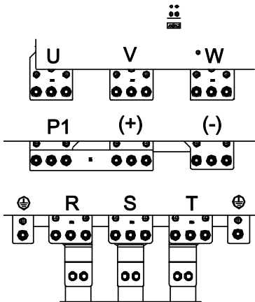
图 4-17 355G/400P~500G 主回路端子示意图
