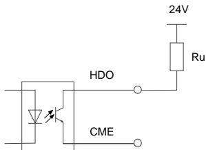
图 4-20 HDO 接线示意图
