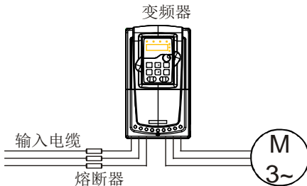
图 4-26 熔断器配置图
