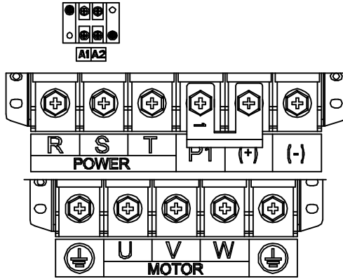
图 4-14 075G/090P~110G/132P 主回路端子示意图
