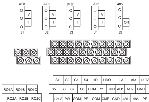
图 4-21 015G/018P 及以下控制端子示意图
