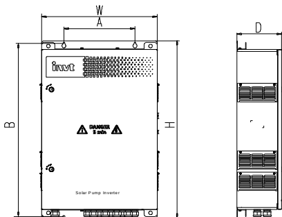
图 C-3 IP54 变频器尺寸图
