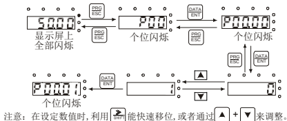
图 4-4 修改参数示意图
