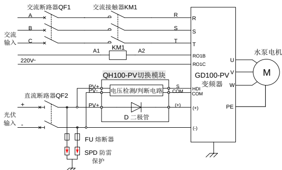
图 C-1 变频器交/直流输入切换方案
