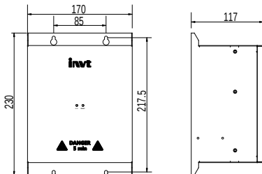
图 A-2 升压模块安装尺寸图
