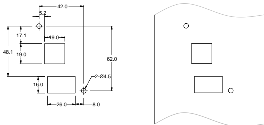
图 B-2 键盘无支架开孔示意图
