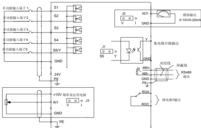
图 3-5 控制回路接线图
