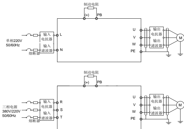
图 3-3 主回路接线图
