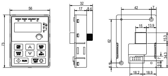
图 B-1 键盘外形图
