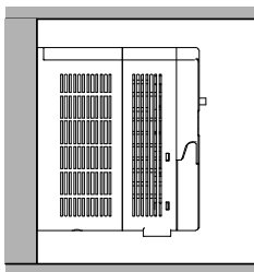
图 3-1 壁挂式安装
