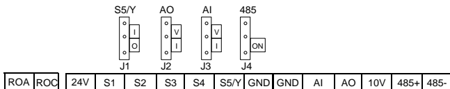
图 3-6 控制端子示意图
