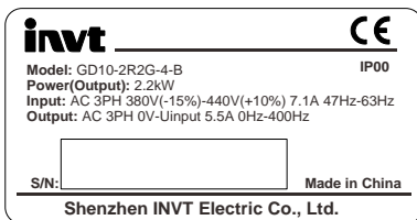
图 2-1 产品铭牌
