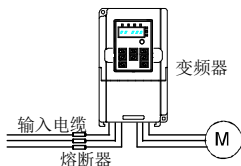
图 3-7 熔断器配置图
