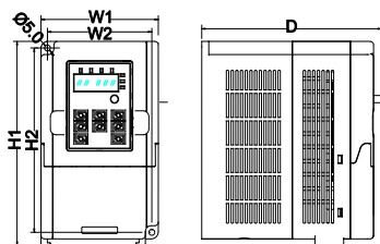
图 B-3 壁挂安装
