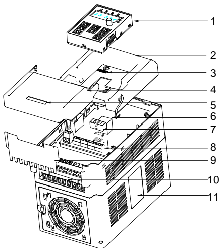
图 2-3 产品结构示意图
