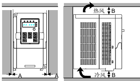
图 3-2 安装间距
