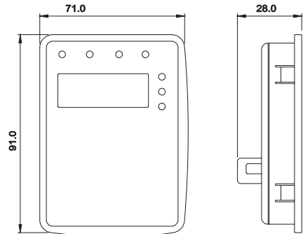
图 A-9 外引键盘（小）的安装尺寸
