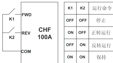
图 6-9 两线式控制（使能与方向合一）
