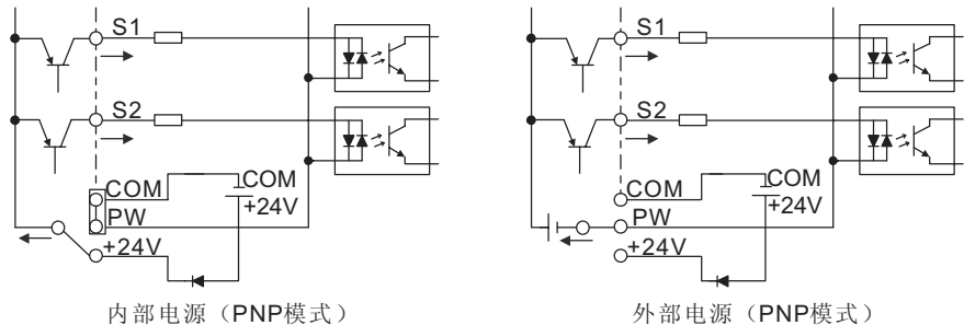
图 4-18 共集电极模式
