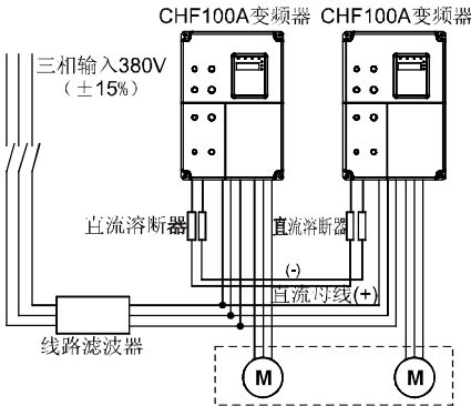
图 4-22 共直流母线的连接
