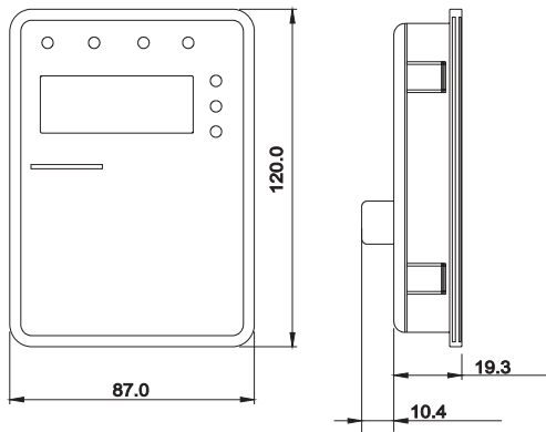
图 A-11 外引键盘（大）的安装尺寸
