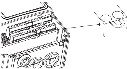
图 4-16 U 型短接片
