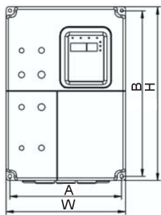
图 A-4 7.5kW 及以下机型的外形尺寸（230V）
