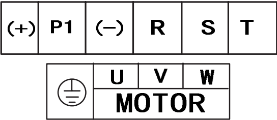
图 4-11 主回路接线端子图（22kW 以上，为上进下出结构）
