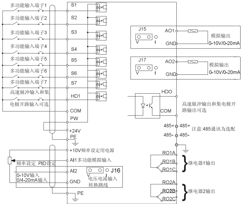
图 4-15 控制回路接线图
