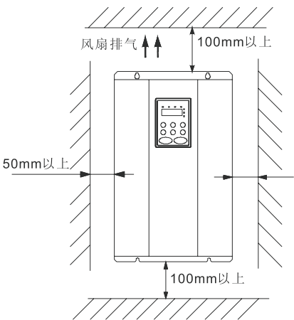
图 A-7 安装的间隔距离
