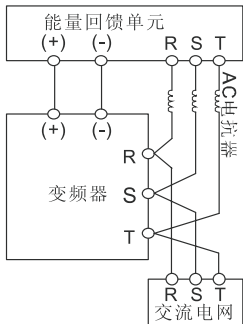
图 4-21 能量回馈单元连接图
