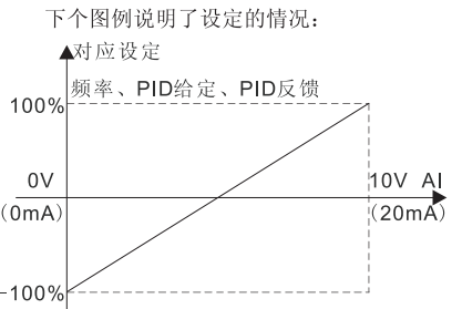
图 6-13 模拟给定与设定量的对应关系
