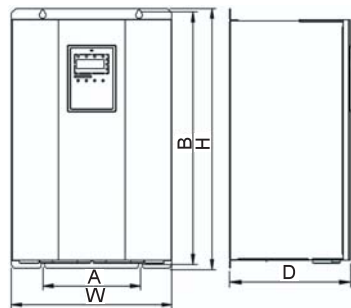
图 A-5 11kW~18.5kW 机型外形尺（230V）
