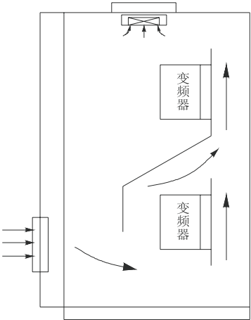
图 A-8 多台变频器的安装
