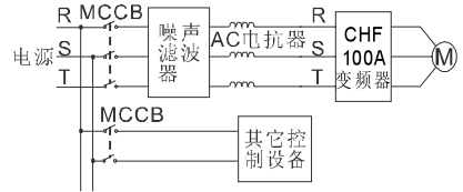
图 4-17 主回路电源侧连接图
