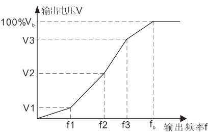
图6-8 V/F曲线设定示意图
