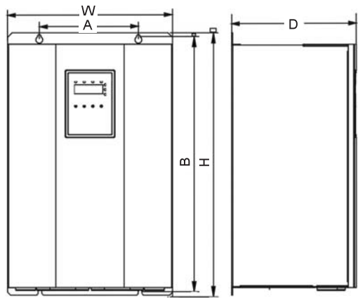
图 A-2 18.5~110kW 机型外形尺寸（400V）
