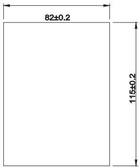
图 A-12 外引键盘（大）的开孔尺寸
