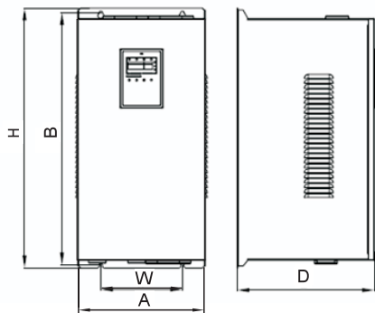
图 A-6 22~55kW 机型的外形尺寸（230V）
