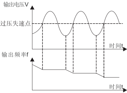
图 6-28 过压失速功能
