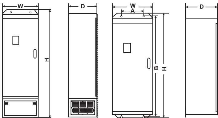
图 A-3 132~500kW 机型（有底座和无底座）外形尺寸（400V）
