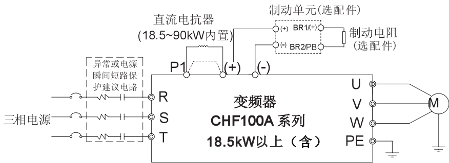
图 4-14 18.5kW以上（含）主回路接线图
