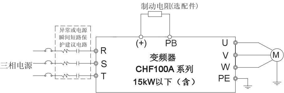
图 4-13 15kW以下（含）主回路接线图
