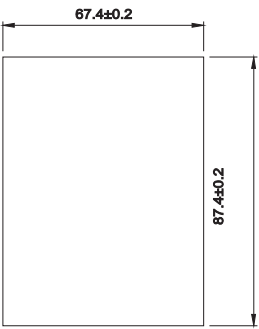
图 A-10 外引键盘（小）的开孔尺寸
