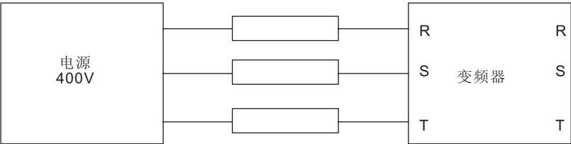
图 8-1 400V 驱动装置充电电路示例
