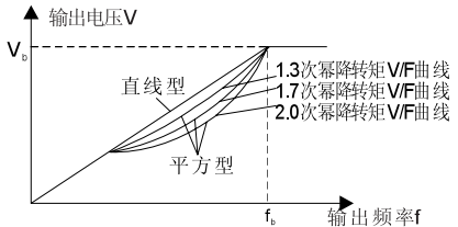
图6-6 V/F 曲线示意图
