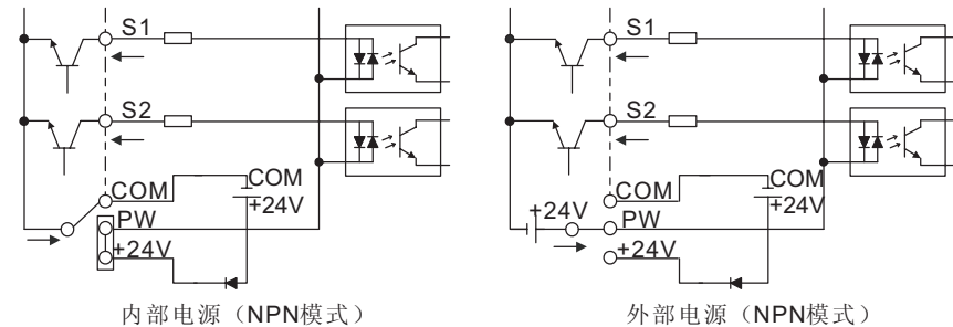
图 4-17 共发射极模式
