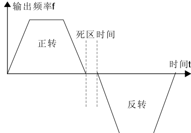
图6-4 正反转死区时间示意图
