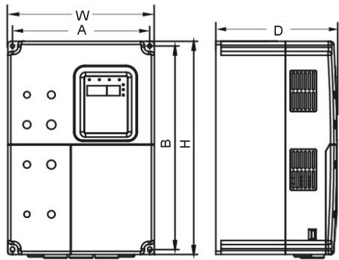
图 A-1 15kW 及以下机型的外形尺寸（400V）
