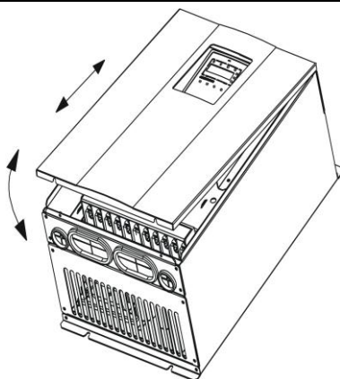
图 A-16 钣金盖板的拆卸和安装示意图
