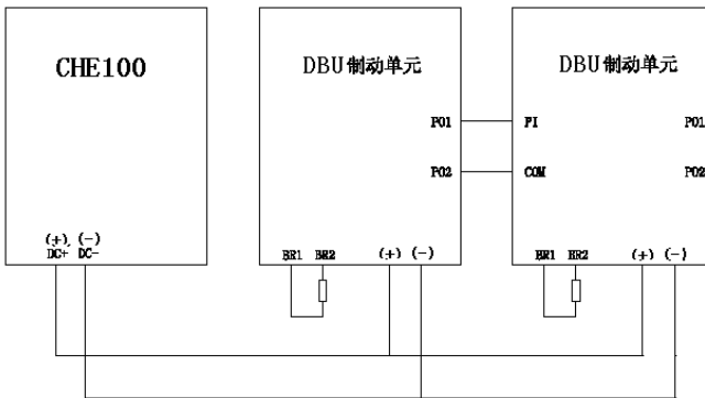
图 B-3 制动单元的并联连接
