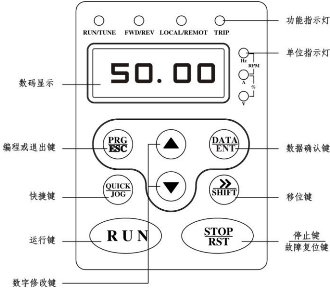
图 5-1 键盘示意图
