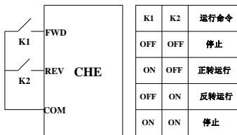
图 6-8 两线式控制 1 (使能与方向合一)
