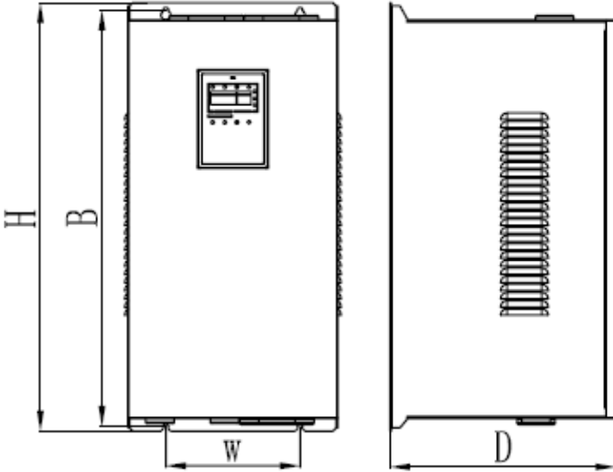
图 A-8 22~55kW 机型的外形尺寸
