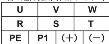
图 4-7 主回路接线端子图(350~500kW)
