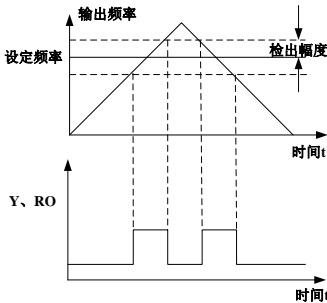
图6-17 频率到达检出幅值示意图
