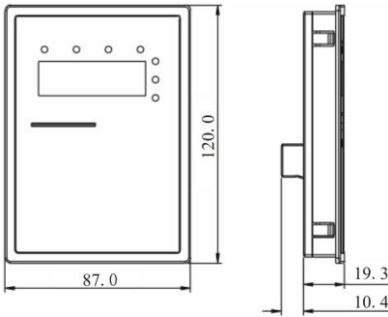
图 A-11 外引键盘（大）的安装尺寸
