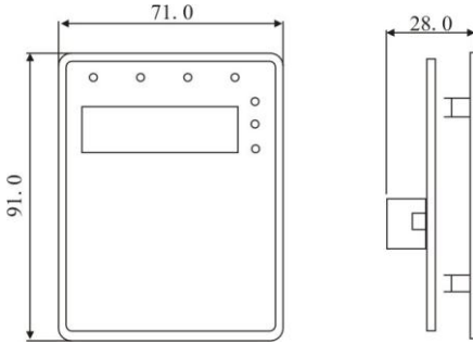
图 A-9 外引键盘（小）的安装尺寸
