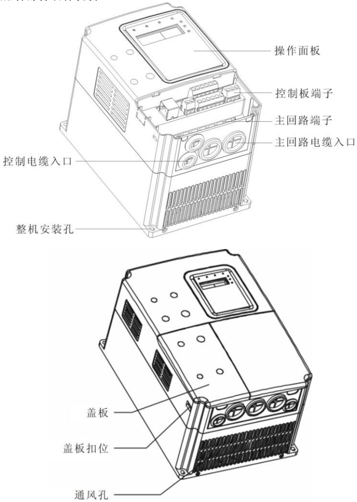
图 1-2 15kW 及以下变频器各部件名称
