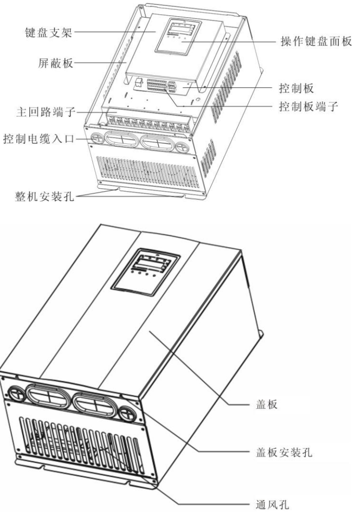
图 1-3 18.5kW~110kW 变频器各部件名称
