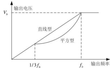
图6-6 V/F曲线示意图
