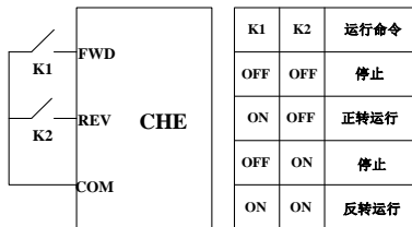
图 6-9 两线式控制 2 (使能与方向分离)
