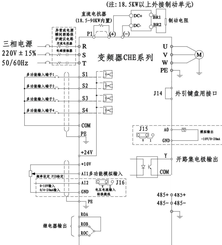
图 4-17 标准接线图
