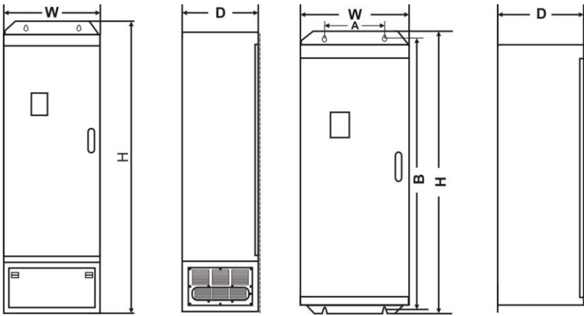
图 A-3 132kW~500kW 机型(无底座)外形尺寸
