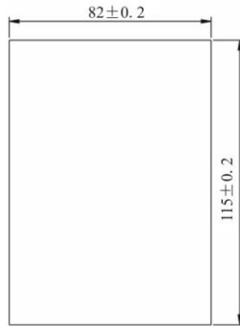
图 A-12 外引键盘（大）的开孔尺寸
