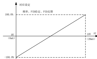
图 6-12 模拟给定与设定量的对应关系
