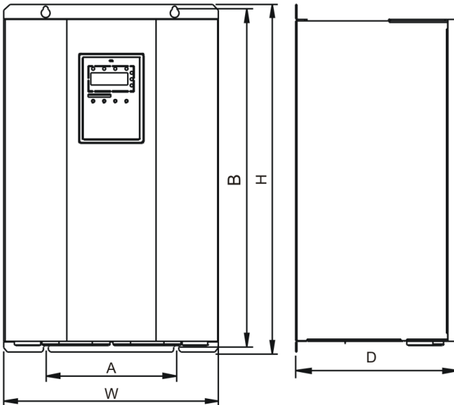
图 A-7 11kW~18.5kW 机型外形尺寸
