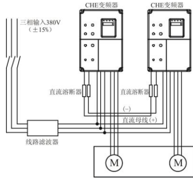
图 4-21 共直流母线的连接
