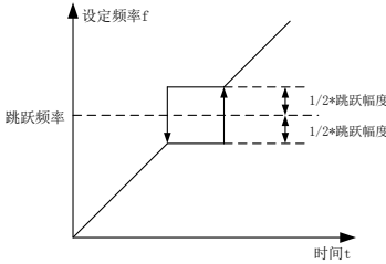
图6-14 跳跃频率示意图
