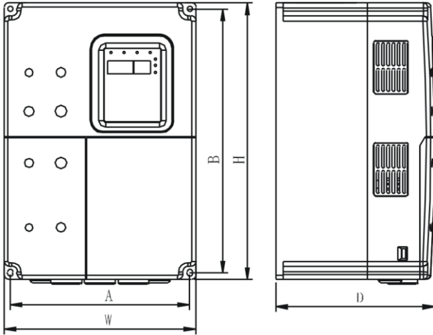
图 A-6 7.5kW 及以下机型的外形尺寸
