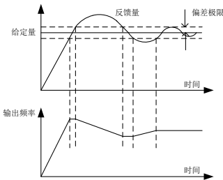
图6-19 偏差极限与输出频率的对应关系
