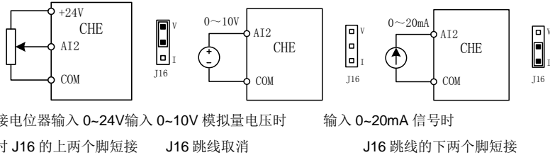
图 4-22 单相 0.4~0.75kW 控制端子连线说明图
