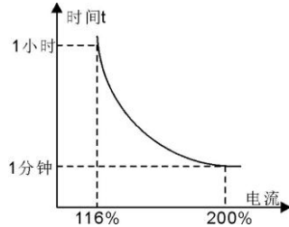
图6-21 电机过载保护系数设定
