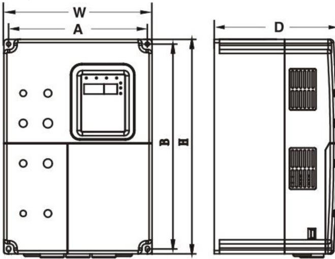
图 A-1 15kW 及以下机型的外形尺寸
