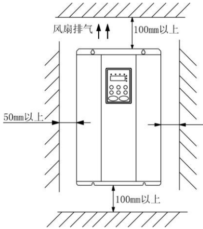
图 A-13 安装的间隔距离
