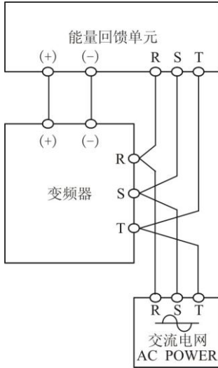
图 4-20 能量回馈单元连接图
