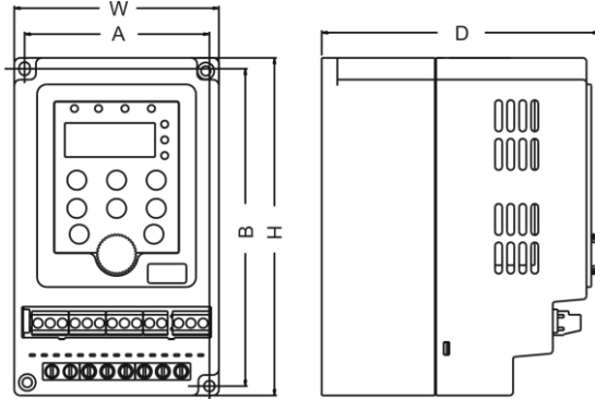
图 A-4 0.4~0.75kW 标准外形尺寸
