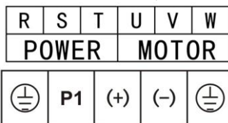
图 4-6 主回路接线端子图(132~315kW)
