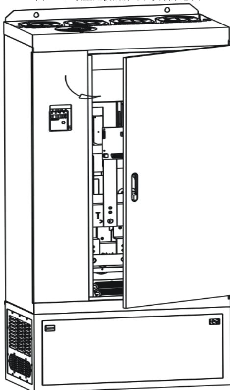
图 A-17 柜式结构的拆卸和安装示意图
