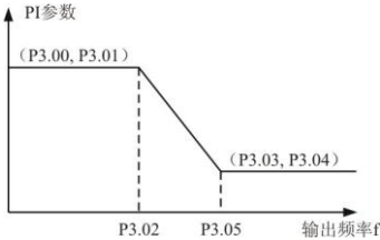
图 6-5 PI 参数示意图
