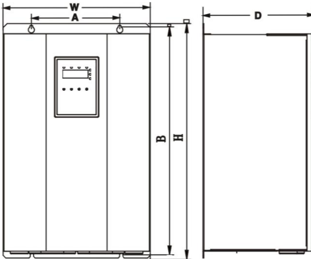
图 A-2 18.5kW~110kW 机型外形尺寸
