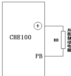
图 B-1 制动电阻的安装
