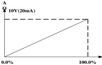
图6-13 给定量与模拟输出对应关系
