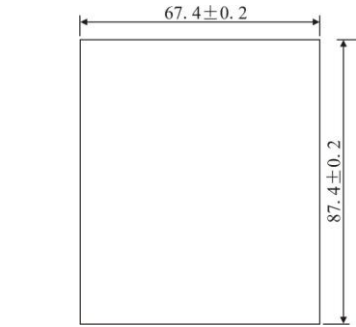
图 A-10 外引键盘（小）的开孔尺寸
