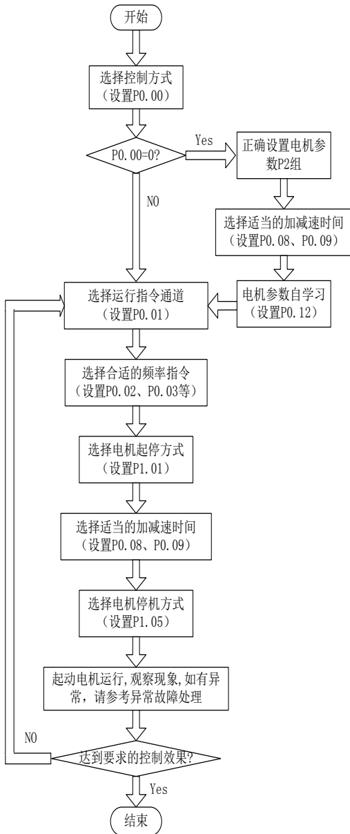
图 5-6 快速调试流程图
