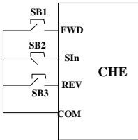
图 6-11 三线式控制模式 2
