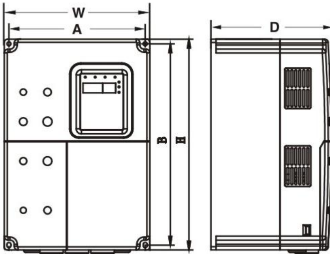
图 A-5 15kW 及以下机型的外形尺寸
