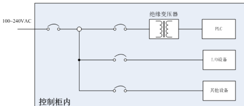
图 5-1 绝缘变压器工作示意图
