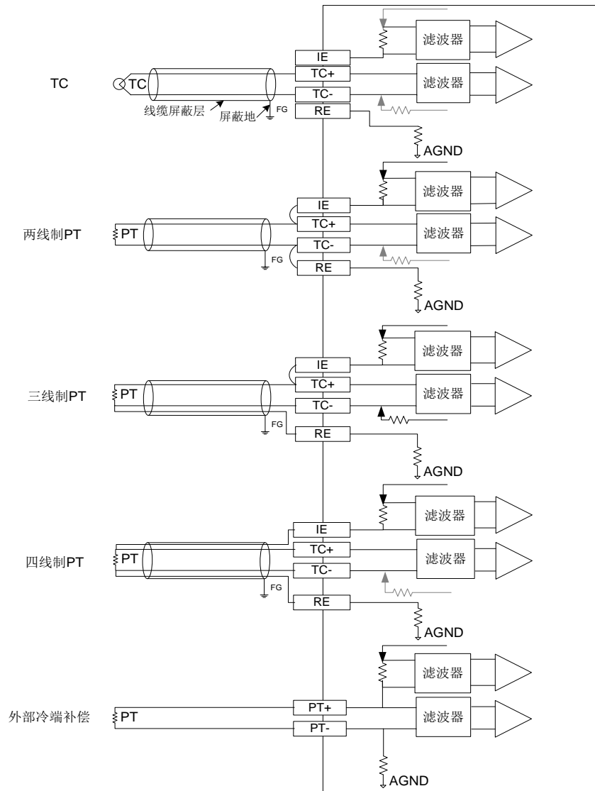
图 5-22 布线示意图
