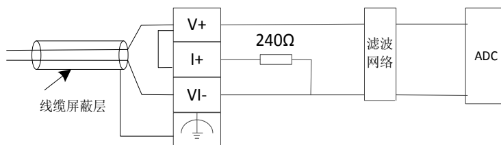
图 5-20 电流输入布线图
