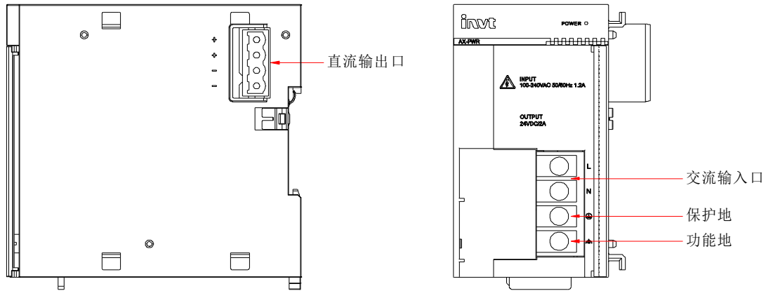
图 5-2 电源模块接口示意图
