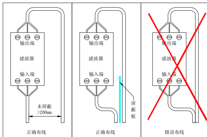
图 5-3 电源滤波器的安装示意图
