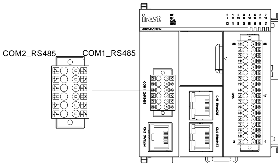
图 5-10 COM1/CN2 接口示意图
