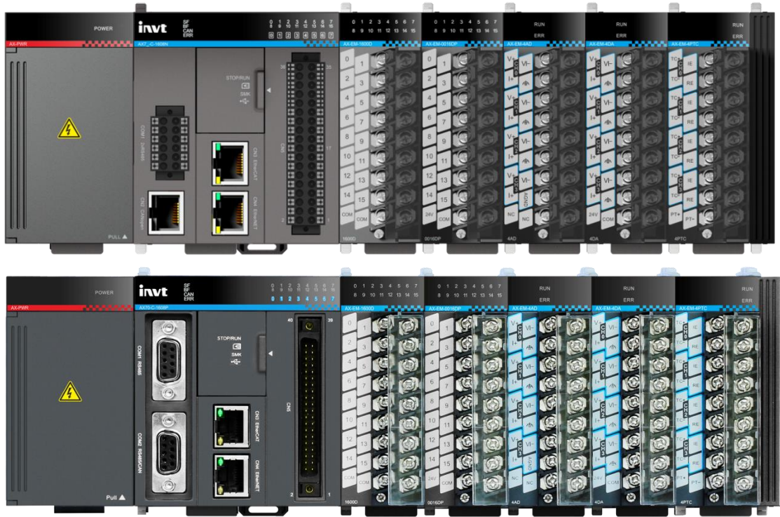
图 2-4 AX7□系列可编程控制器组合示意图
