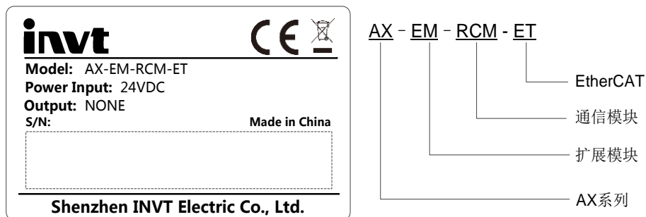
图 2-12 AX-EM-RCM-ET 远程扩展通信模块
