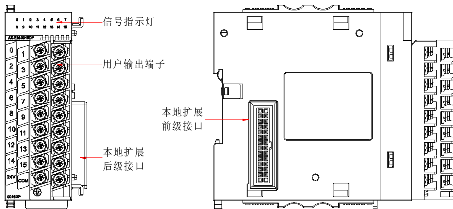
图 3-6 数字量输出模块接口示意图
