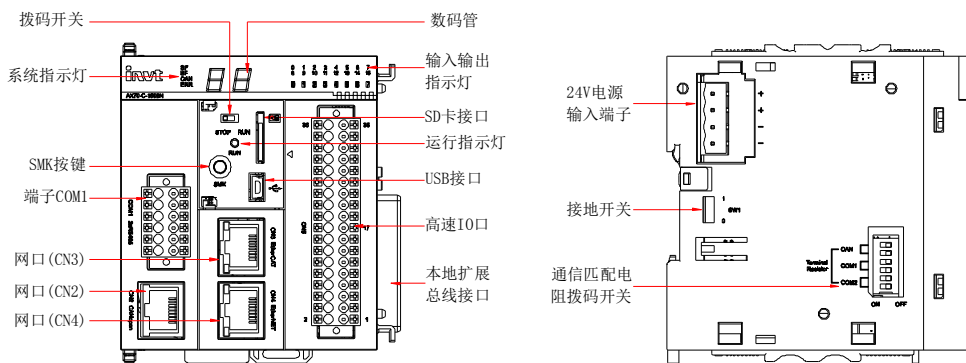
图 3-2 AX7□-C-1608N CPU 模块接口示意图
