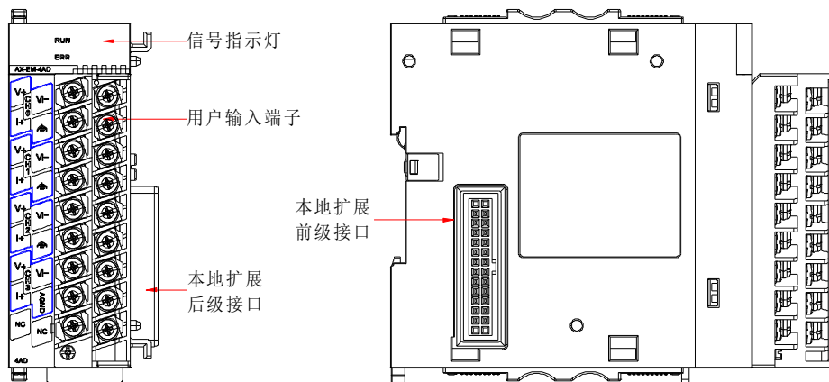
图 3-7 模拟量输入模块接口示意图
