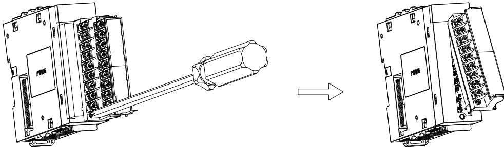
图 4-3 端子排拆卸示意图
