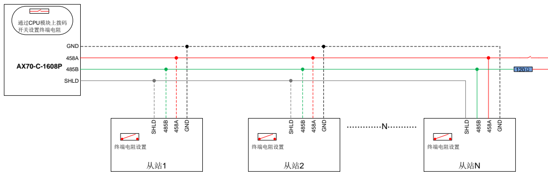
图 5-11 RS485 总线连接拓扑结构
