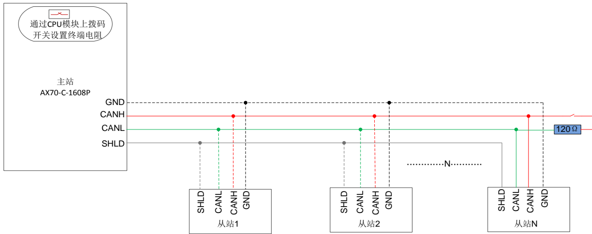
图 5-12 CAN 总线连接示意图
