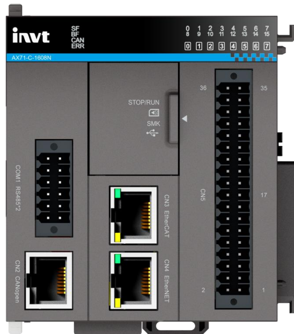
图 2-3 AX7□-C-1608N CPU 模块示意图
