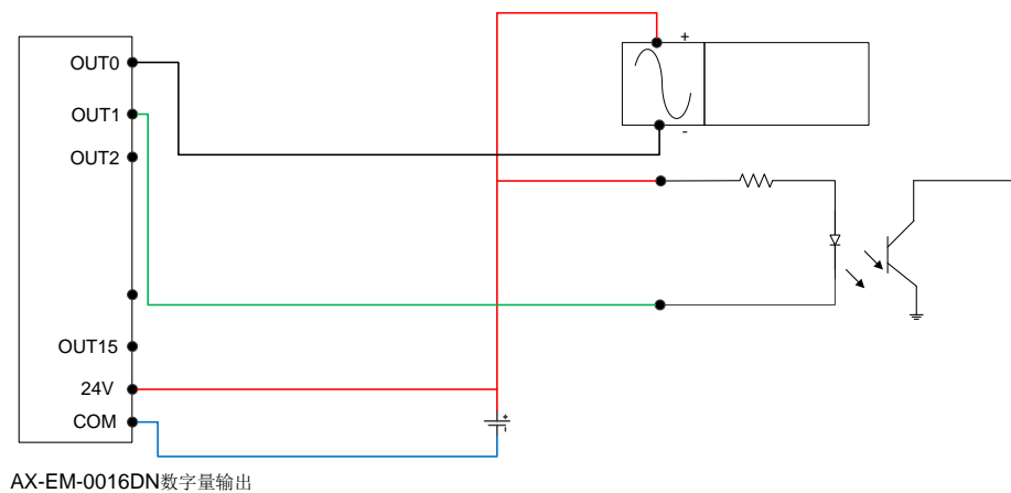
AX-EM-0016DN数字量输出
