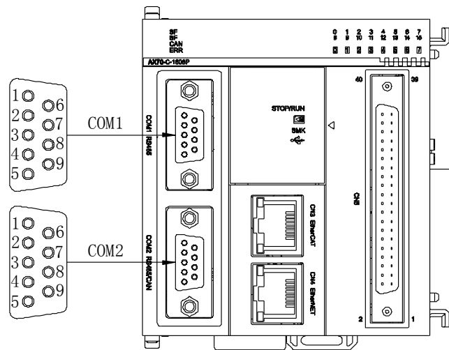
图 5-9 DB9 接口分布示意图
