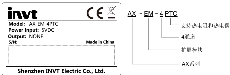
图 2-11 AX-EM-4PTC 温度测量模块
