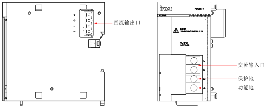
图 3-3 电源模块接口示意图
