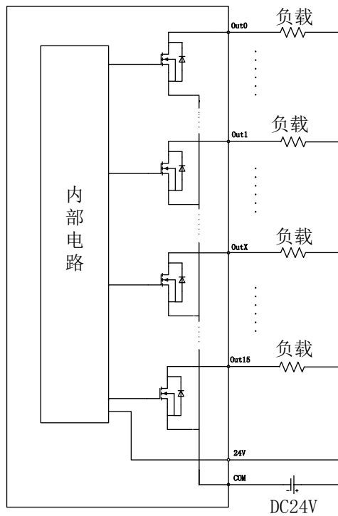
图 5-18 用户端子布线示意图
