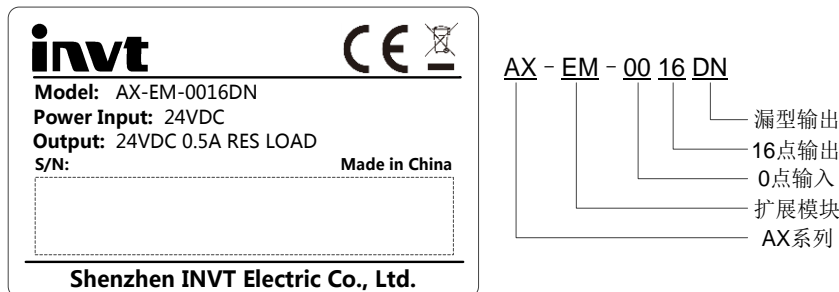
图 2-8 AX-EM-0016DN 数字量输出模块（漏型）
