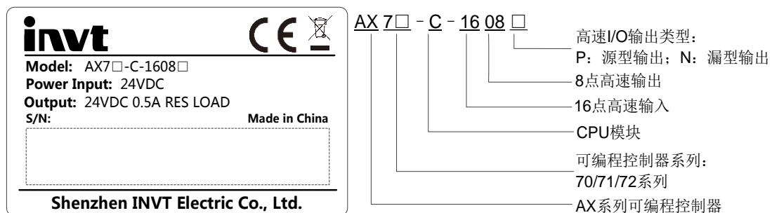
图 2-5 AX7□系列 CPU 模块
