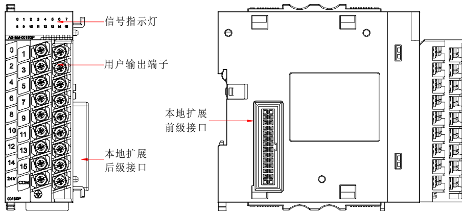
图 3-5 数字量输出模块接口示意图
