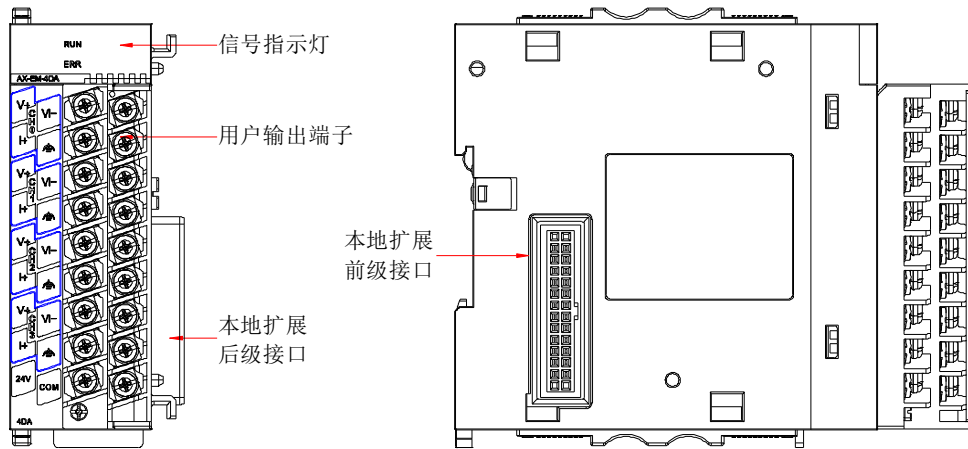
图 3-8 模拟量输出模块接口示意图
