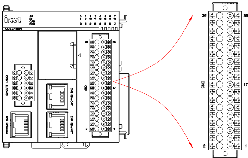
图 5-7 CPU 高速 I/O 接线端子图
