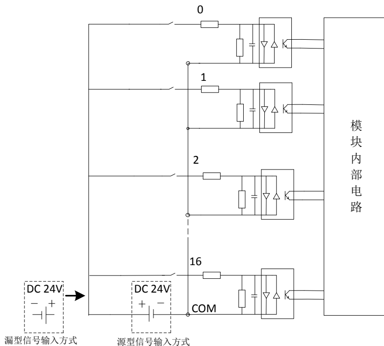
图 5-16 AX-EM-1600D 用户端子布线示意图
