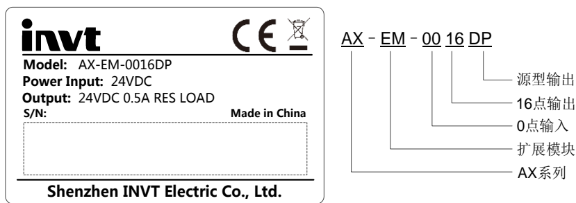
图 2-7 AX-EM-0016DP 数字量输出模块（源型）
