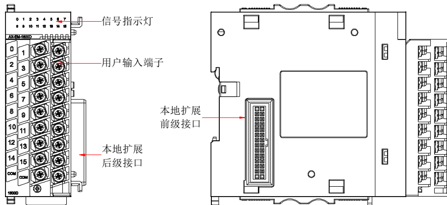
图 3-4 数字量输入模块接口示意图
