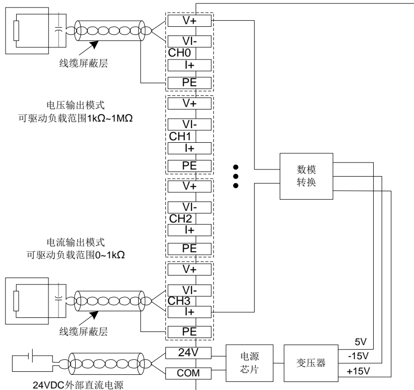
图 5-21 用户端子布线示意图
