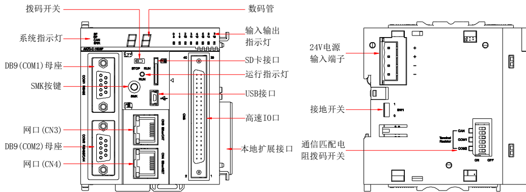
图 3-1 AX7□-C-1608P CPU 模块接口示意图
