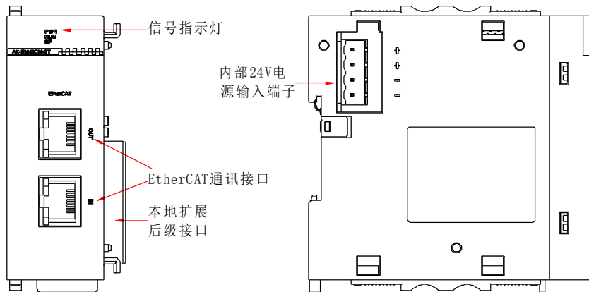
图 3-10 EtherCAT 远程扩展通信模块接口示意图
