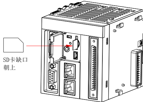
图 4-5 SD 存储卡安装示意图
