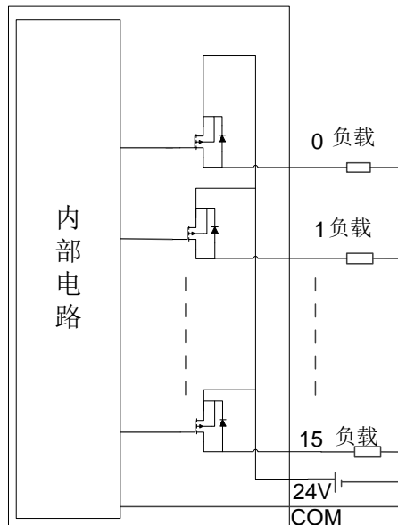
图 5-17 用户端子布线示意图
