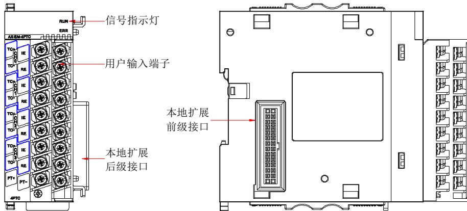
图 3-9 温度测量模块接口示意图
