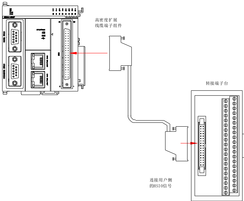
图 5-6 转接示意图
