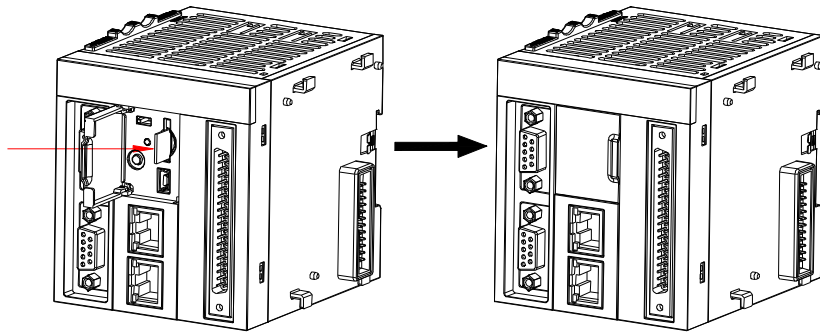
图 4-6 SD 存储卡拆卸示意图
