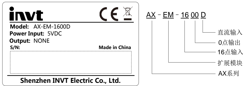
图 2-6 AX-EM-1600D 数字量输入模块
