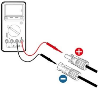
图 5.3 测量直流输入电压
