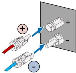
图 5.4 光伏直流组串接入逆变器
