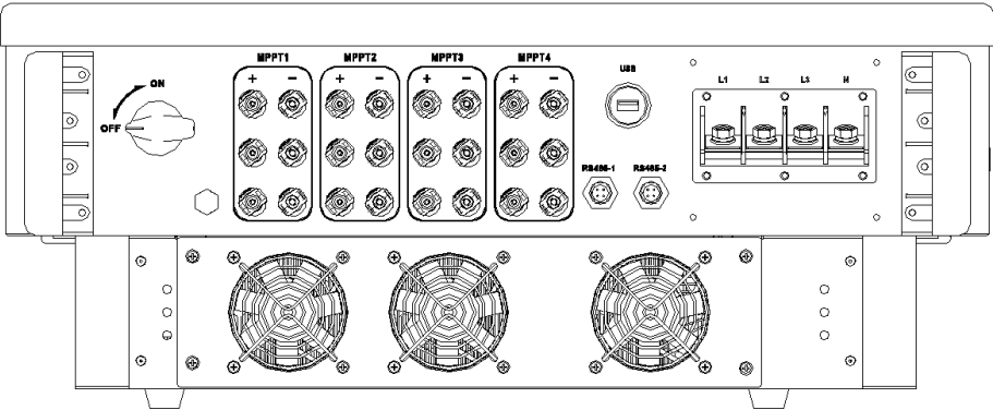
XG50KTR 底部视图
