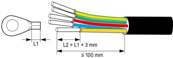
图 5.6 压接电缆端子
