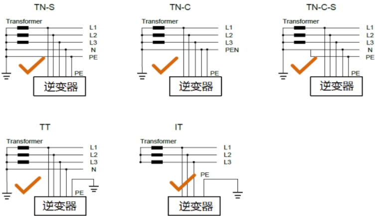
图 2.2 光伏并网逆变器支持的电网形式
