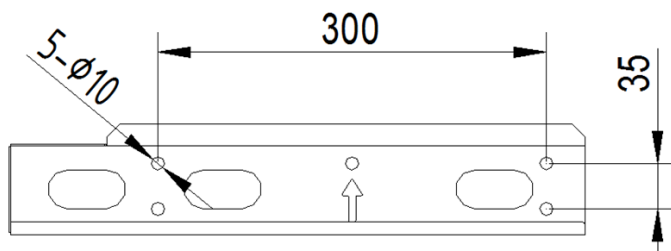
图 4.6 安装挂板尺寸图
