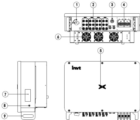
图 2.3 三相光伏逆变器外观图
