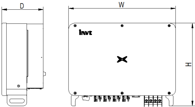
图 2.5 逆变器外形尺寸
