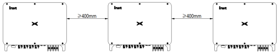
图 4.5 并排安装尺寸要求
