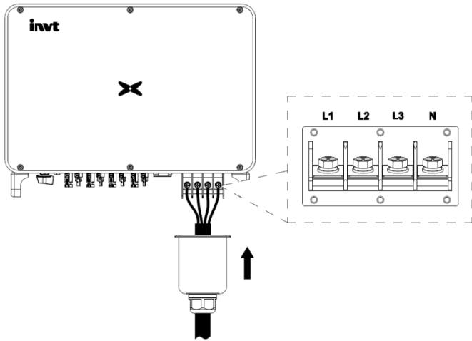
图 5.7 三相逆变器电网接入
