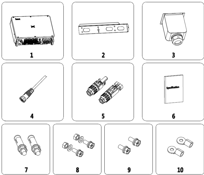
图 4.1 三相逆变器 50-70kW 交付内容
