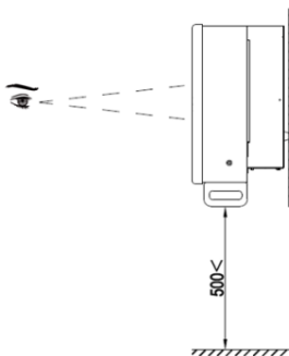
图 4.3 最佳安装高度区域
