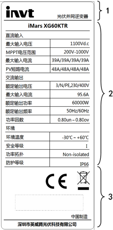
图 2.4 铭牌模板
