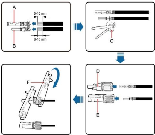
图 5.2 MC4 直流连接器与光伏组串的连接
