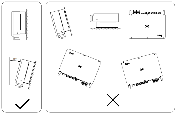
图 4.5 逆变器安装位置
