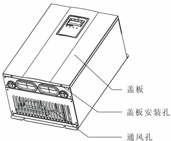
图 1-3 18.5kW 及以上金属外壳变频器各部件名称
