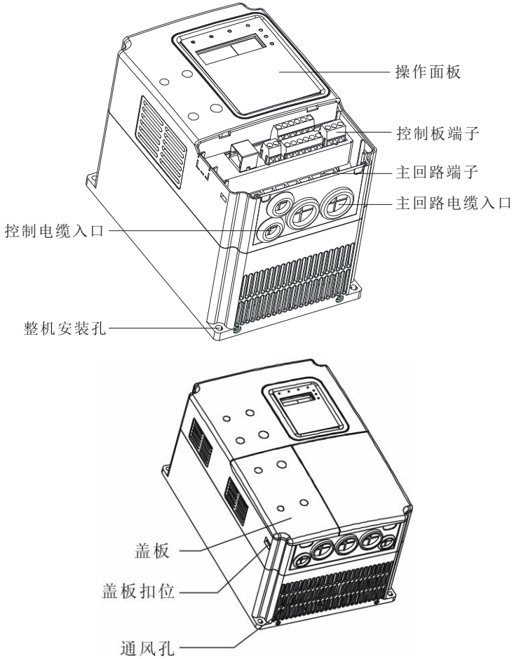
图 1-2 15KW 及以下塑料外壳变频器各部件名称
