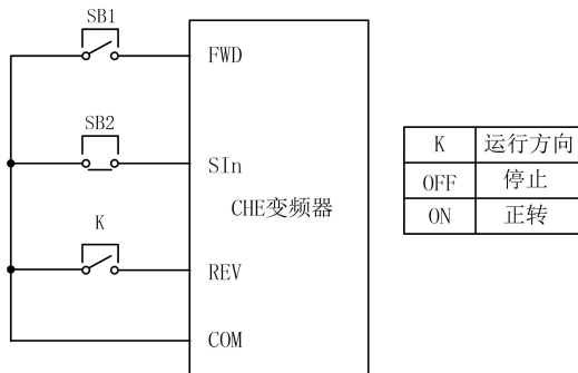
图 6-10 三线式运转模式 1 示意图
