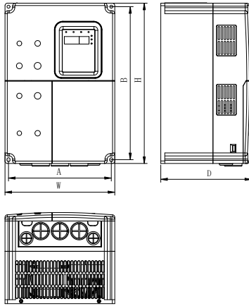
图 1-4 15kW 以下机型的外形尺寸
