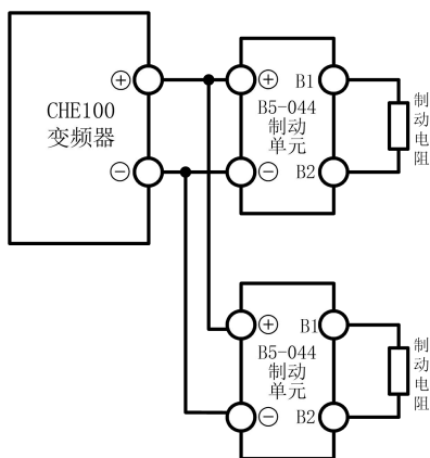
图 10-3 制动单元的并联连接
