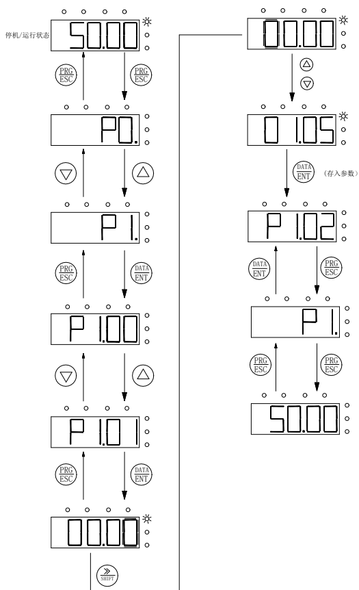
图 5-2 三级菜单操作流程图
