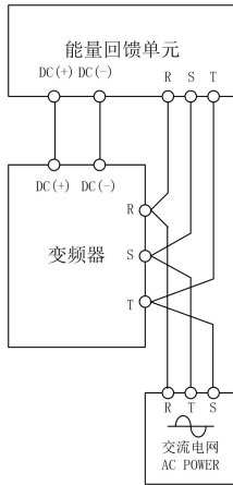
图 4-12 能量回馈单元连接图
