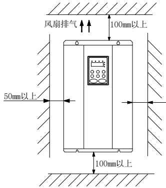
图 3-2 安装的间隔距离
