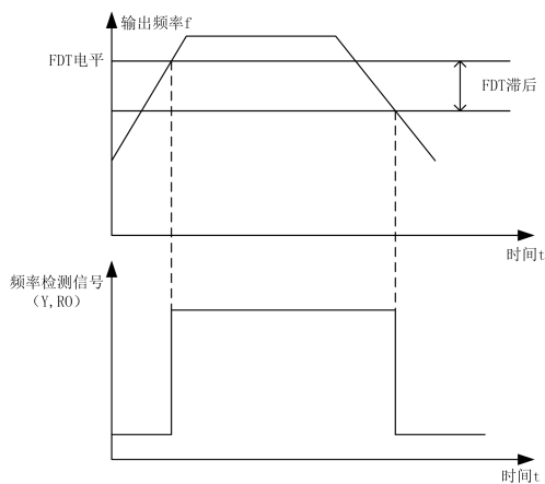
图6-16 FDT电平示意图
