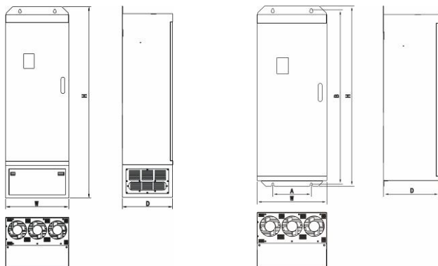
图 1-6 132KW~315KW 机型(有底座和无底座)外形尺寸
