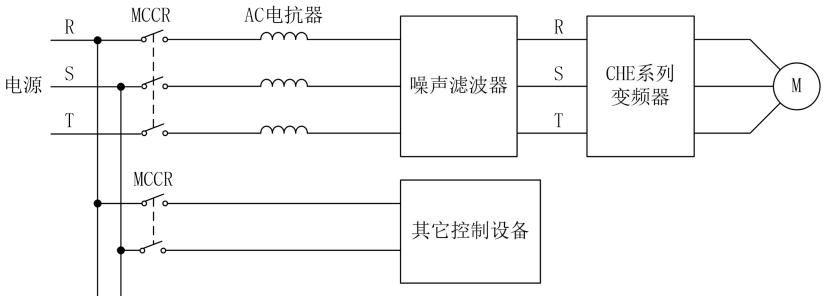
图 4-10 主回路电源侧连接图
