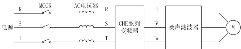
图 4-11 主回路电机侧连接图
