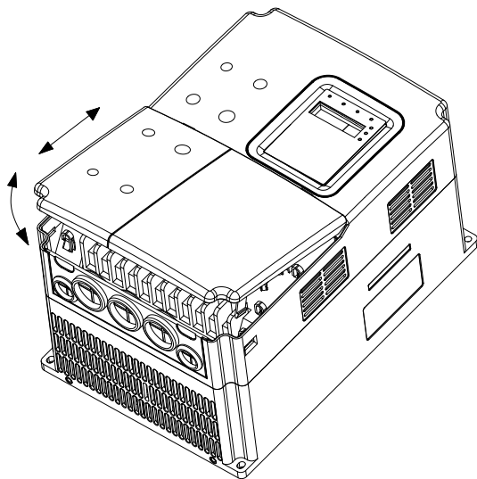
图 3-8 塑胶盖板的拆卸和安装示意图
