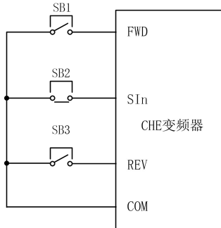
图6-11 三线式运转模式2示意图
