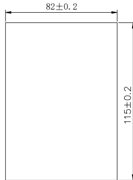
图 3-7 外引键盘的开孔尺寸
