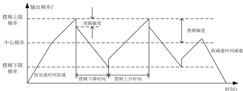
图6-15 摆频运行示意图
