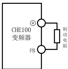
图 10-1 制动电阻的安装
