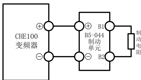
图 10-2 制动单元的连接
