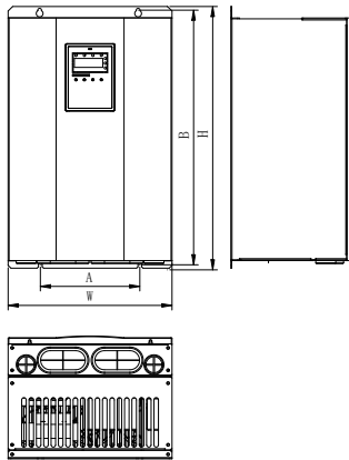
图 1-5 18.5KW~110KW 以上机型外形尺寸
