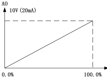
图6-13 给定量与模拟量输出的对应关系
