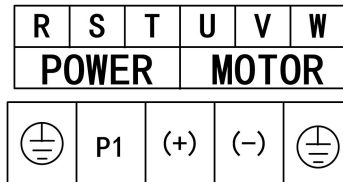
图 4-6 主回路接线端子图(132KW~315KW)
