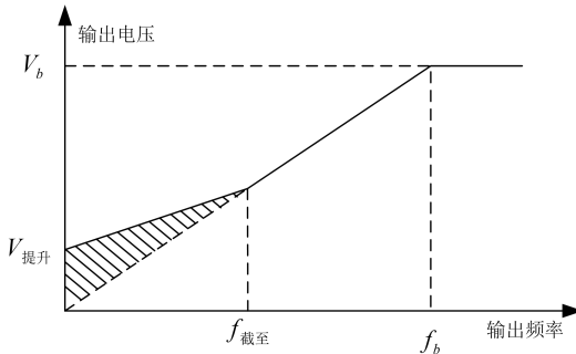
图6-7 手动转矩提升示意图
