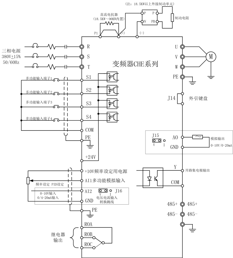
图 4-9 标准接线图
