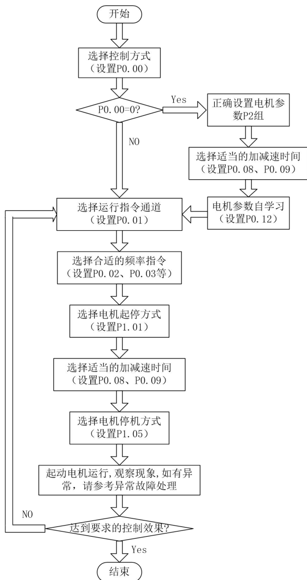
图 5-3 快速调试流程图
