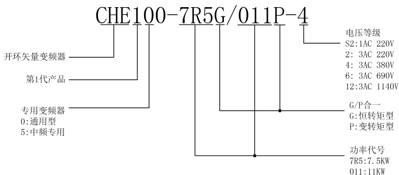
图 1-1 变频器铭牌说明
