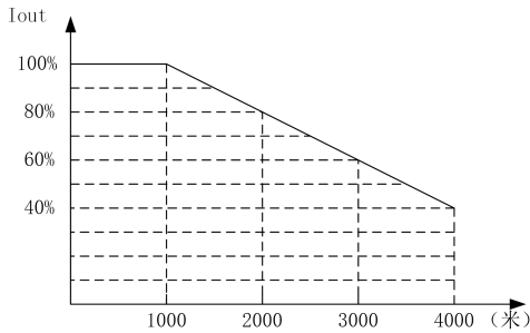
图 3-1 安装地点的海拔高度
