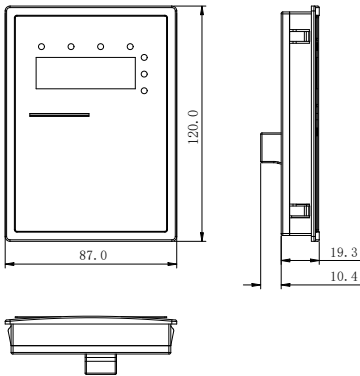
图 3-6 外引键盘的安装尺寸
