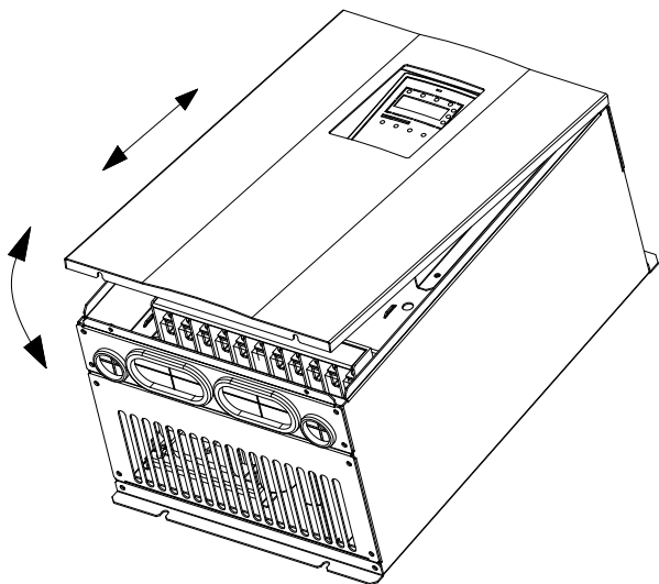
图 3-9 钣金盖板的拆卸和安装示意图
