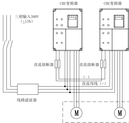
图 4-13 共直流母线的连接
