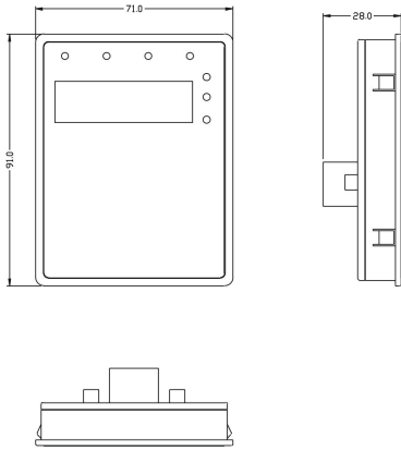
图 3-4 外引键盘（小）的安装尺寸
