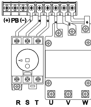
图 4-9 7R5G/011P-015G/018P 主回路端子示意图
