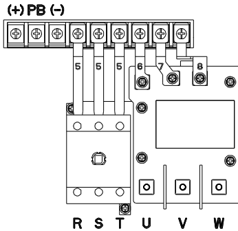
图 4-10 018G/022P-022G/030P 主回路端子示意图
