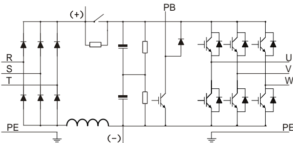
图 3-2 018G/022P~110G（含）主回路简图
