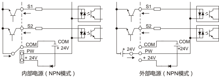
图 4-17 NPN 模式示意图
