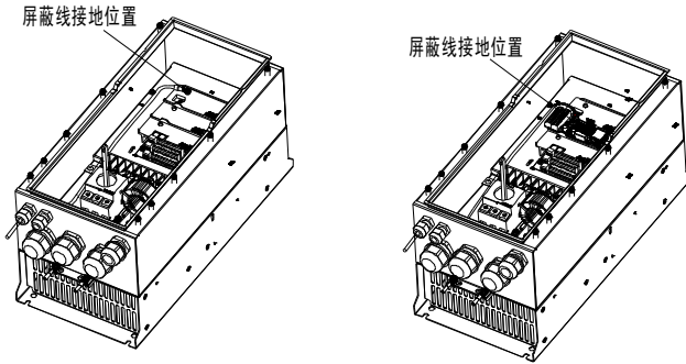
图 A-3 扩展卡地线连接示意图
