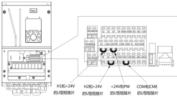
图 4-16 U 型短接位置示意图
