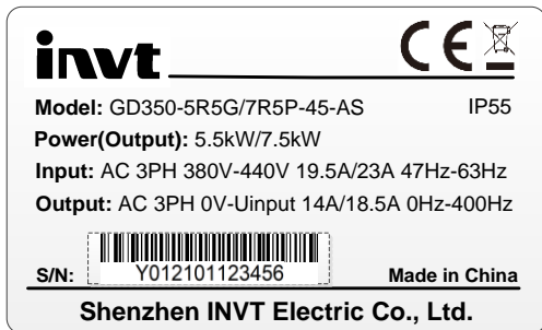
图 3-3 产品铭牌
