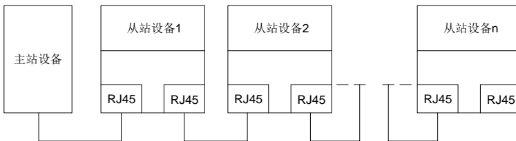
图 A-5 线型网络拓扑电气连接图
