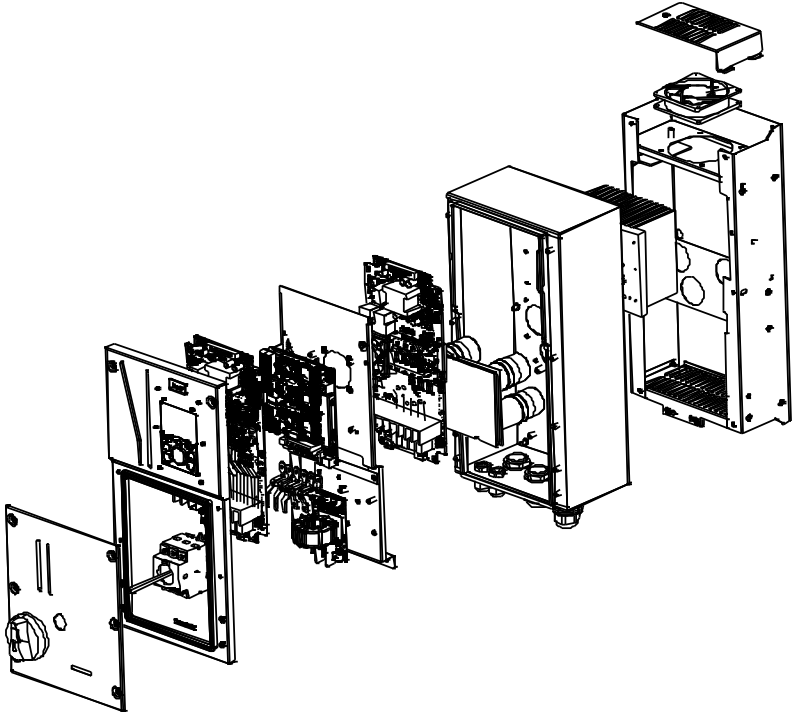
图 C-1 变频器结构图
