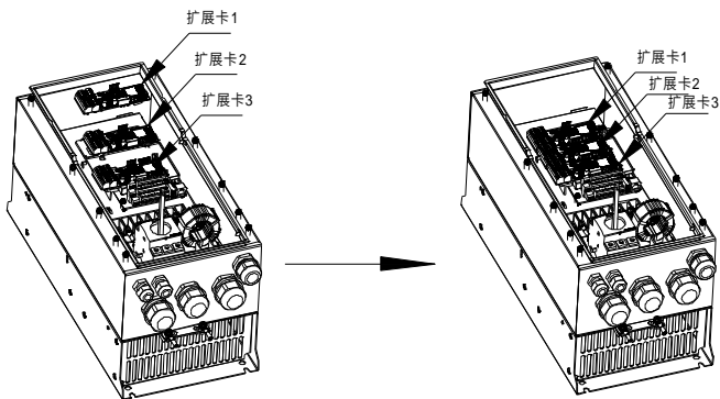
图 A-1 7R5G/011P（含）以上机型效果图
