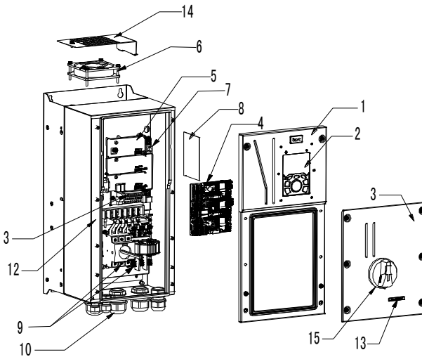
图 3-5 产品结构示意图
