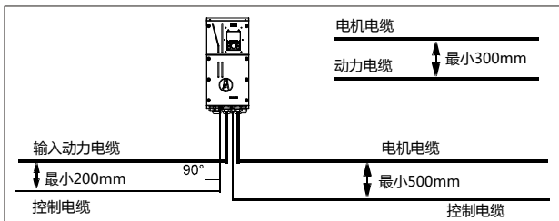
图 D-4 布线距离
