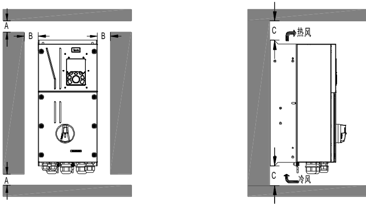
图 4-3 单台安装
