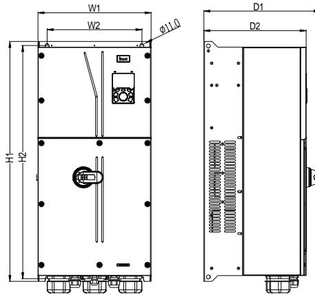
图 C-3 045G/055P~110G 壁挂安装示意图
