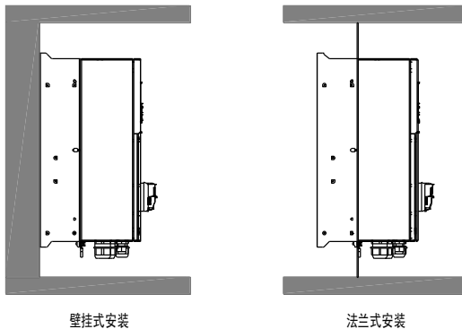
图 4-2 安装方式
