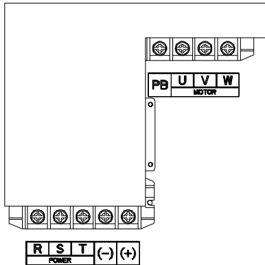
图 4-12 045G/055P-055G/075P 主回路端子示意图
