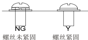
图 4-14 螺丝安装是否正确示意图
