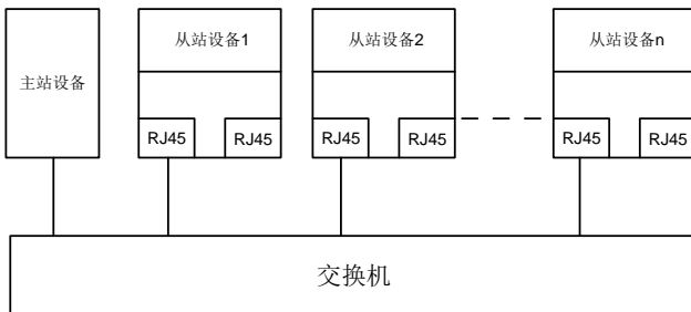
图 A-6 星型网络拓扑电气连接图
