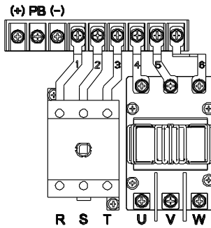
图 4-9 7R5G/011P-015G/018P 主回路端子示意图
