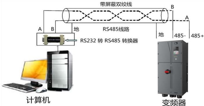
图 10-1 RS485 单机应用时的物理接线图
