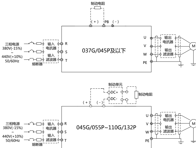
图 4-7 主回路接线图
