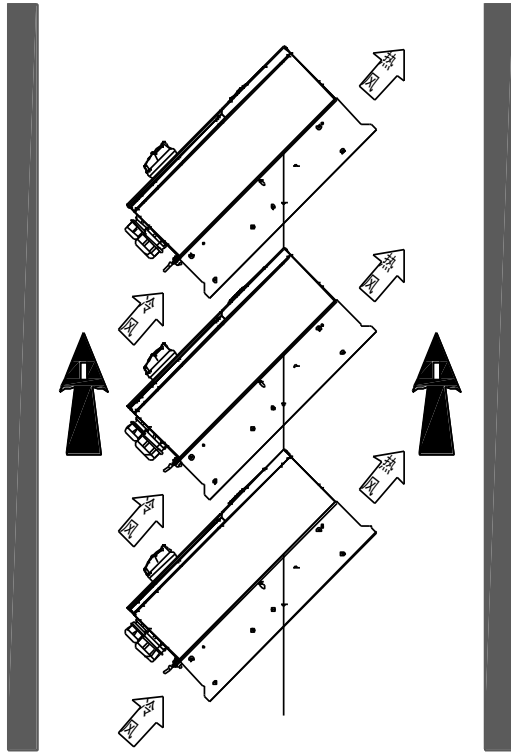
图 4-6 倾斜安装
