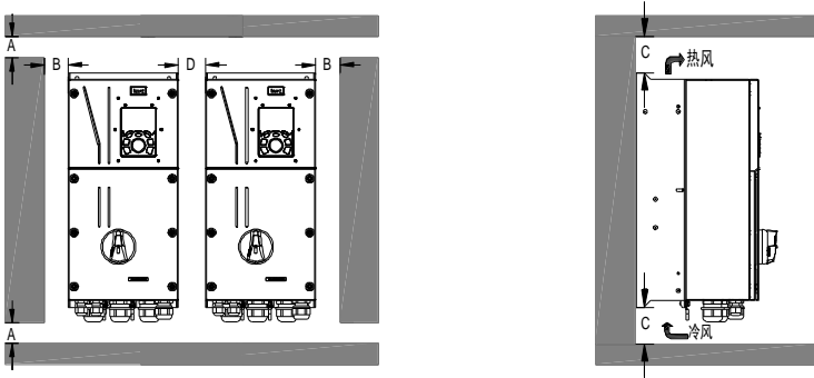
图 4-4 并行安装
