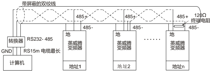
图 10-4 菊花接法运用图
