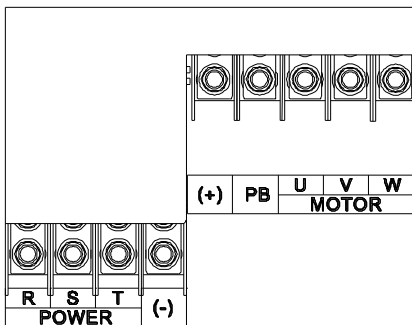
图 4-13 075G/090P-110G 主回路端子示意图
