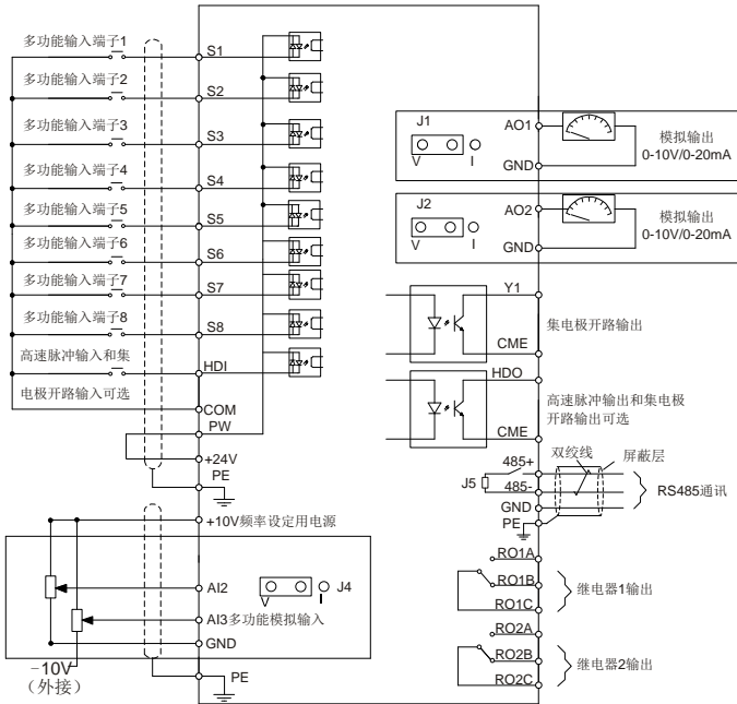
图 4-19 控制回路接线图
