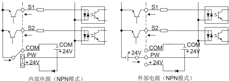
图 4-23 NPN 模式示意图
