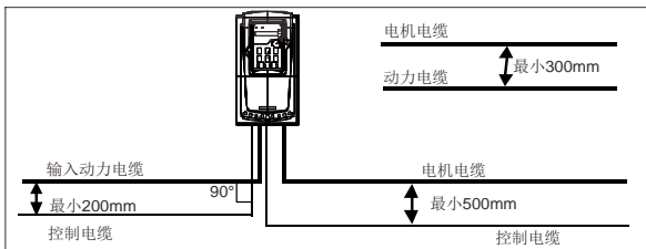
图 C-4 布线距离
