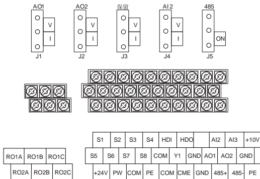
图 4 - 20 015G/018P 及以下控制端子示意图
