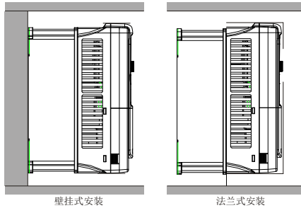
图 4-2 安装方式
