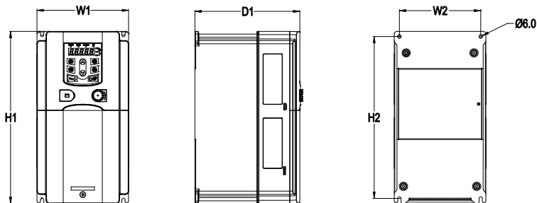
图 B - 3 0R7G~015G/018P 壁挂安装示意图
