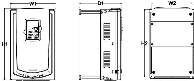
图 B - 4 018G/022P~030G/037P 壁挂安装示意图
