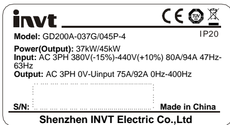
图 3-3 产品铭牌
