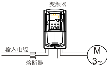
图 4 - 25 熔断器配置图
