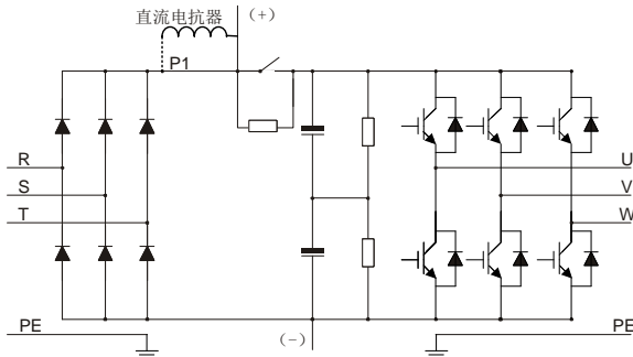
图 3 - 2 037G/045P 及以上主回路简图
