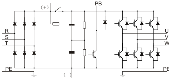
图 3 - 1 030G/037P 及以下主回路简图
