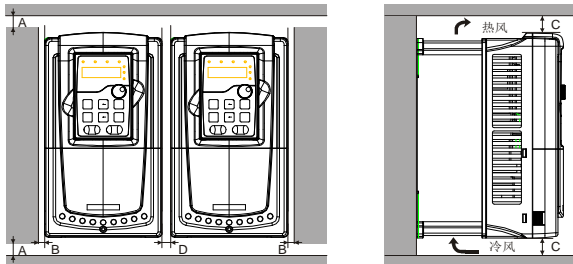
图 4-3 并行安装
