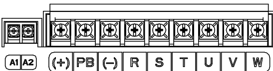
图 4 - 11 018G/022P 主回路端子示意图
