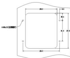
图 B - 2 037G/045P~500G 键盘安装架 (标配)
