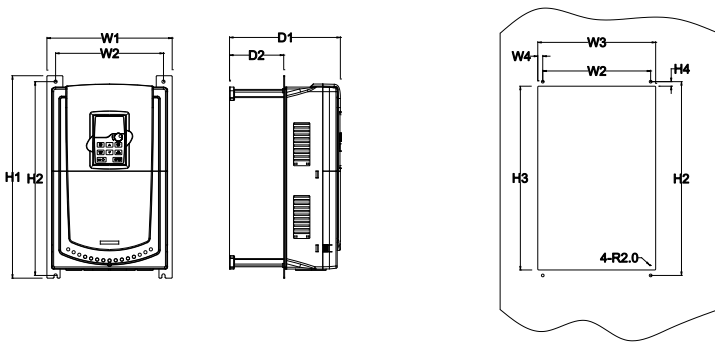
图 B - 9 018G/022P~030G/037P 法兰安装示意图
