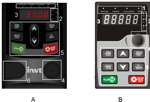
图 5-1 键盘示意图
