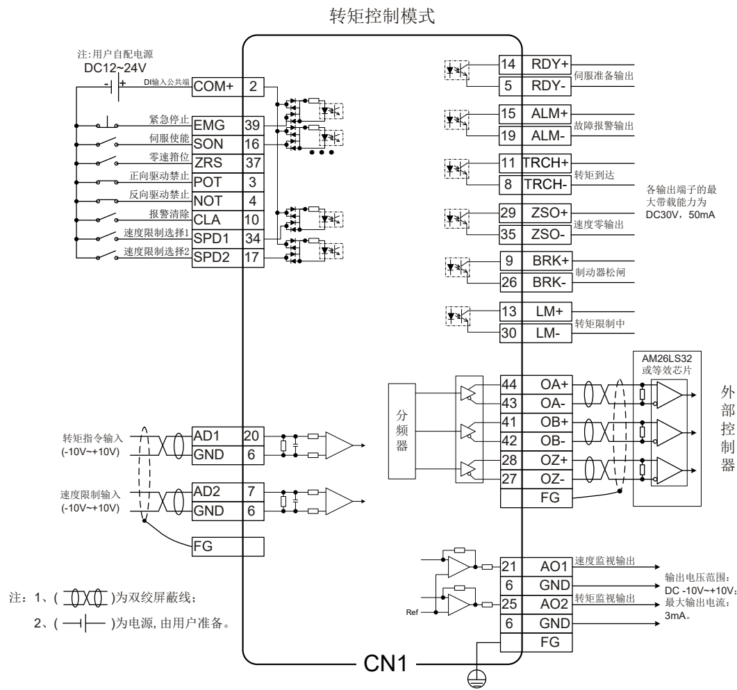
CN1端子
