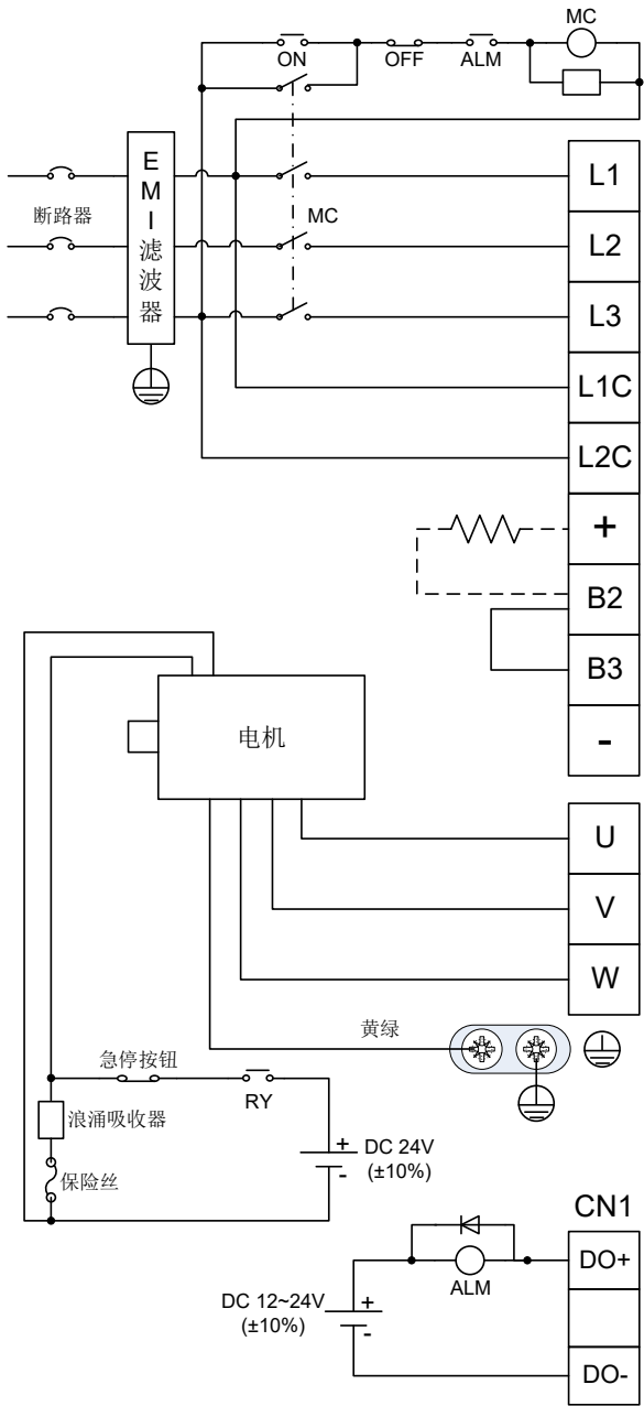
主回路端子配线图
