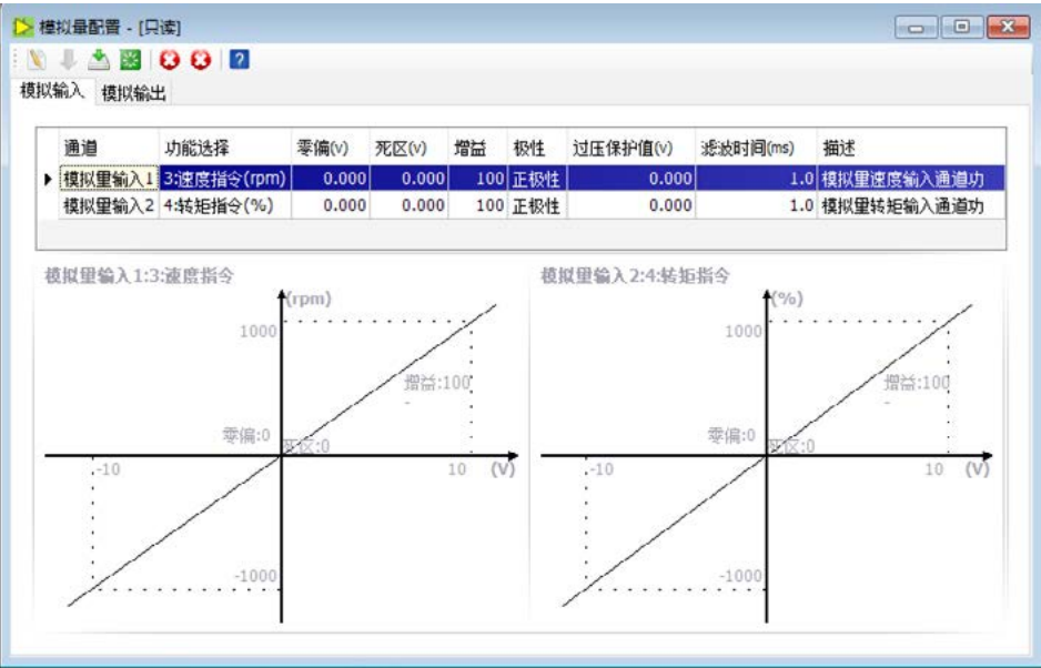
模拟量输入输出可以在图示中设定增益、零偏、死区等参数
