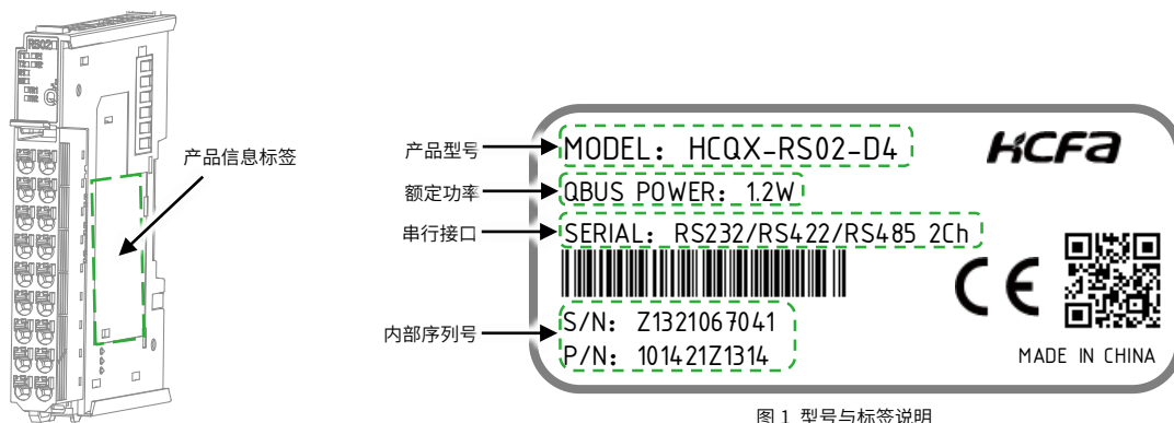
图 1 型号与标签说明
