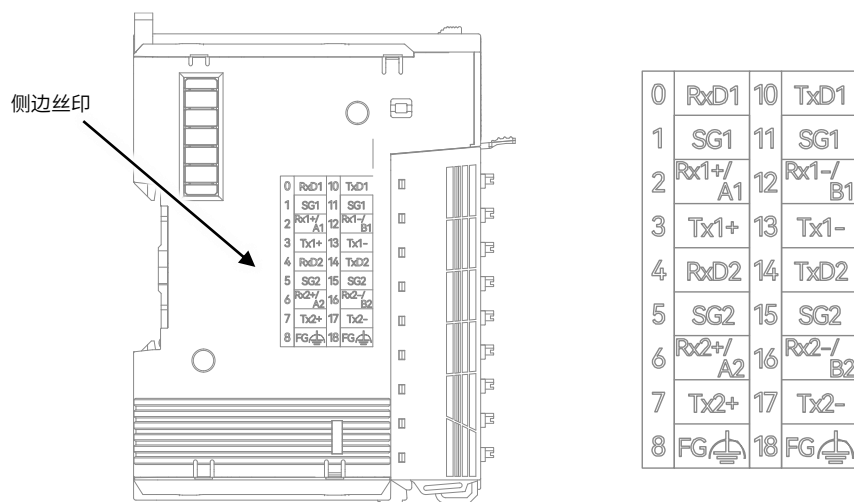
图4 HCQX-RS02-D4 模块侧边丝印
