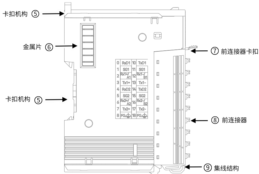
图 3 HCQX-RS02-D4 模块左视图
