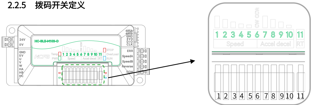
图 8 HC-BLE103-D IO 拨码开关说明图
