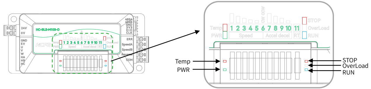
图 9 HC-BLEM103-D LED 指示灯说明图
