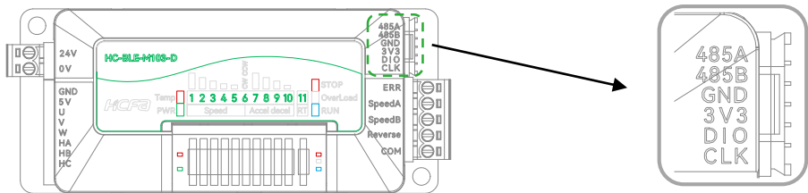
图 5 HC-BLEM103-D 程序烧写口说明图
