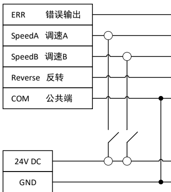
图 7 HC-BLE103-D 跳线调速口说明图
