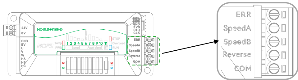
图 6 HC-BLE103-D IO 信号端口说明图
