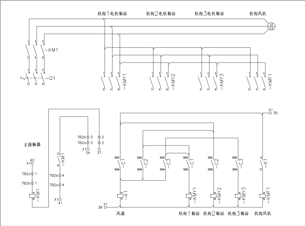
(H1~H4 机型电气图)
