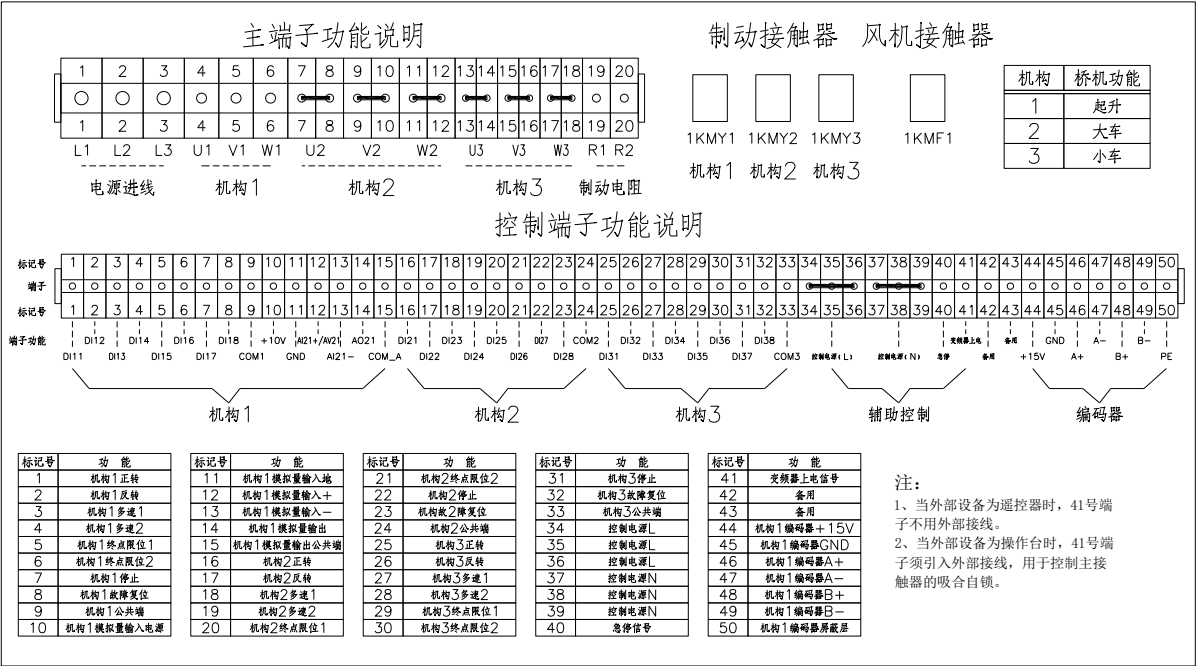
(H1~H4 机型端子功能图)
