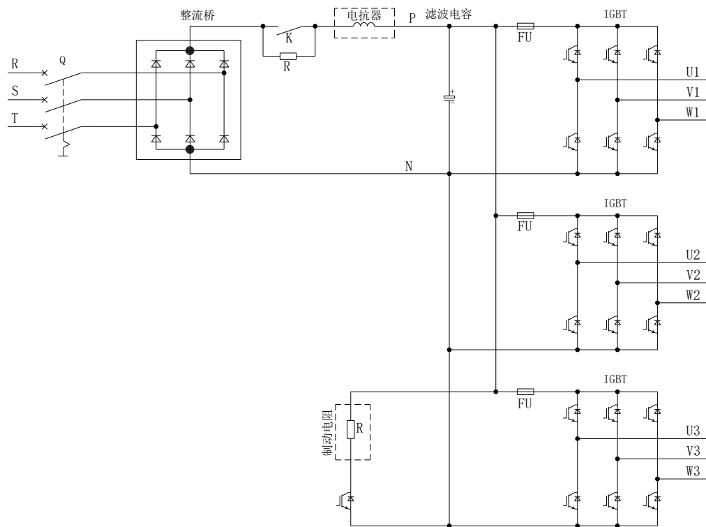
37KW 以下机器不配置电抗器和主变频器的快熔
