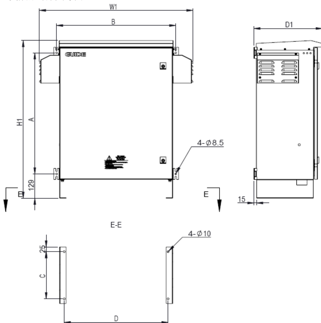
外形尺寸及安装尺寸
