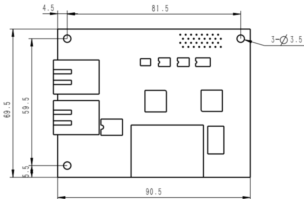
图5 PROFINET 模块尺寸（单位 mm）
