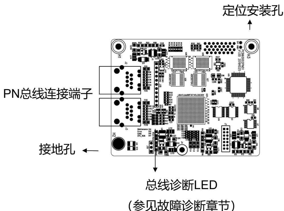
图1 GDHF-PN02 总线卡布局图
