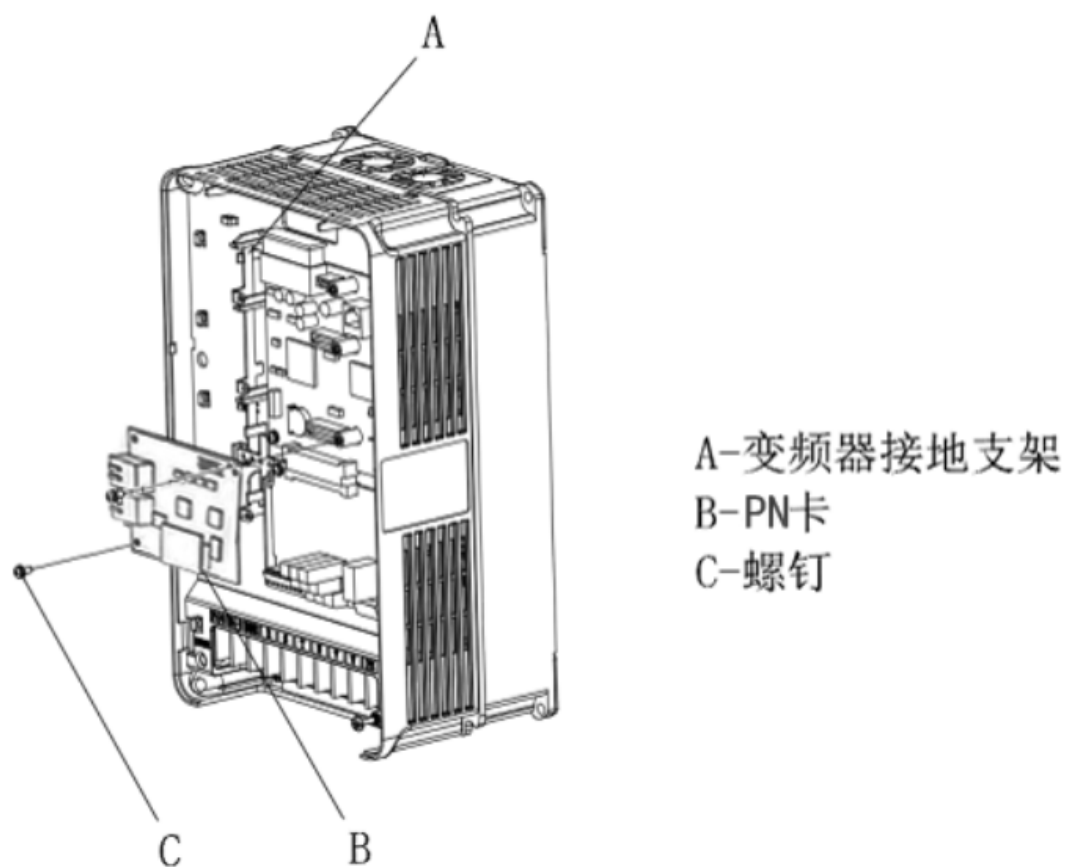
图2 总线卡的安装与接地
