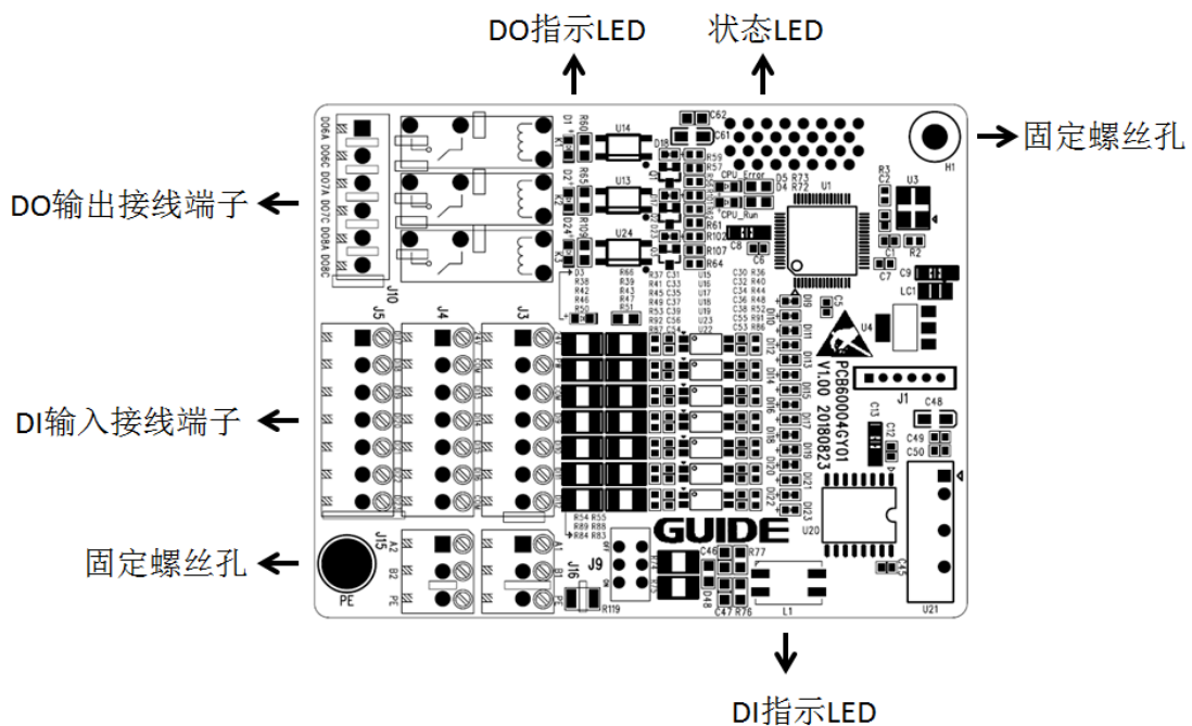
GDHF-GY02 工艺卡布局图
