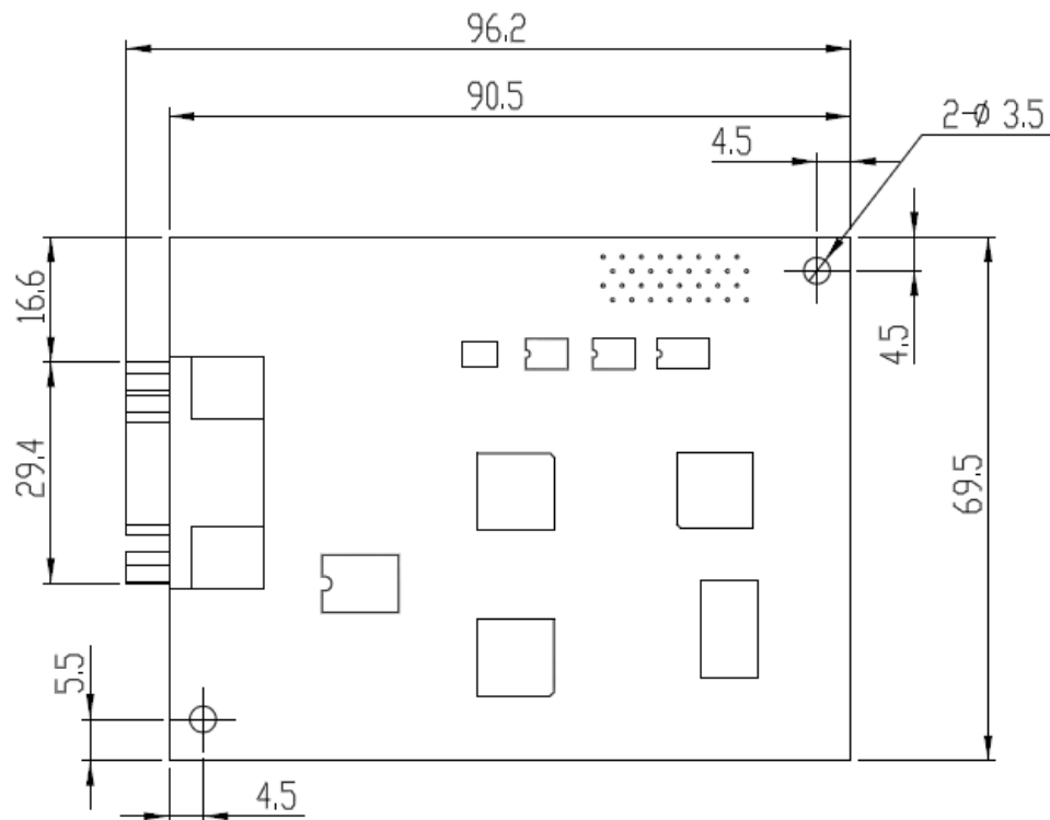
图5 PROFIBUS_DP 模块尺寸（单位 mm）
