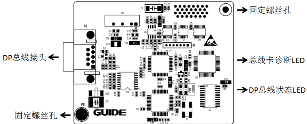
图1 GDHF-DP03 总线卡布局图
