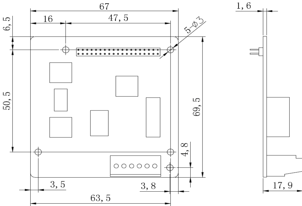
图6 PROFIBUS_DP 模块尺寸（单位 mm）
