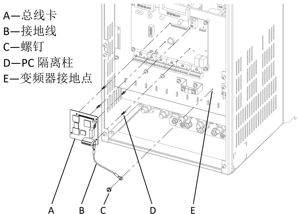
图2 总线卡的安装与接地（37kW 以下变频器）
