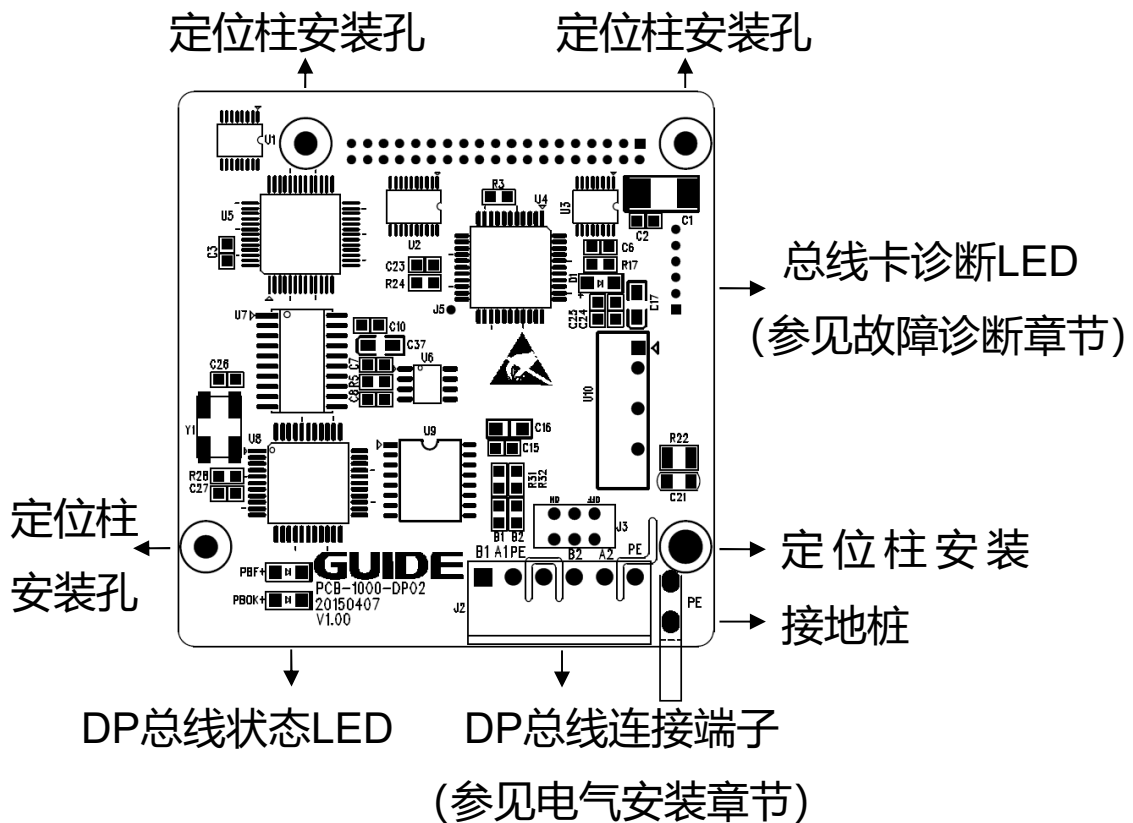
图1 GDHF-DP02 总线卡布局图
