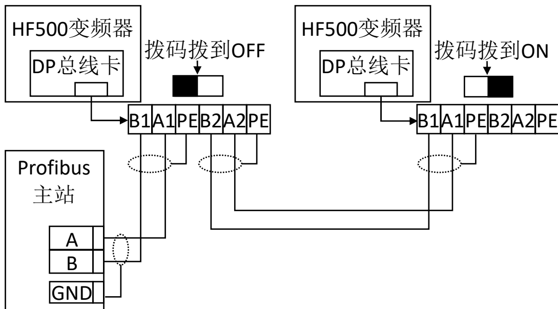
图4 标准 PROFIBUS 电缆接线图
