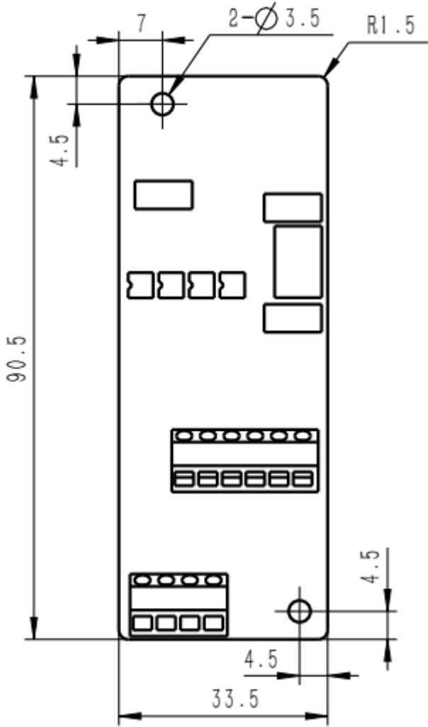
图 1 PG 卡安装示意图及 PG 卡外形尺寸
