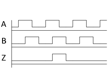
图 4 编码器单端输出信号
