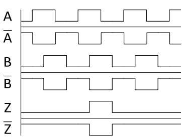
图 3 编码器差分输出信号
