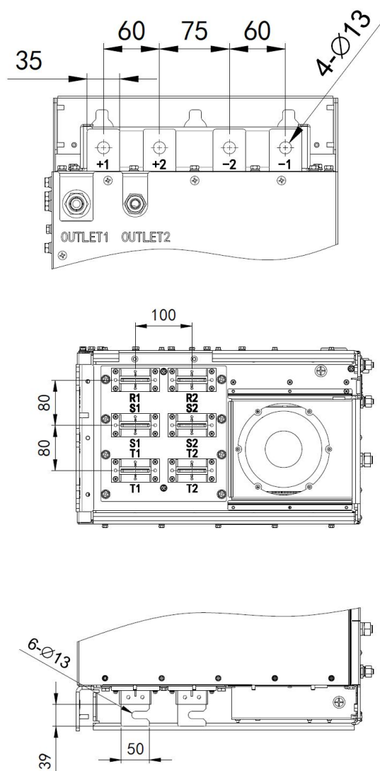
二极管整流单元主接线端子示意图
