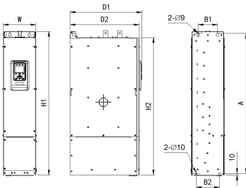
B4 机型整流回馈模块外形示意图
