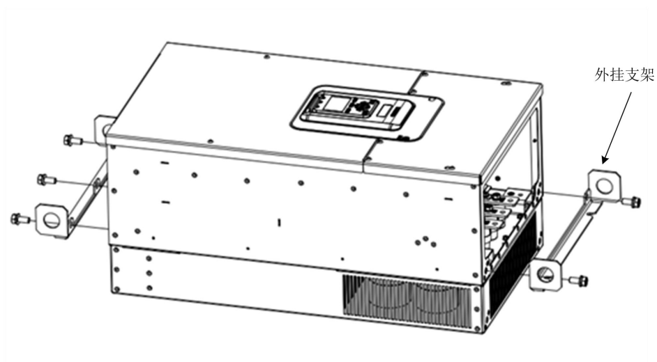
图 3-2 钣金结构安装外挂支架示意图
