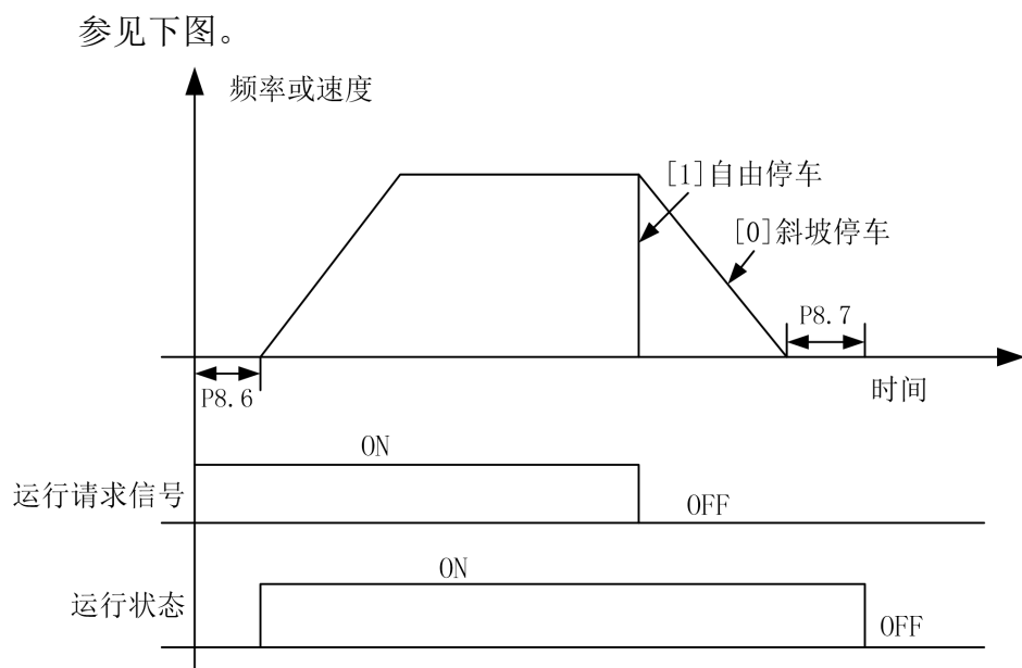
停车方式控制图
