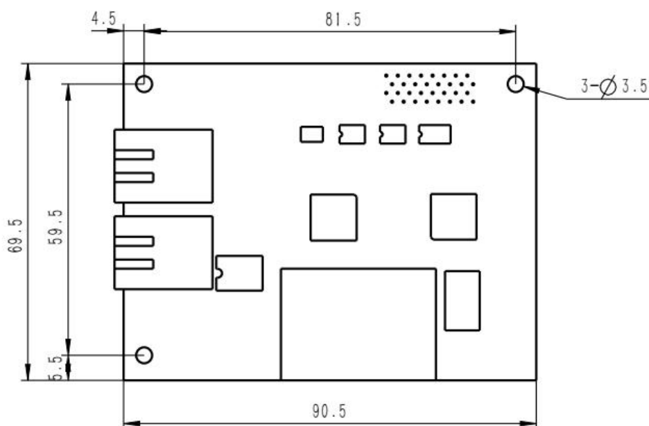
PROFINET 模块尺寸 (单位 mm)
