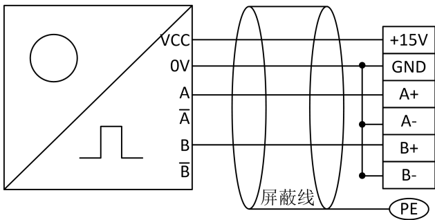
常用推挽输出（单端接线方式）编码器应用举例：
