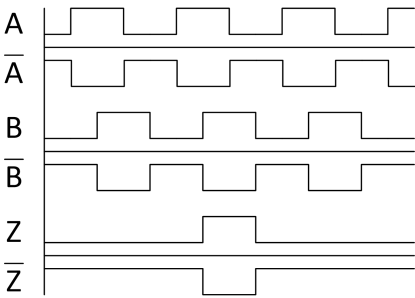
编码器差分输出信号
