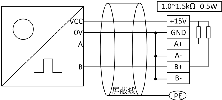
常用集电极开路输出编码器应用举例：
