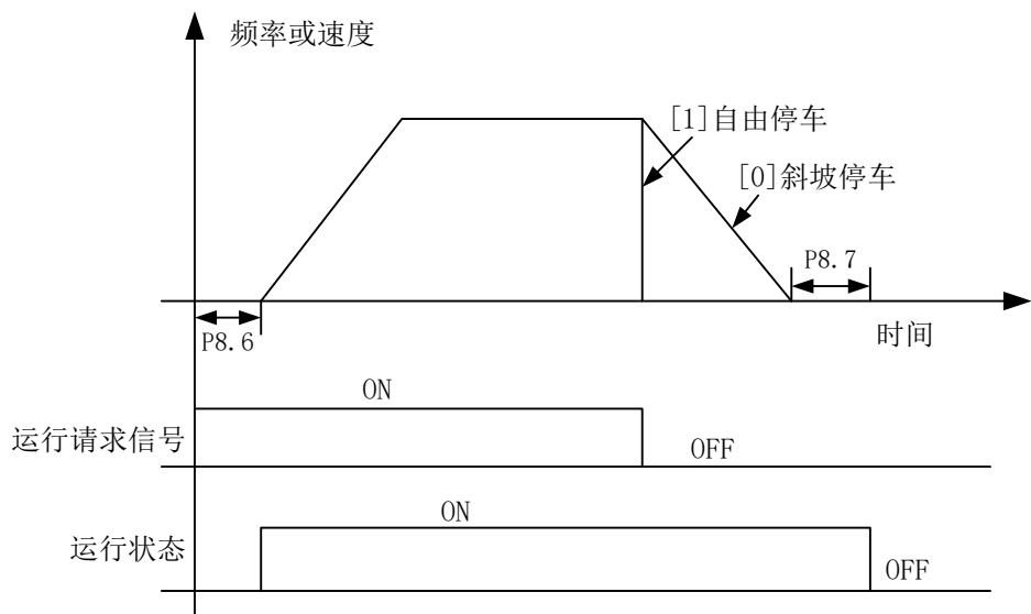
停车方式控制图
