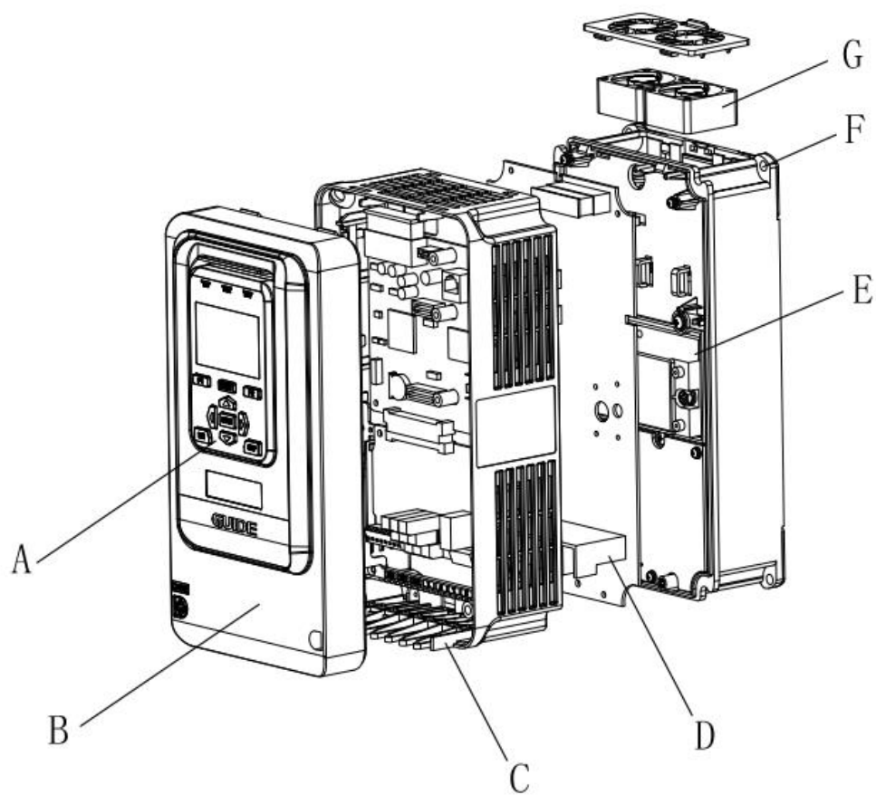
A-操作器 B-面盖 C-进线板 D-主回路端子 E-散热器 F-安装孔 G-冷却风扇
