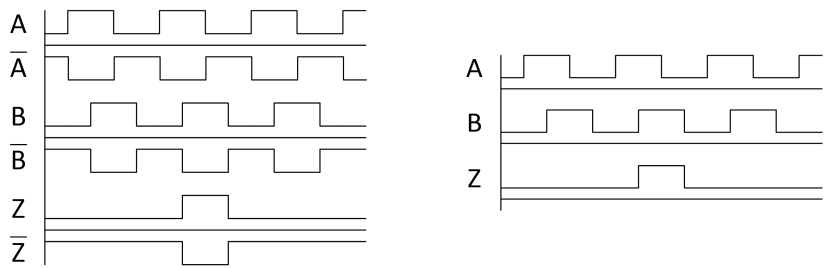
编码器差分输出信号 编码器单端输出信号
