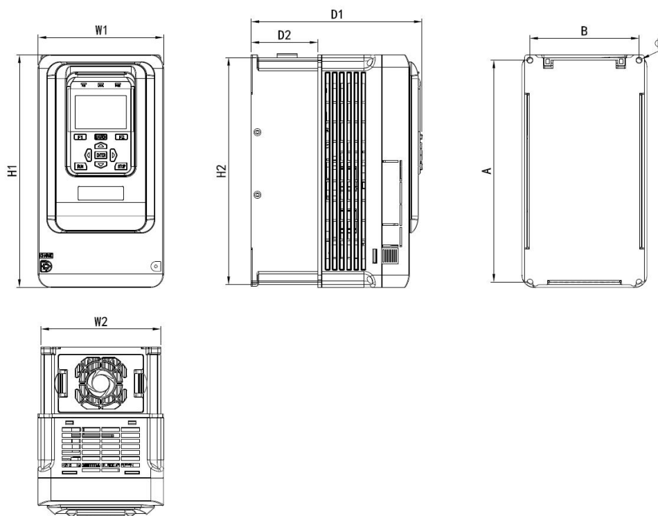
N2 机型尺寸及安装尺寸示意图
