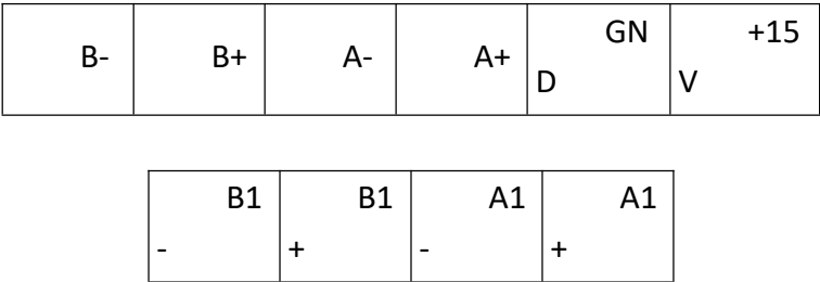
接线端子示意
