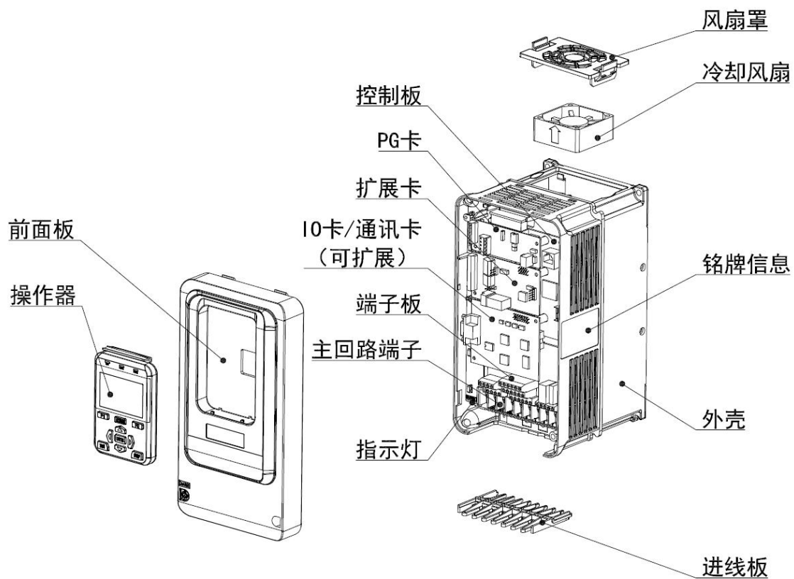
N2 产品部件示意图（三相 380V~480V，3.7kW~11kW）
