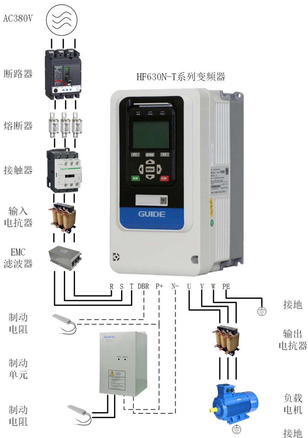
HF630N-T 变频系统外围电气元件的使用说明
