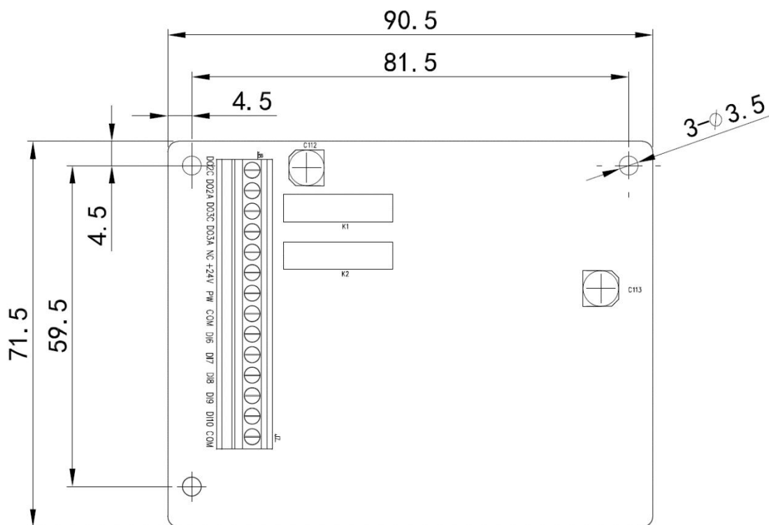
IO 扩展卡选件 GDHF-AIOX2 尺寸 (单位 mm)
