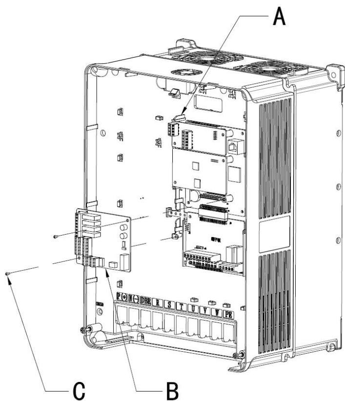
IO 扩展卡的安装
