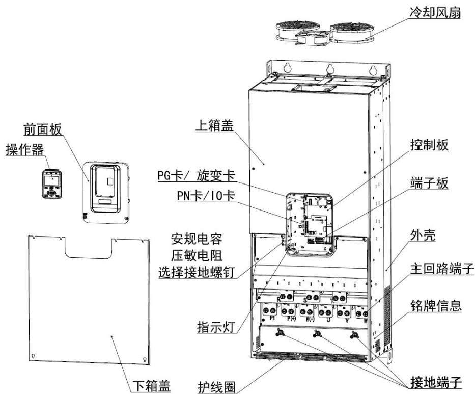
N9 产品部件示意图 (三相 380V~480V, 250kW~280kW)
