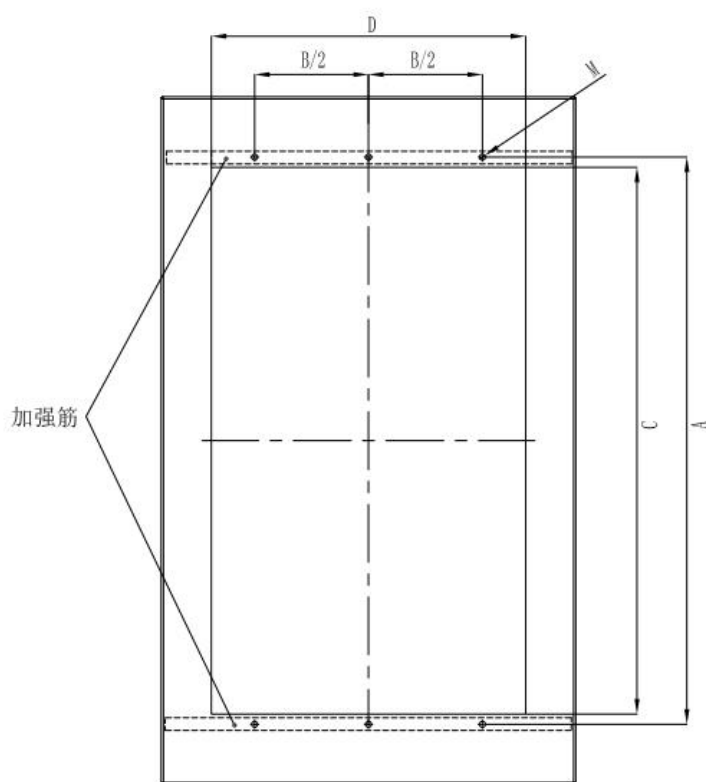
图 3-9 钣金结构 17-19 机型嵌入式安装板示意图
