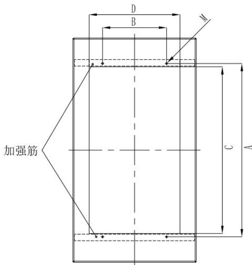
图 3-8 钣金结构 15-16 机型嵌入式安装板示意图
