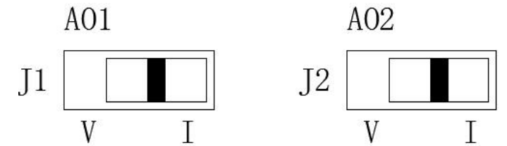
图 a. 模拟量输出为电流时，跳线示意图
