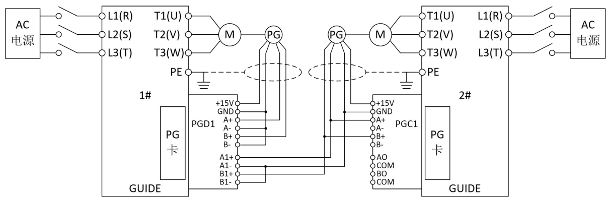
同步功能应用中，编码器为单端输出信号的接线示意图：
