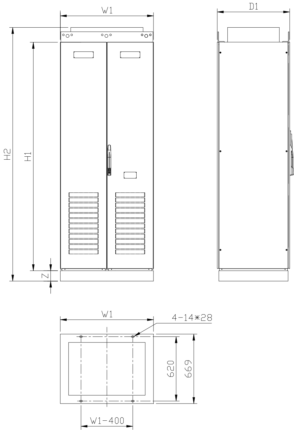
逆变器外形示意图
