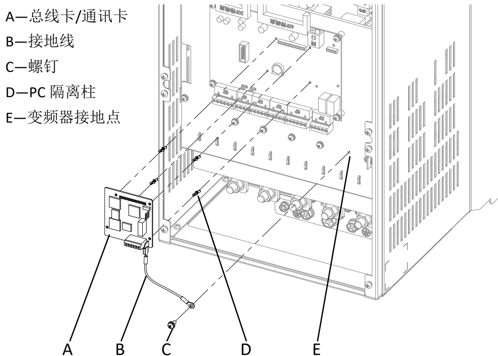
37kW 以上变频器总线卡/通讯卡的安装与接地
