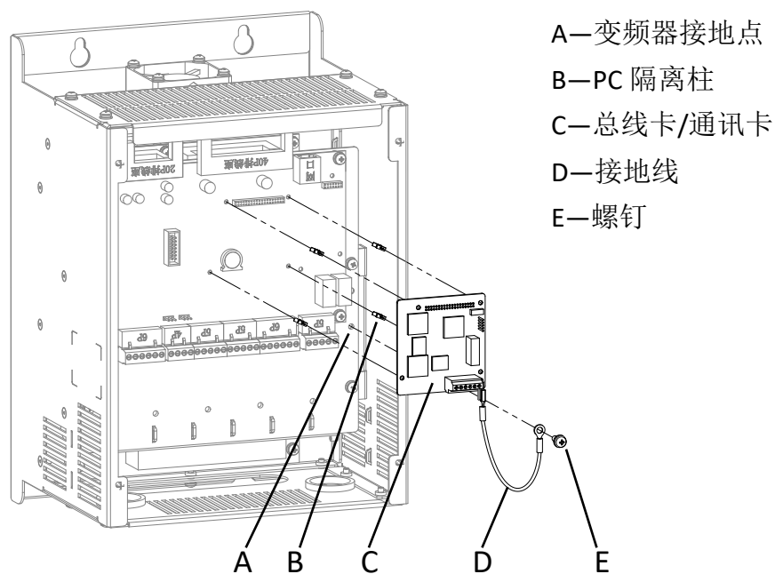
37kW 及以下变频器总线卡/通讯卡的安装与接地
