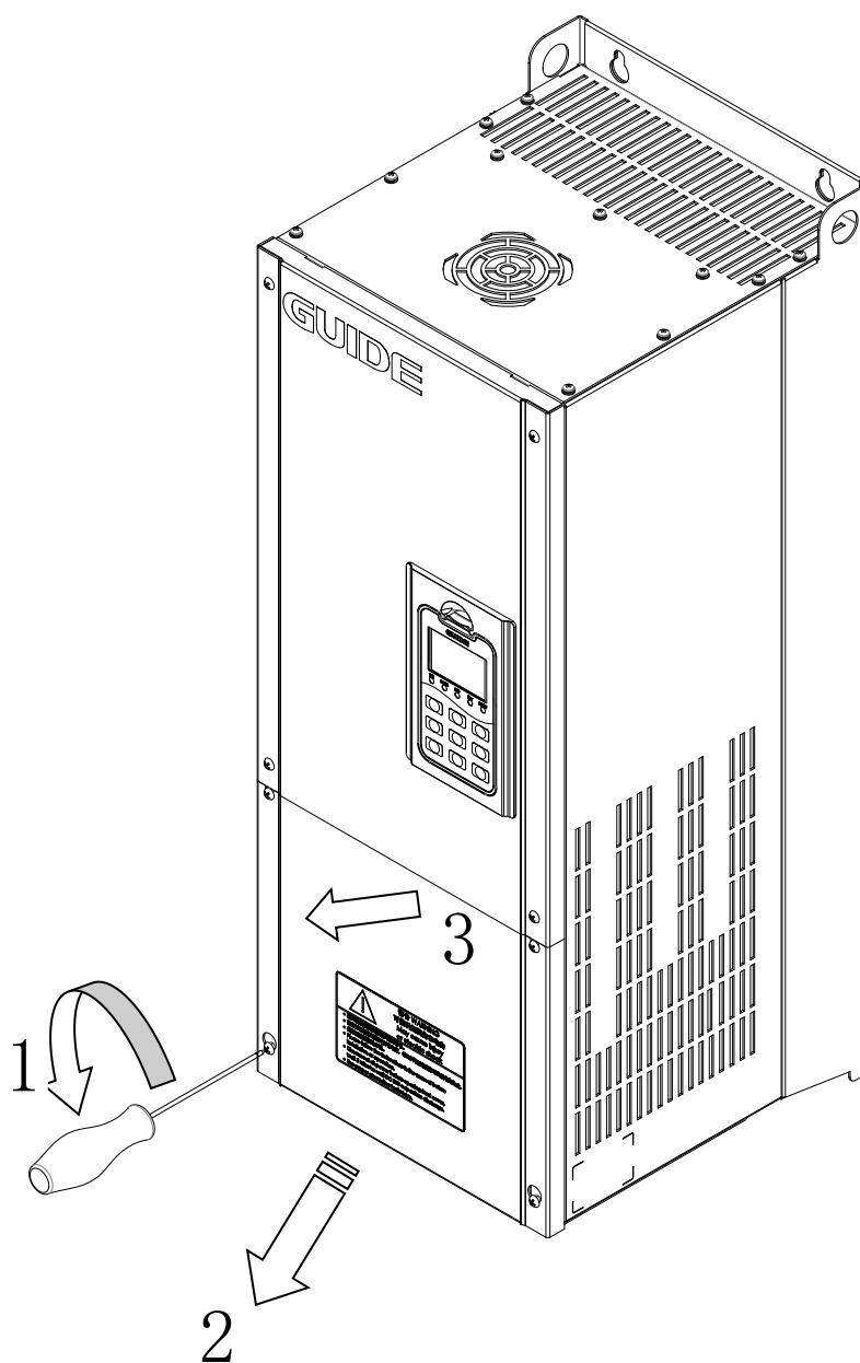
图 3-1 变频器盖板的拆卸和安装
