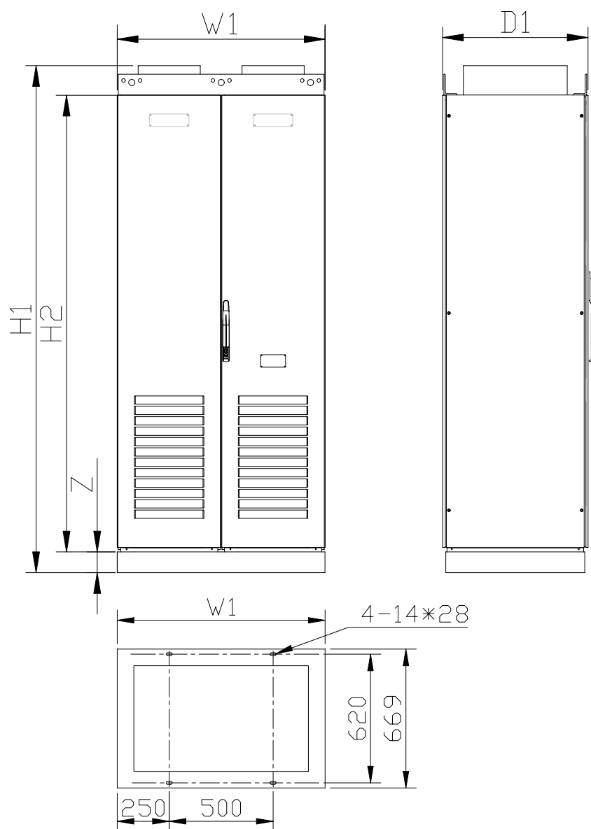
F10 机型示意图
