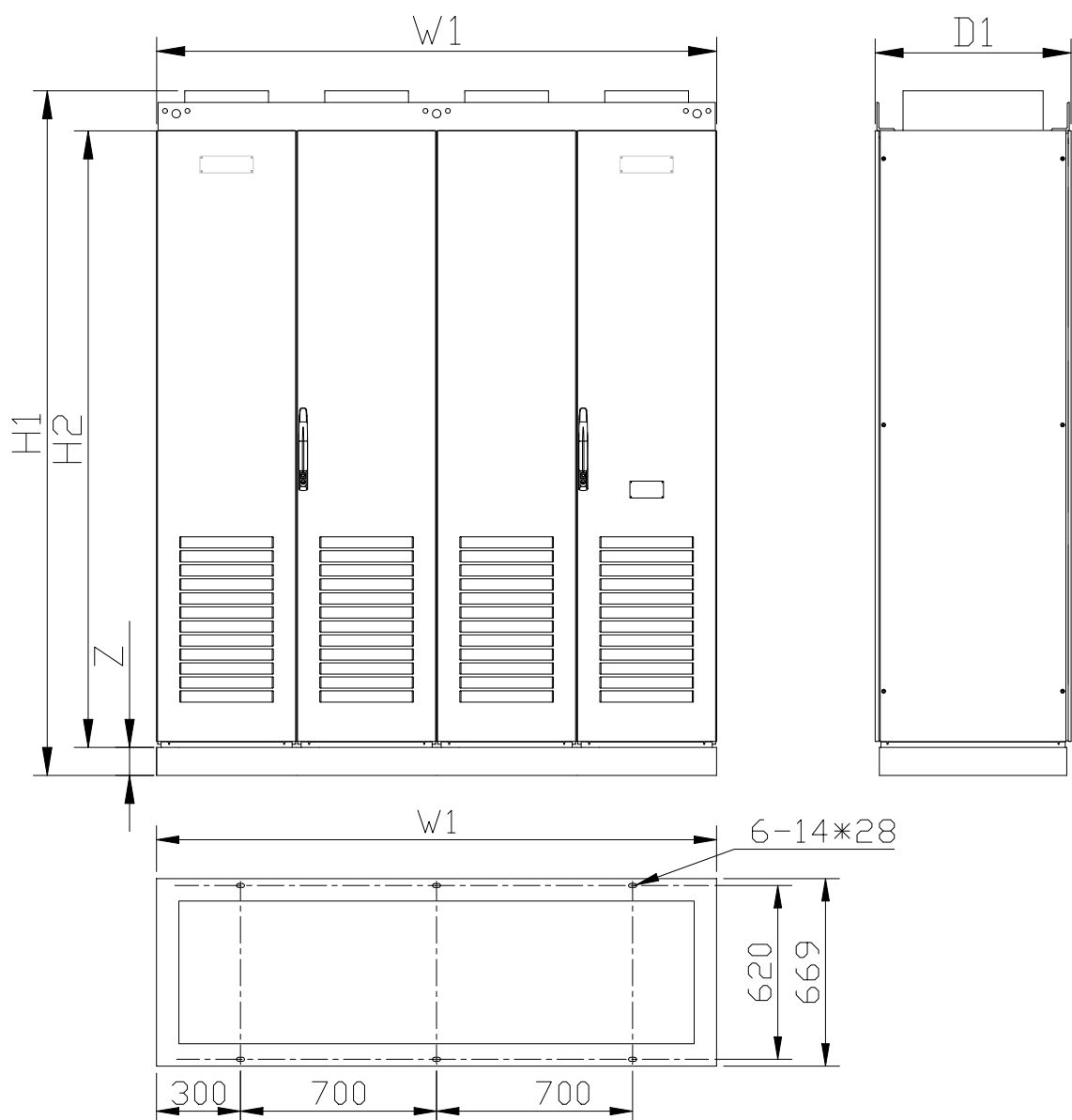
F11 机型示意图
