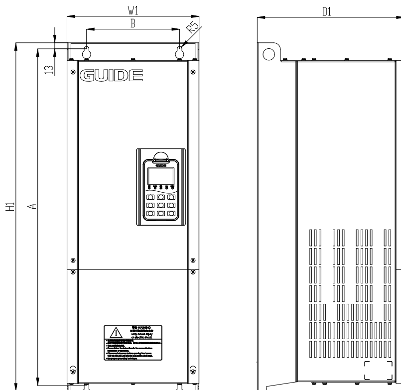
F3 机型示意图
