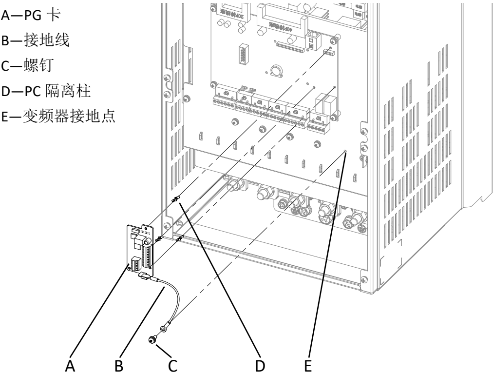
37kW 以上变频器 PG 卡的安装与接地
