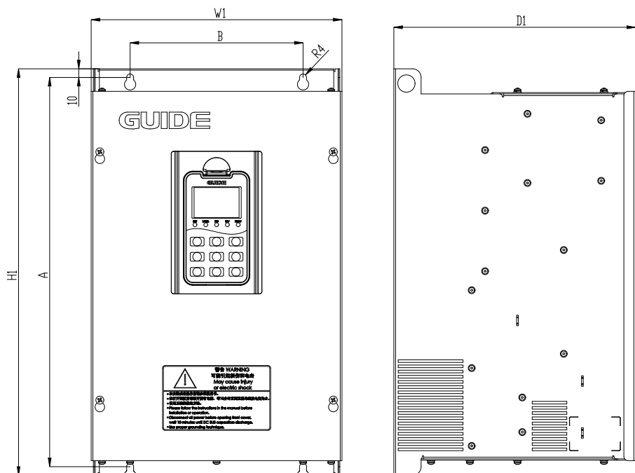
F2 机型示意图
