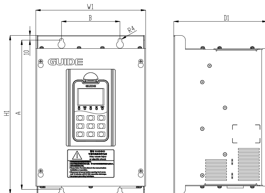
F0 机型示意图
