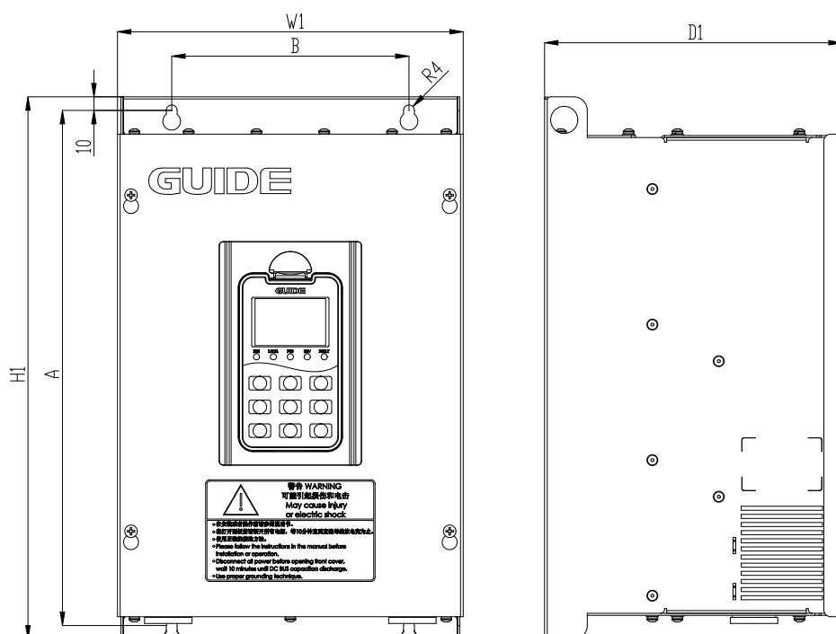
F1 机型示意图
