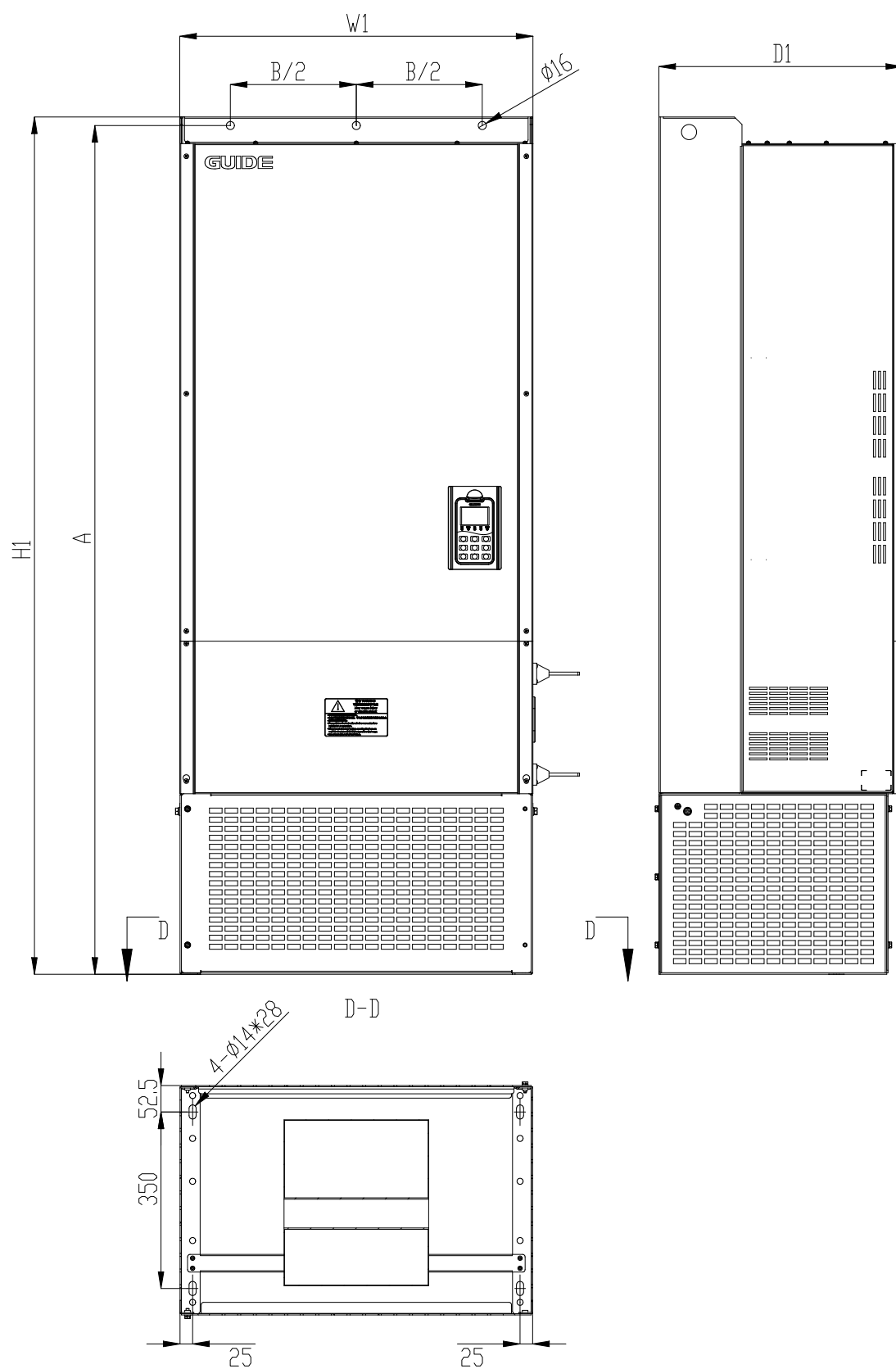
F9 机型示意图
