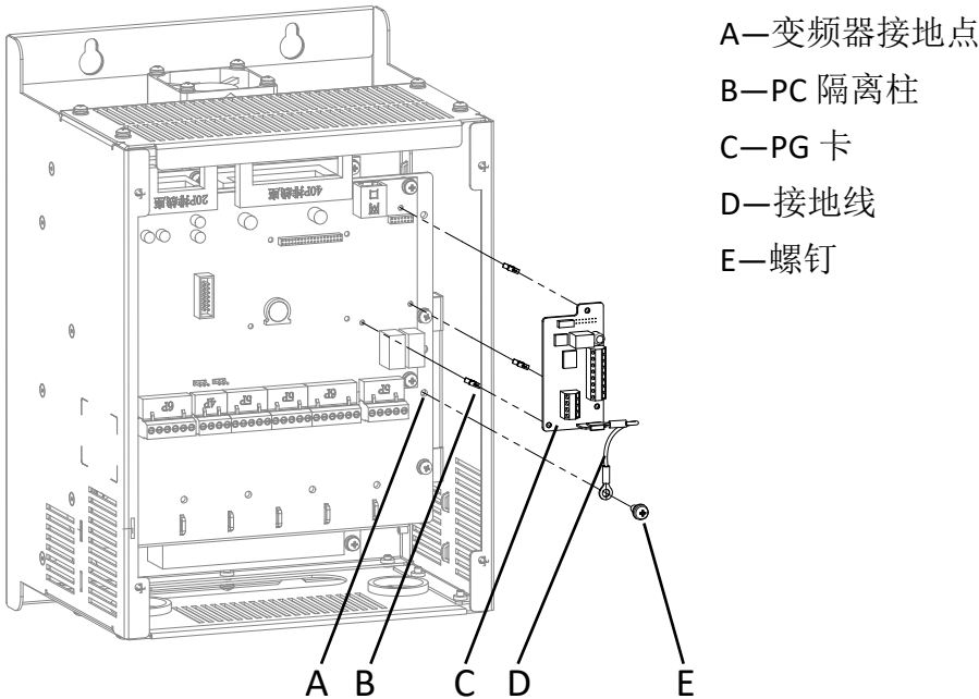
37kW 及以下变频器 PG 卡的安装与接地
