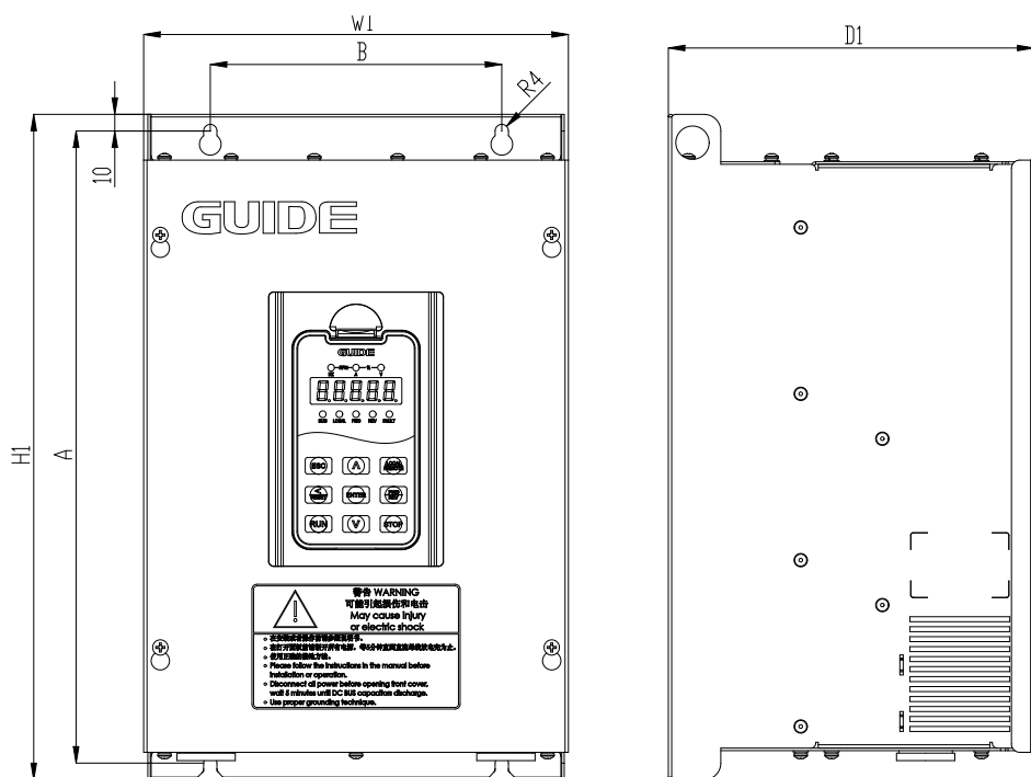
F2 机型示意图
