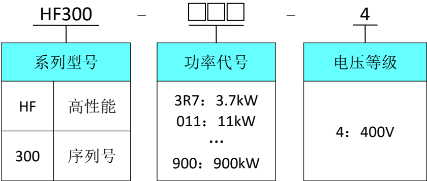
图 2-1 产品型号含义
