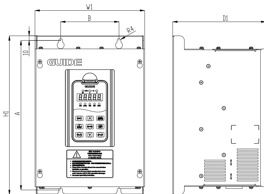
F1 机型示意图
