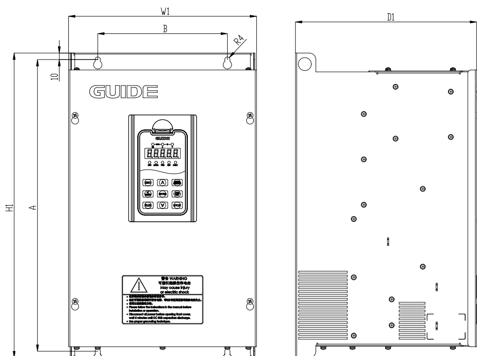
F3 机型示意图
