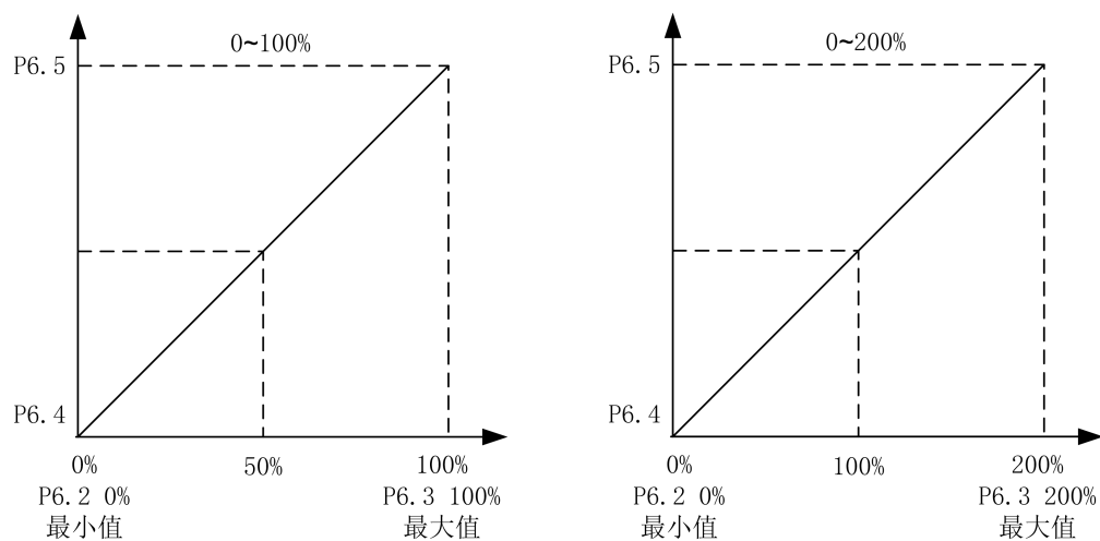
(a) 输出设置范围为 0~100%
