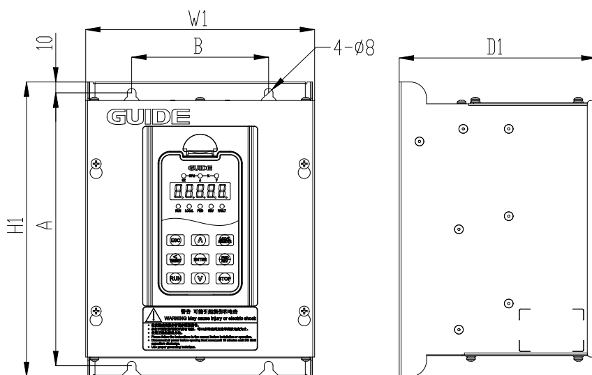
F0 机型示意图
