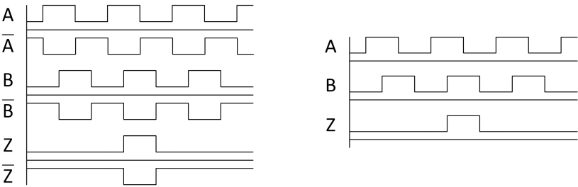
编码器差分输出信号 编码器单端输出信号
