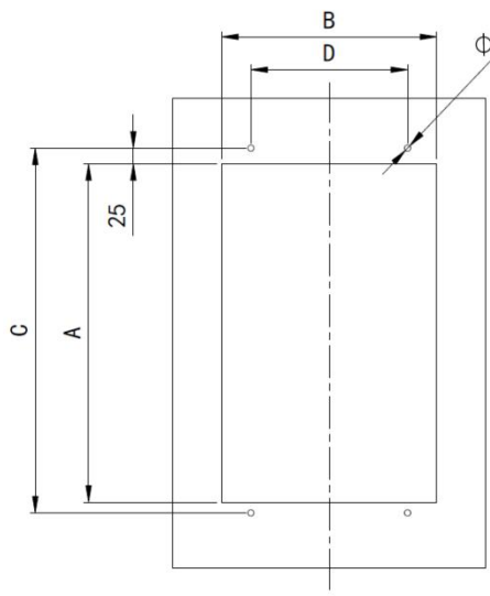
S3 安装开孔尺寸图
