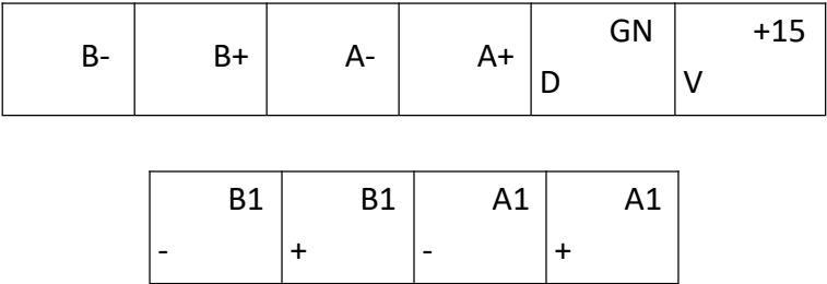
接线端子示意图
