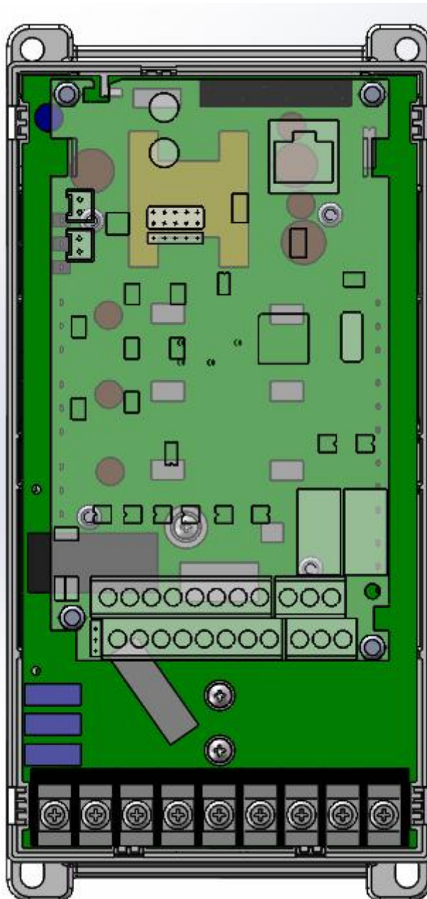
GF630N01 控制板安装位置示意图
