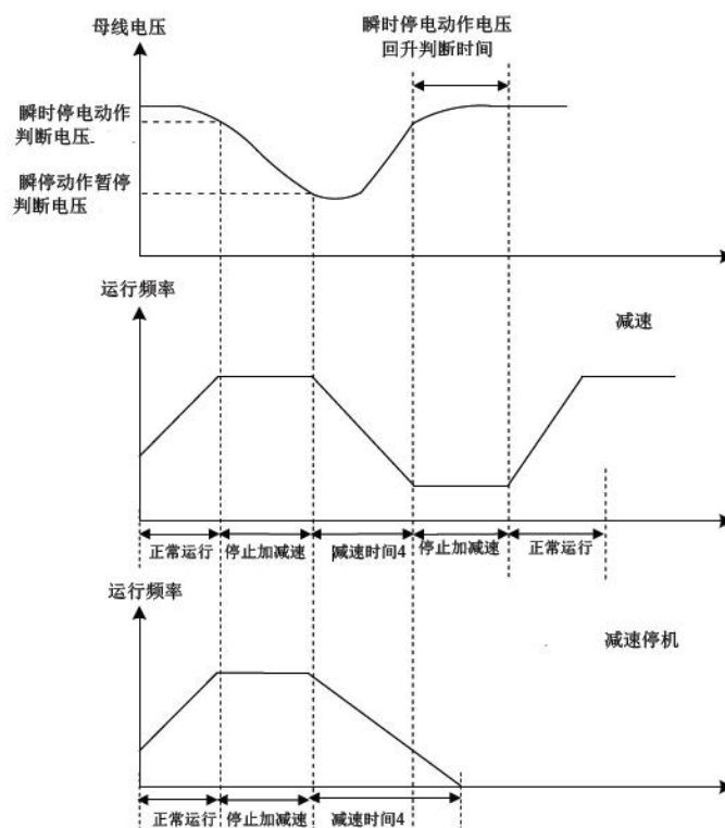
瞬时停电动作示意图
