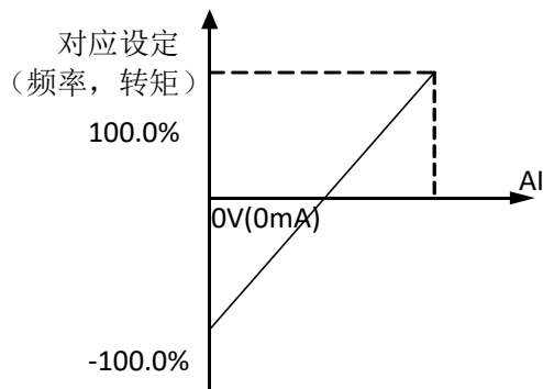
模拟给定与设定量的对应关系
