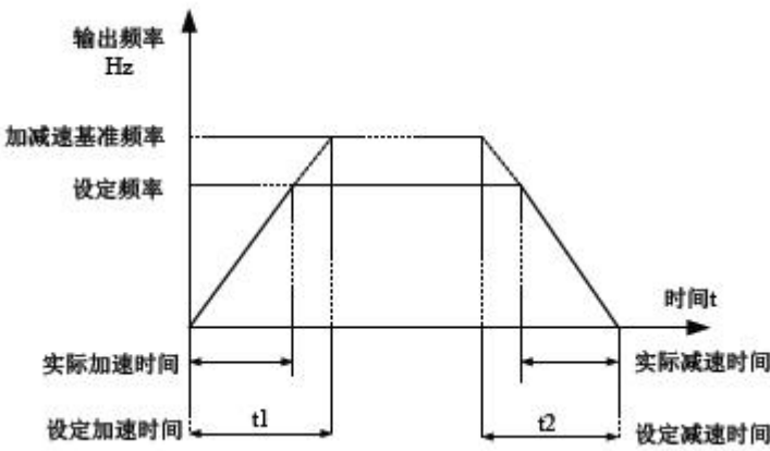
加减速时间示意图
