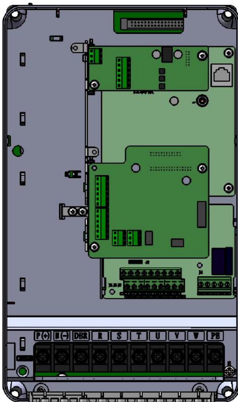
GF630N 控制板安装位置示意图
