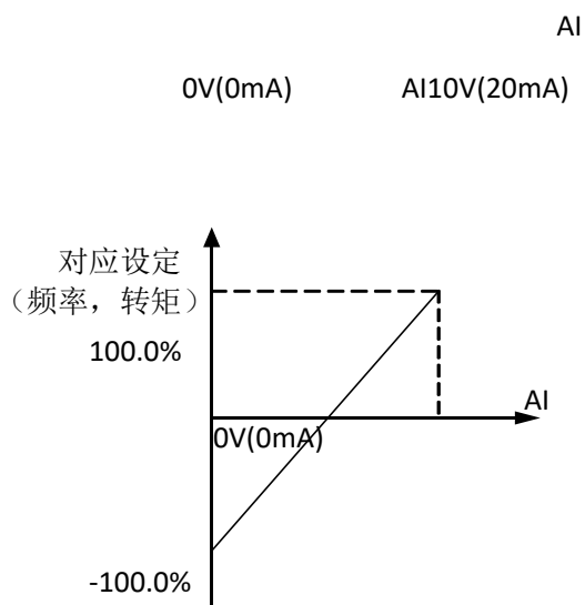
模拟给定与设定量的对应关系
