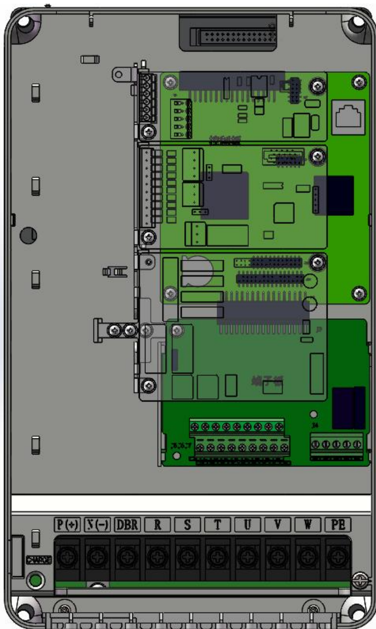
GF630N 控制板安装位置示意图
